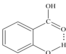
Салициловая кислота
