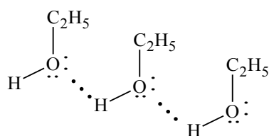
“ пример этилового спирта
