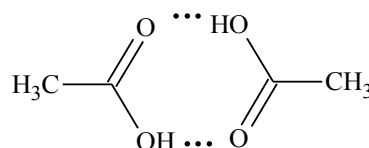
f имер уксусной кислоты
