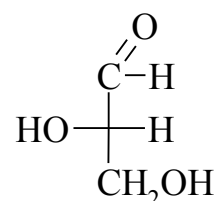
L(-)-глицериновый альдегид
