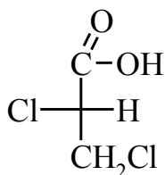
(R)-2,3-дихлорпропионовая кислота
