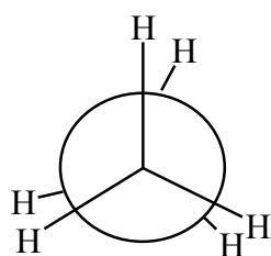
заслоненная конформация этана
