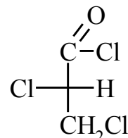
(S)-2,3-дихлорпропионилхлорид
