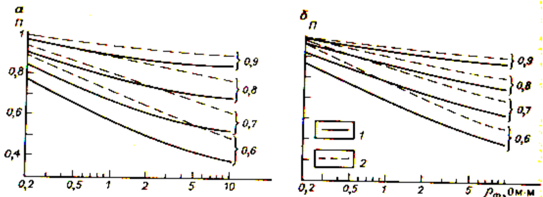
Рисунок 7.5- Зависимости \Pi = f(\rho_v) для различных значений \alpha_{пс} (шифр кривых)
