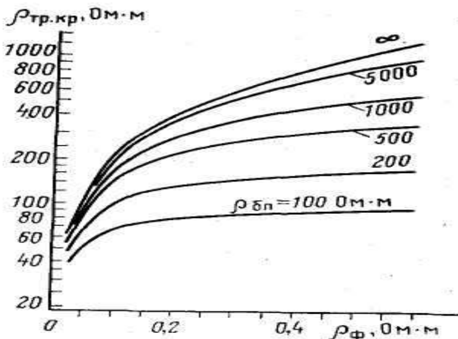
Рисунок 3.2 - Расчётные зависимости критического сопротивления от сопротивления фильтрата промывочной жидкости, насыщающего трещины (по А. Ф. Боярчуку)
