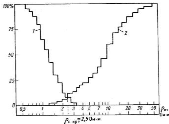
Рисунок 5.4- Определение величины \rho_{пкр} по пересечению статистических распределений \rho_{п} для водоносных (1) и продуктивных (2) коллекторов
