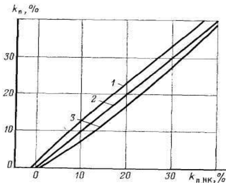
Рисунок 9.3- Сравнение истинной пористости k_n и пористости k_{пнк} > определенной по нейтронному гамма-каротажу для пород различной литологии : 1 — песчаник; 2 — известняк; 3 — доломит
