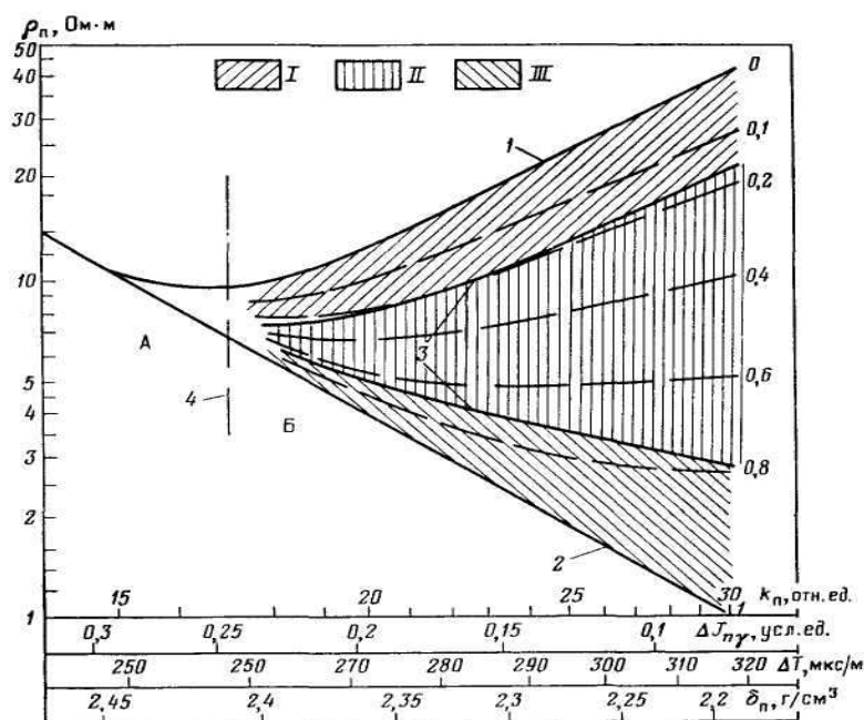
Рисунок 6.4-Палетка для определения характера насыщения коллектора при заданных значениях r_p и k_p .
