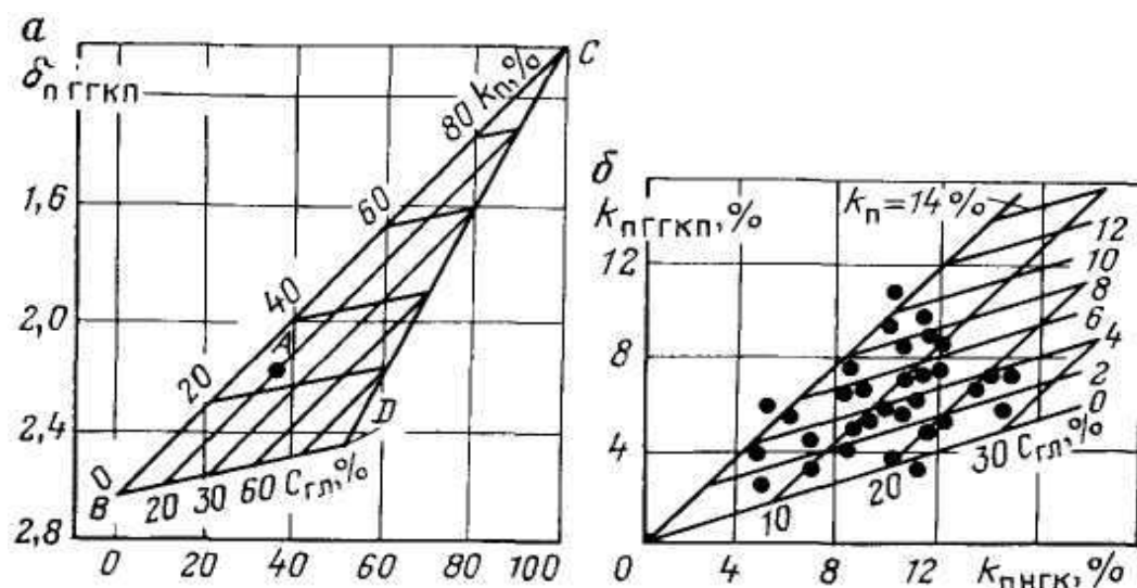
Рисунок 8.3. Треугольная номограмма для определения пористости k_{п} и глинистости C_{г\text{л}} по НГК и ГГК (по данным фирмы Шлюмберже) Зависимости: а - \delta_{п\text{ ГГКП}} = f(k_{п\text{ НГК}}) , б - k_{п\text{ ГГКП}} = f(k_{п\text{ НГК}})
