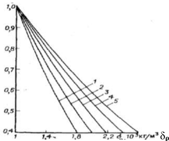
Рисунок 7.3- Зависимость \rho_f от \rho_p и t при \delta_p для тяжёлых растворов . 1 – чистая глина; 2 – то же + 20% барита или 23% гематита; 3 – то же, +40% барита или 46% гематита; 4- то же, + 60% барита или 70% гематита; 5 - то же, + 90% барита
