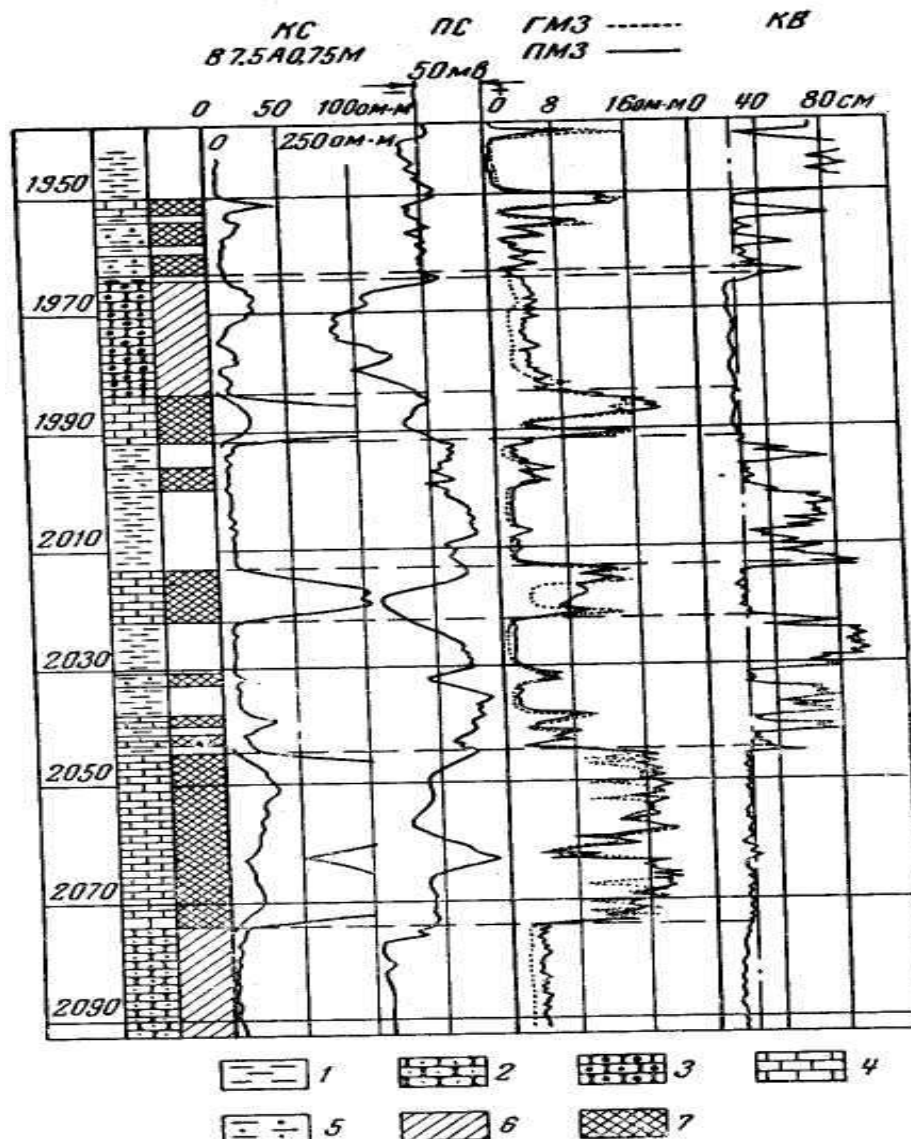
Рисунок 4.2- Расчленение плотных и пористых пород по данным каротажа.
