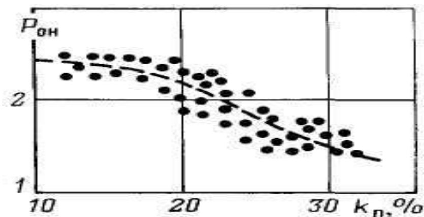
Рисунок 8.2- Сопоставление коэффициента увеличения сопротивления R_{он} промытой зоны с пористостью k_{п} (по В. Д. Шароварину)
