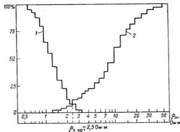
Рисунок 6.1- Определение величины \rho_{пкр} по пересечению статистических распределений \rho_{п} для водоносных (1) и продуктивных (2) коллекторов
