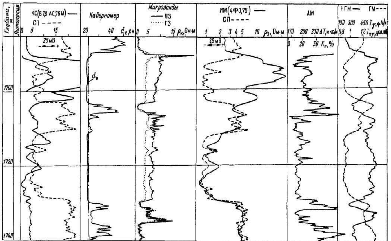
Рисунок 4.3 - Расчленение терригенного разреза и выделение коллекторов по стандартному комплексу ГИС.
