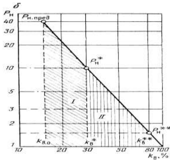
Рисунок 7.6- Зависимости k_{пр.н} = f(k_B) , k_{пр.в} = f(k_B) (а) и p_H = f(k_B) (б). / — нефть; // — нефть + вода; /// — вода
