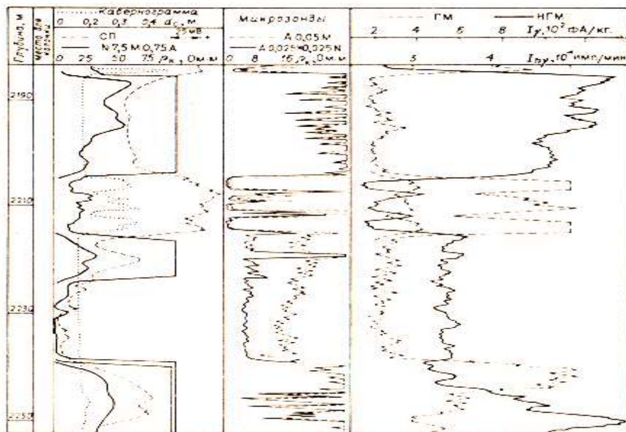
Рисунок 7.3- Комплекс диаграмм методов ГИС по участку терригенно-карбонатного разреза : d_c=0,25\text{м} , \rho_p=1,2 \text{ Ом}
