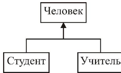
Рисунок 6.1 – Иерархия классов.
