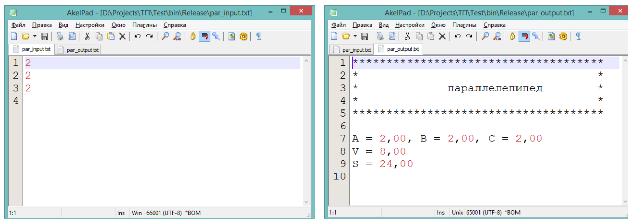
Рисунок 6.7 – Файлы release-приложения
