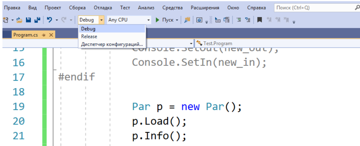
Рисунок 6.5 – Настройки конфигурации
