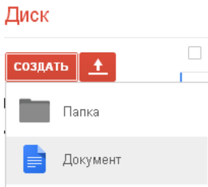
Рисунок 9.10 – Создание документа
