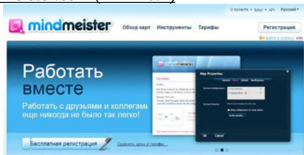
Рисунок 10.7 – Сервис mindmeister
