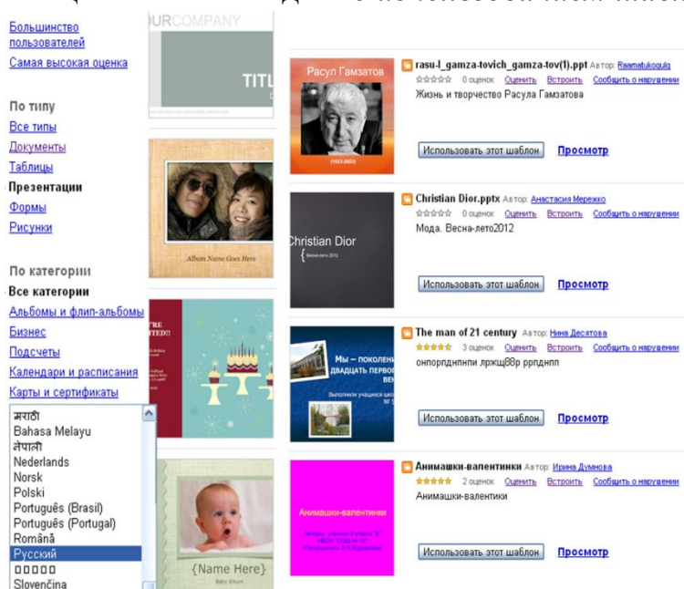
Рисунок 9.16 – Использование шаблонов
