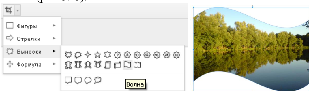
Рисунок 9.19 – Операция кадрирования
