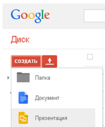
Рисунок 9.14 – Создание презентации
