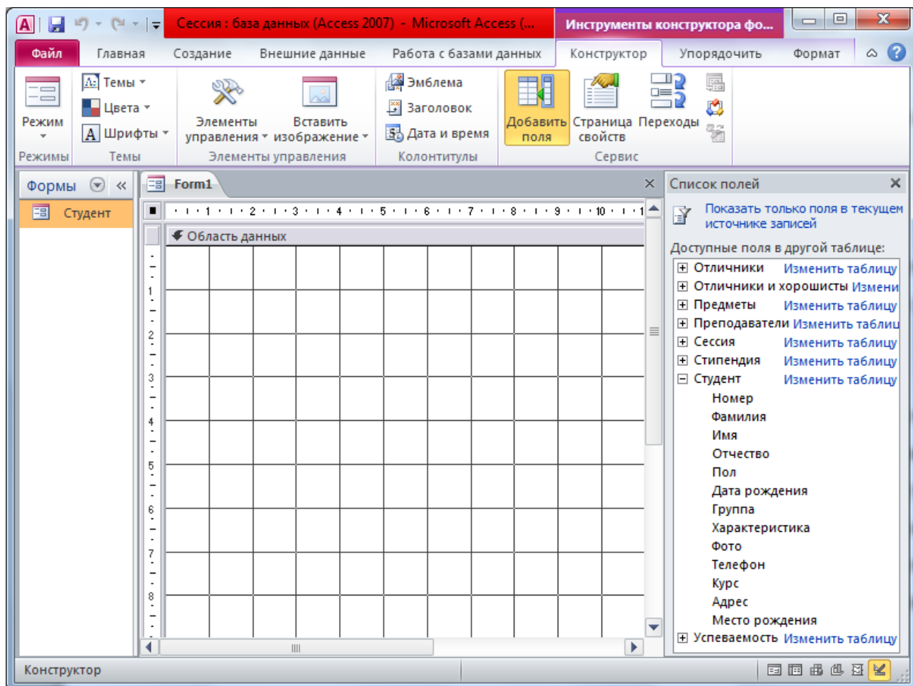
Рисунок 4.17. - Конструктор форм
