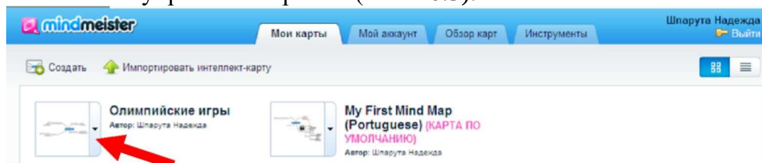
Рисунок 10.9 – Окно программы
