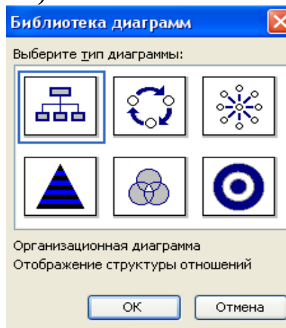
Рисунок 5.12. – Библиотека диаграмм
