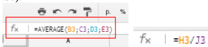
Рисунок 9.30 – Ввод формул
