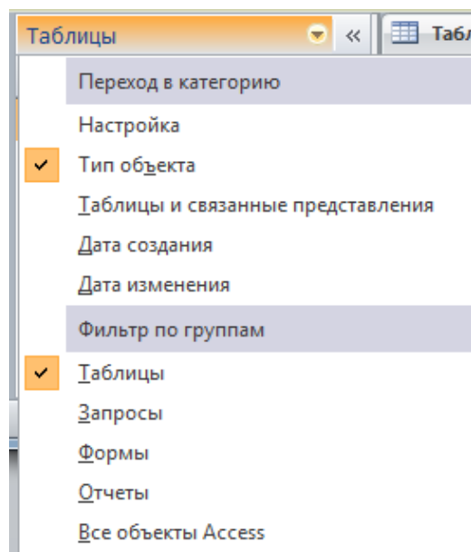
Рисунок 4.3. - Панель объектов
