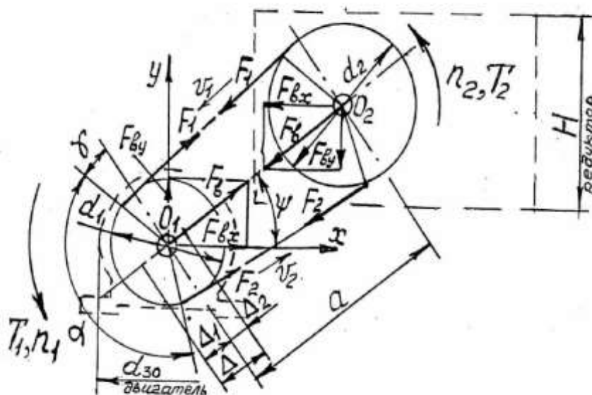
Рис.1.1. Расчетная схема ременной передачи
