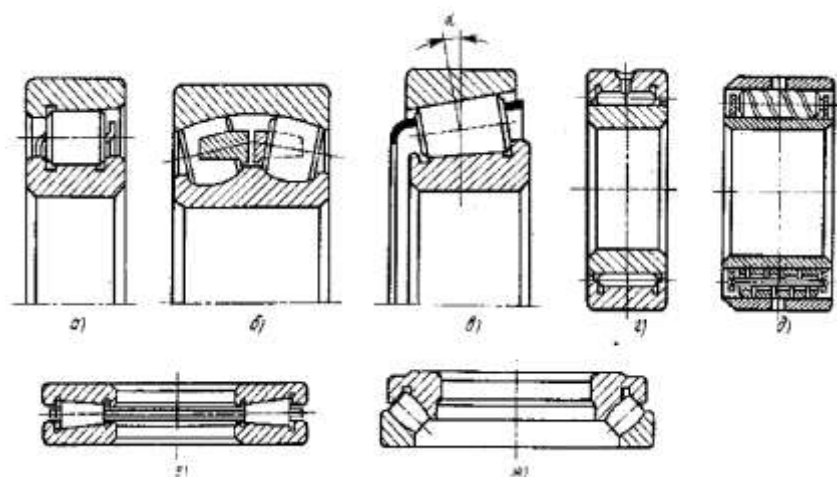
Рис. 1.3. Основные типы роликоподшипников: а – радиальные с короткими (или с длинными) цилиндрическими роликами; б – радиальные с бочкообразными роликами двухрядные
