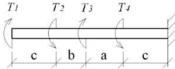
Схема вала
