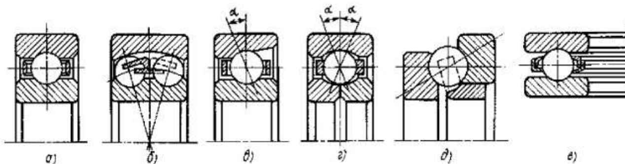
Рис. 1.2. Основные типы шарикоподшипников: а – радиальные однорядные; б – двухрядные; в, г – радиально-упорные; д – упорно-радиальные; е – упорные
