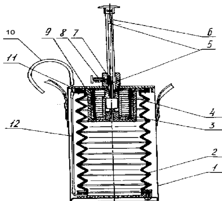
Рис. 12. Газоанализатор УГ-2
