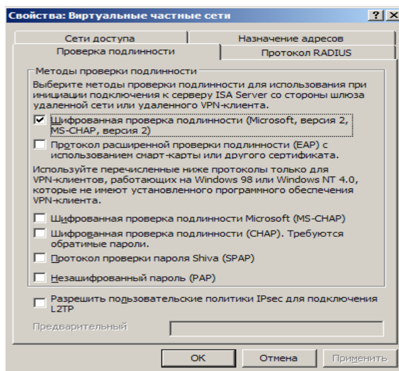
Рис.16. Вкладка «Проверка подлинности (Authentication)»
