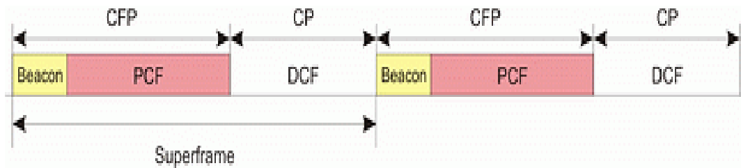
Рис. 8. Объединение режимов PCF и DCF в одном суперфрейме
