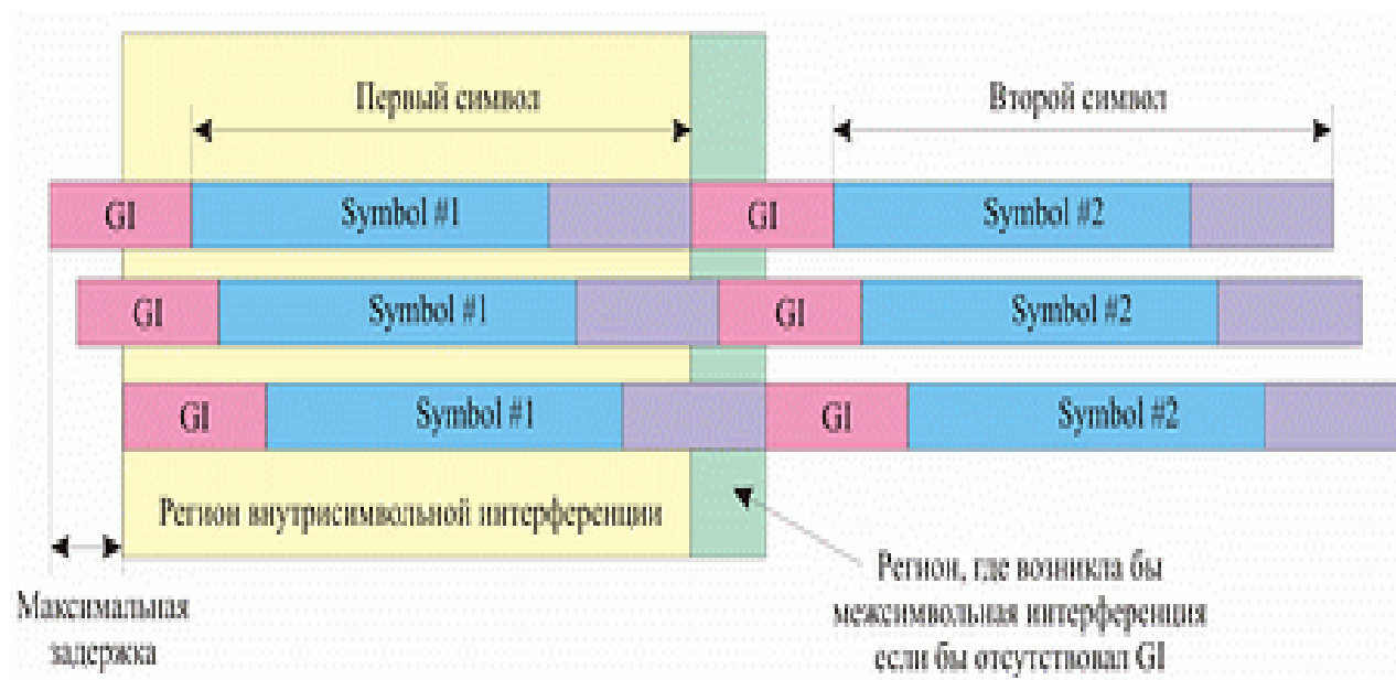
Рис. 19. Избежание междисимвольной интерференции за счет использования охранных интервалов
