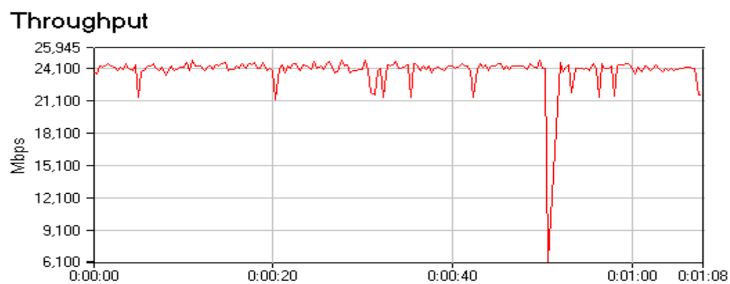
Рис. 59. Размер пакета 512 байт.
