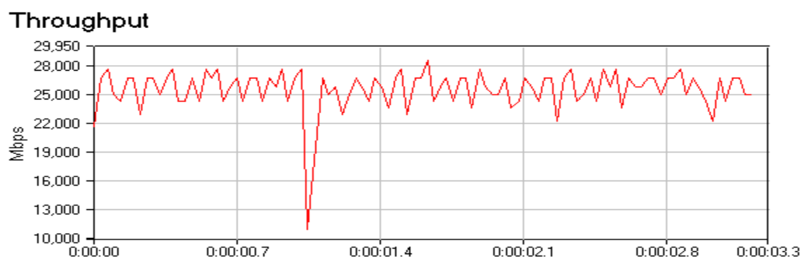
Рис. 60. Размер пакета 64 байта.
