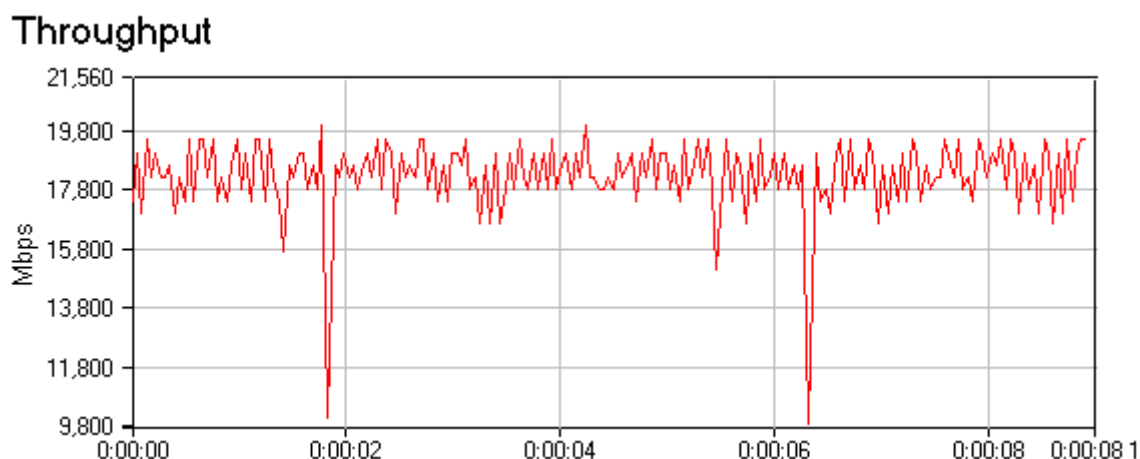
Рис. 69. длина поля данных 2000 бит
