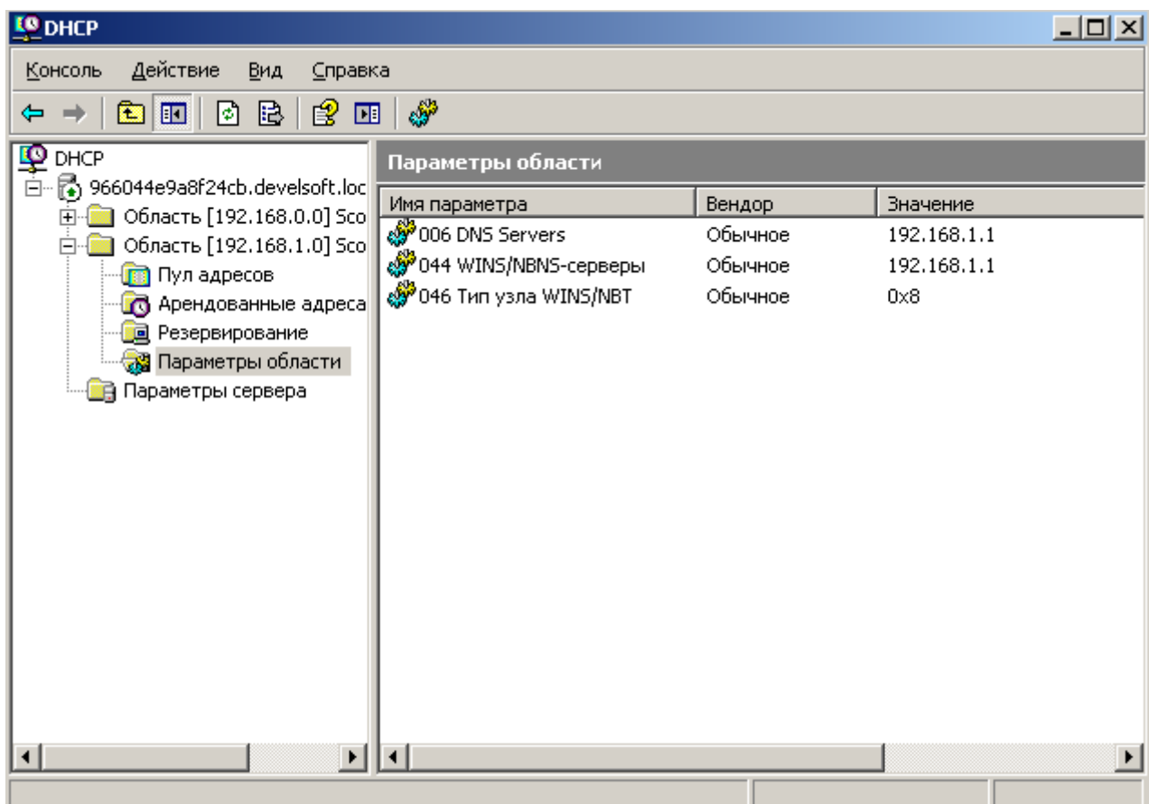
Рис. 14. Параметры области, по консоли DHCP
