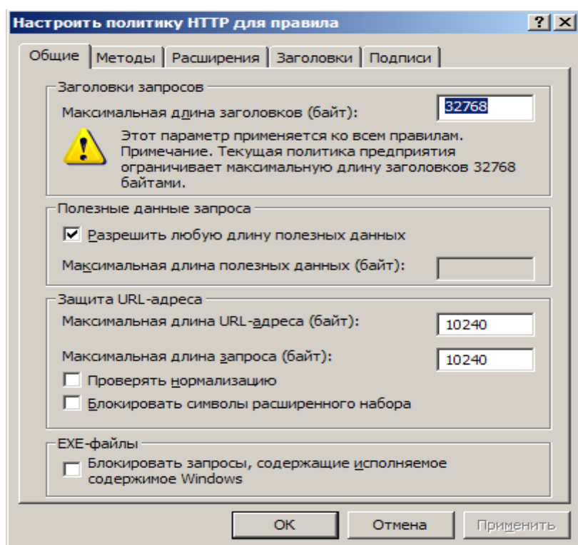
Рис. 1. Вкладка «Общие (General)»
