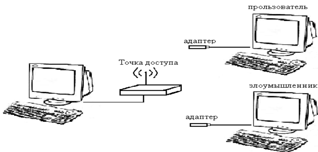
Рис. 79. Тестовый стенд для проверки методов шифрования
