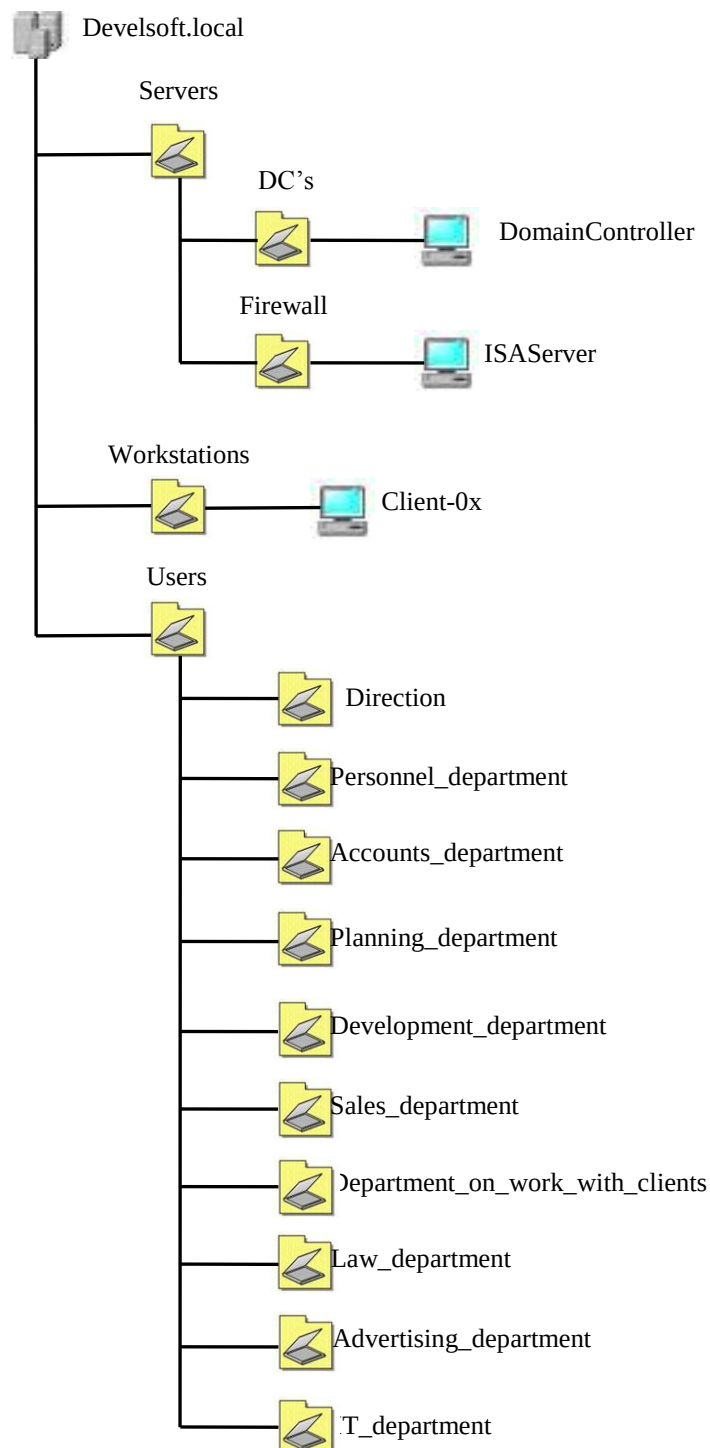
Рис. 3. Схема Active Directory
