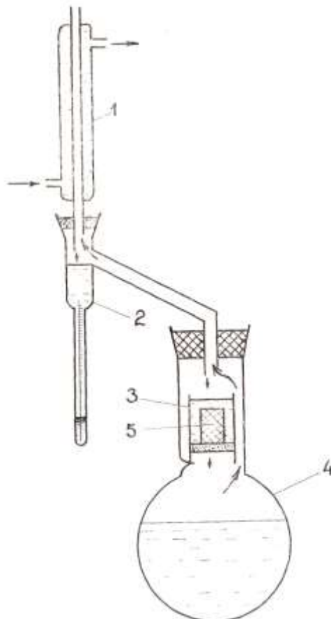
Рис. 7.1. Прибор Закса
