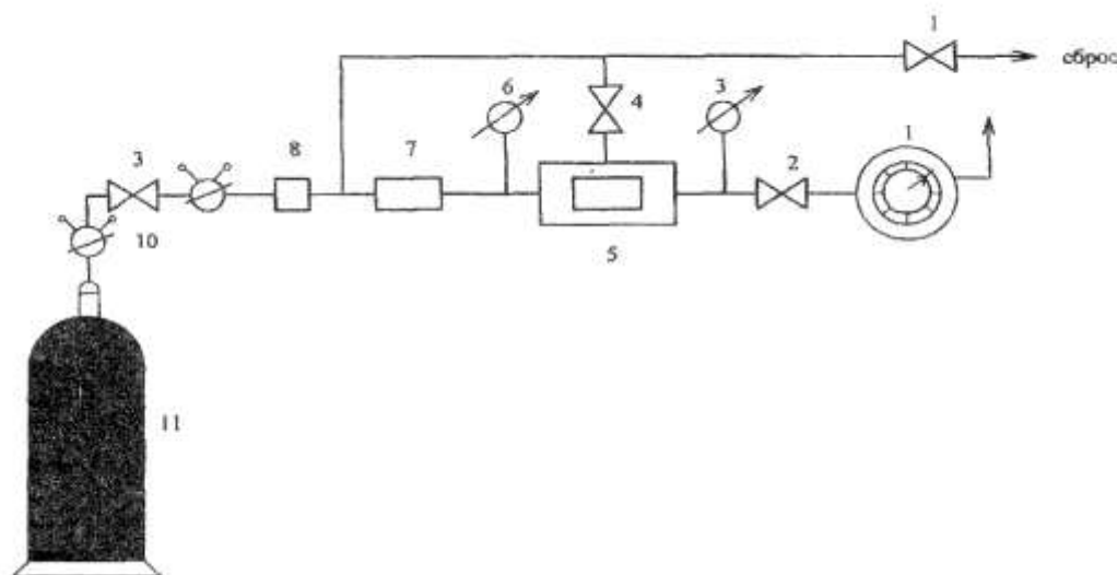
Рис. 4.1. Схема установки для определения газопроницаемости 1 – газочасовой счетчик; 2 – кран сброса газа; 3 – манометр перед образцом; 4 – кран обжима керна; 5 – кернодержатель; 6 – манометр перед образцом; 7 – хлоркальциевая трубка; 8 – фильтр; 9 – кран подачи газа; 10 – редуктор давления; 11 – источник давления.
