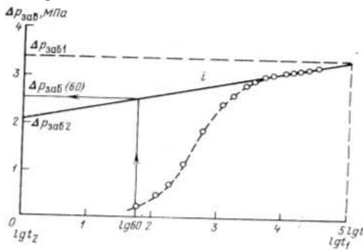
Рисунок 2 – Кривая восстановления давления в координатах \Delta P и \lg t
