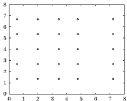
Конфигурация статистической системы в момент времени t = 0,05
