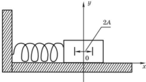
К построению модели линейного гармонического осциллятора
