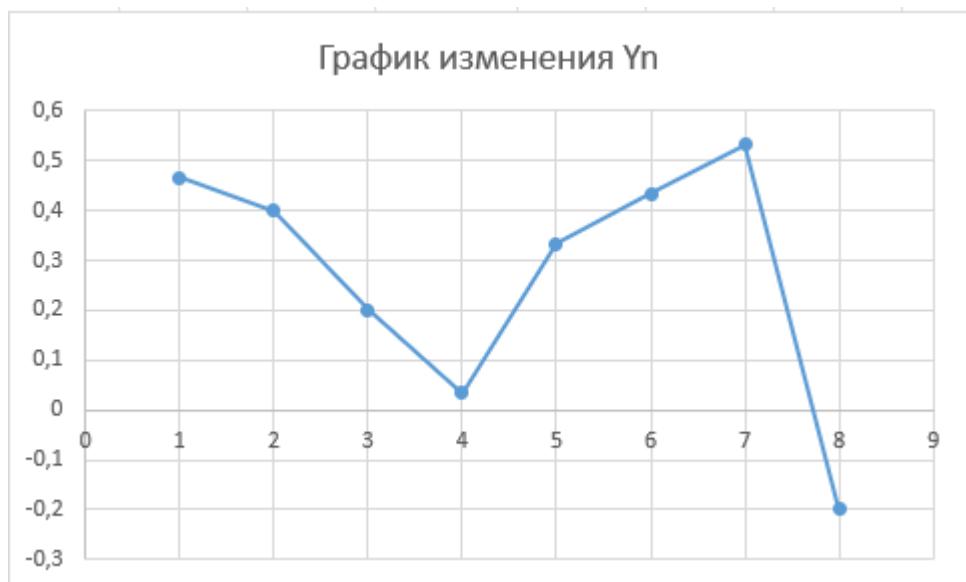
Рисунок 8. График изменения Y_n
