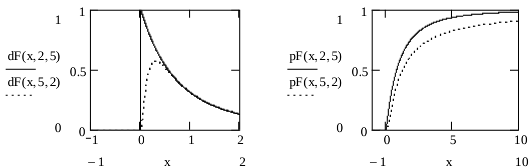
Рисунок 6. Графики плотности вероятностей и функций распределения в случае F-распределения для p=2,5 и m=5,2
