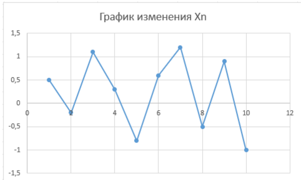
Рисунок 7. График изменения X_n
