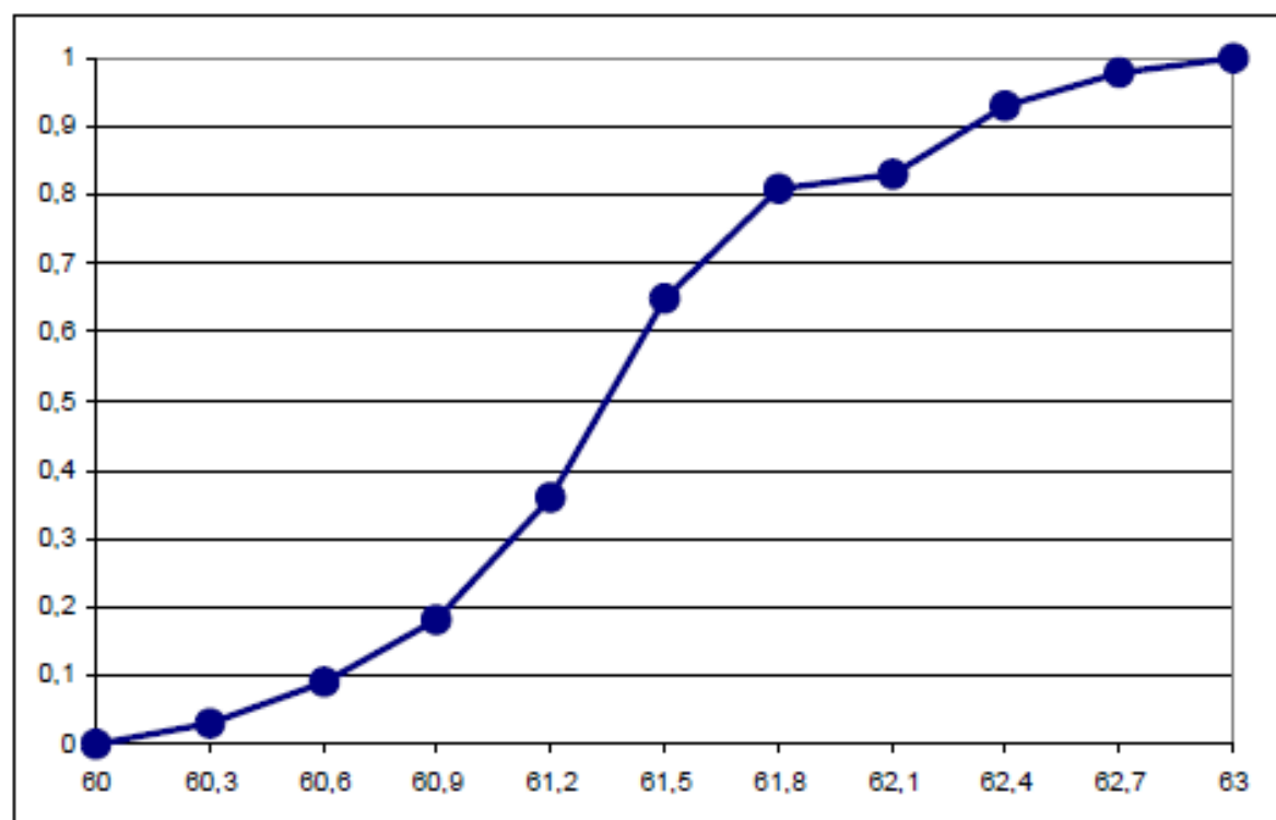
Рис. 3. Кумулятивная кривая.
