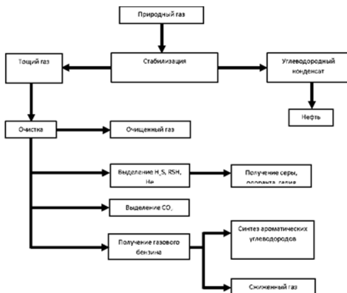
Рисунок - Структурная схема переработки природного газа
