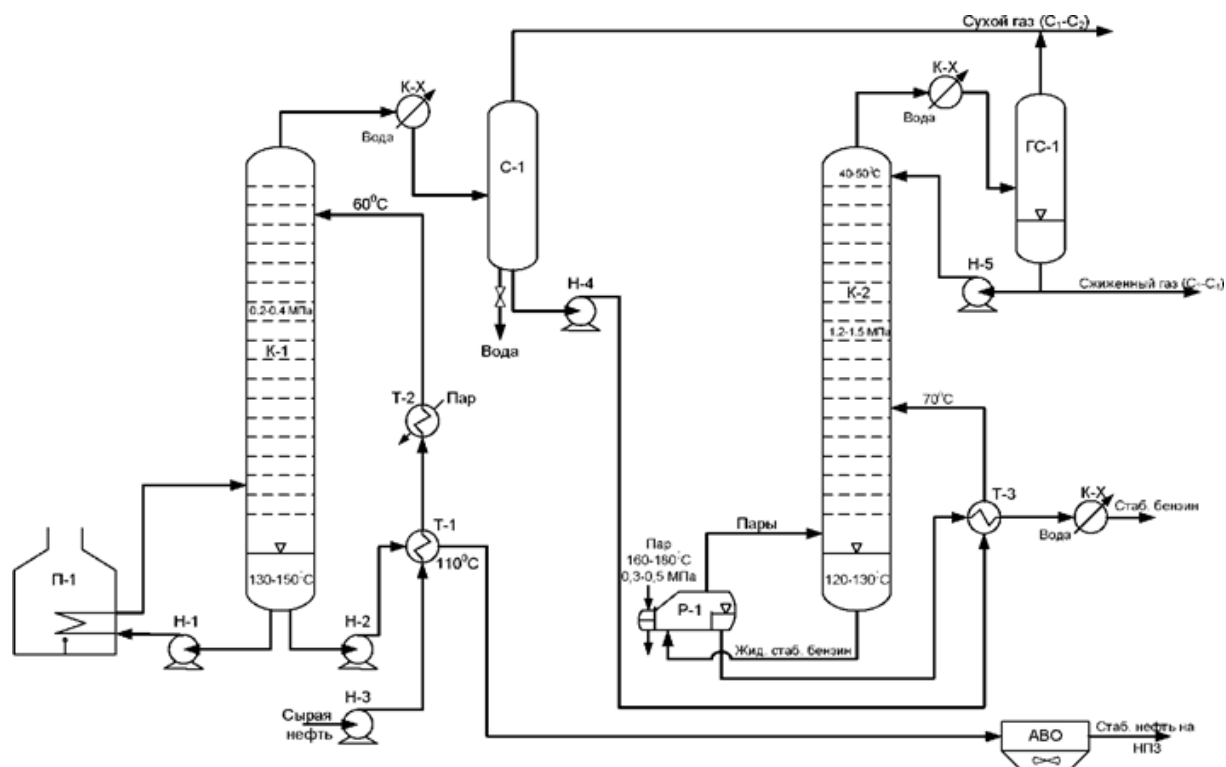
Рисунок - Технологическая схема установки стабилизации нефти
