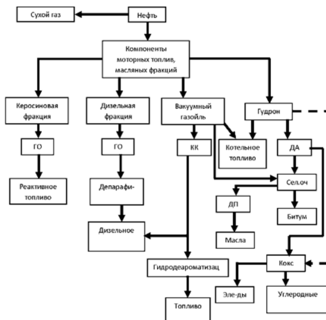
Рисунок - Структурная схема переработки нефти
