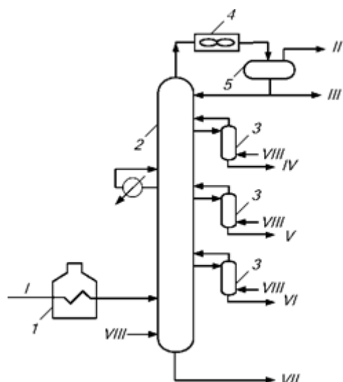
Рисунок - Перегонки нефти по схеме однократного испарения в сложной колонне с отпарными секциями:
