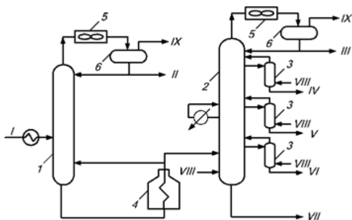
Рисунок - Перегонка нефти по схеме двукратного испарения с частичным отбензиниванием нефти: 1 - колонна под давлением; 2 - атмосферная колонна; 3 - отпарная секция; 4 - трубчатая печь; 5 - конденсатор воздушного охлаждения; 6 - сепаратор-отстойник
