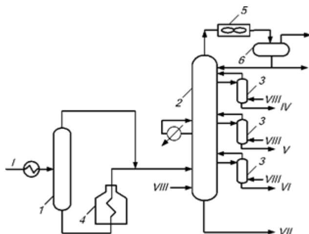
Рисунок - Перегонка нефти по схеме с предварительным однократным испарением: 1 -
