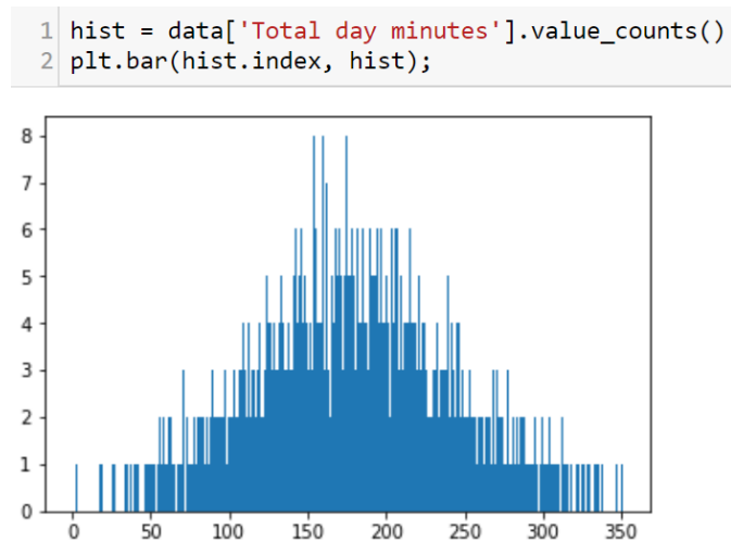
Рисунок 2.6 – Использование matplotlib для представления распределения значений признака
