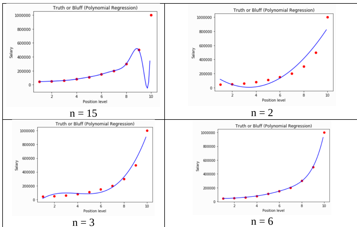
Рисунок 10.2 – Анализ модели полиномиальной регрессии
