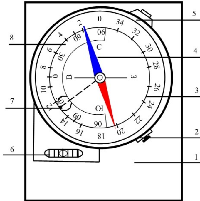
Рисунок 8 – Горный компас (1 – металлическая пластинка, 2 – стопорный винт, 3 – лимб, 4 – магнитная стрелка, 5 – стопор отвеса, 6 – уровень, 7 – отвес, 8 – клинометр)
