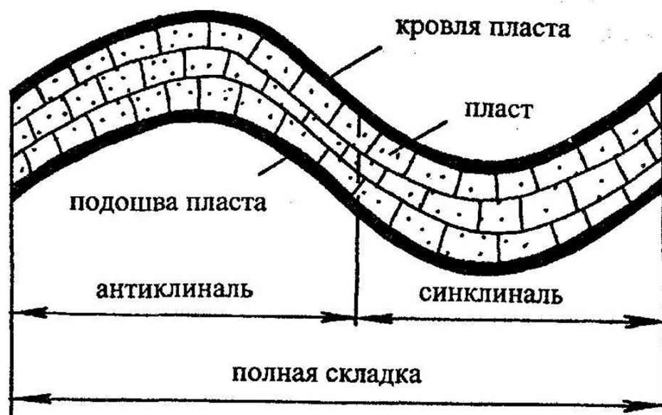
Рисунок 7 – Элементы пласта и складки
