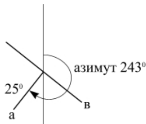
Рисунок 9 – Элементы залегания пород (а – линия падения, в – линия простирания)
