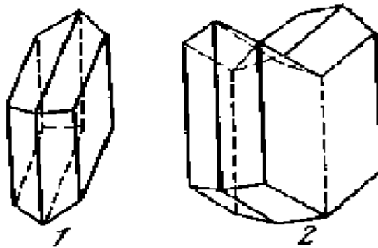
Рисунок 1. Единичный кристалл гипса (1) и двойник сростания «ласточкин хвост» (2)
