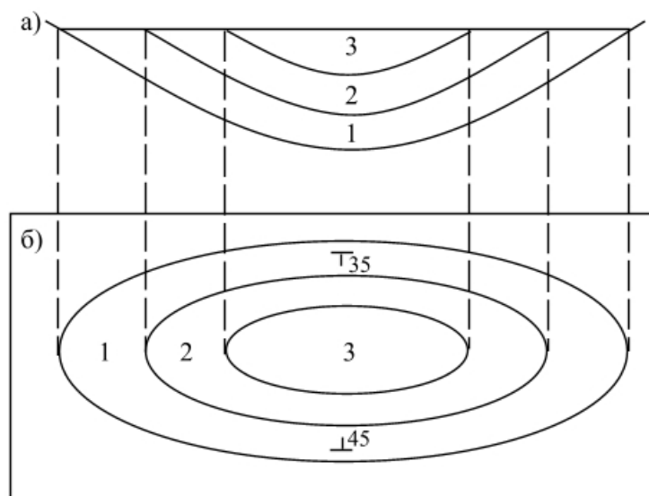
Рисунок 15 – Изображение синклиналей (а – разрез, б – карта)
