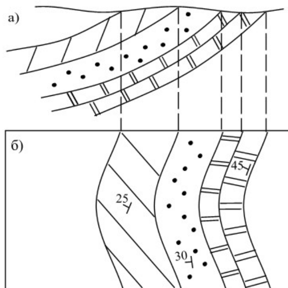
Рисунок 13 – Наклонное залегание пород (а – разрез, б – карта)
