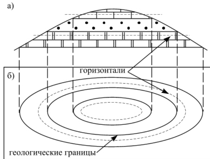
Рисунок 12 – Горизонтальное залегание пород (а – разрез, б – карта)
