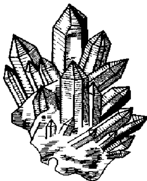
Рисунок 2. Друза кварца
