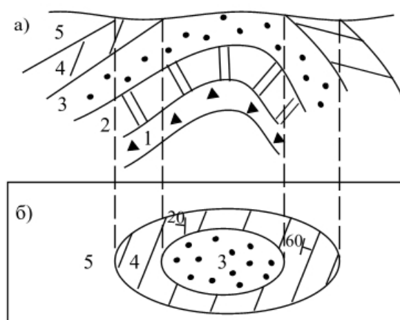
Рисунок 14 – Складчатое залегание пород (а – разрез, б – карта)
