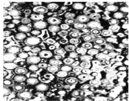
Рисунок 4. Оолиты арагонита
