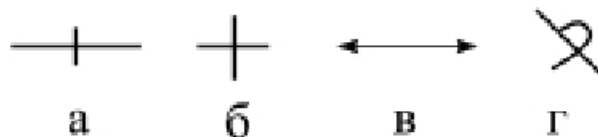
Рисунок 10 – Положение слоев (а, б – горизонтальное, в – вертикальное, г – перевернутое)
