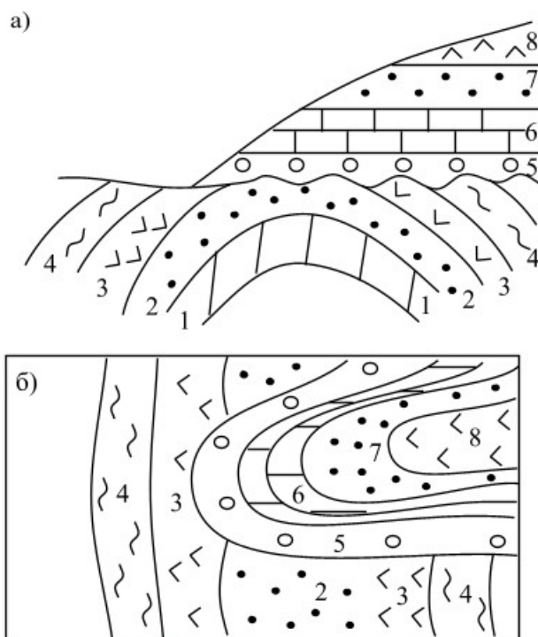
Рисунок 17 – Стратиграфические несогласия (а- разрез, б – карта)
