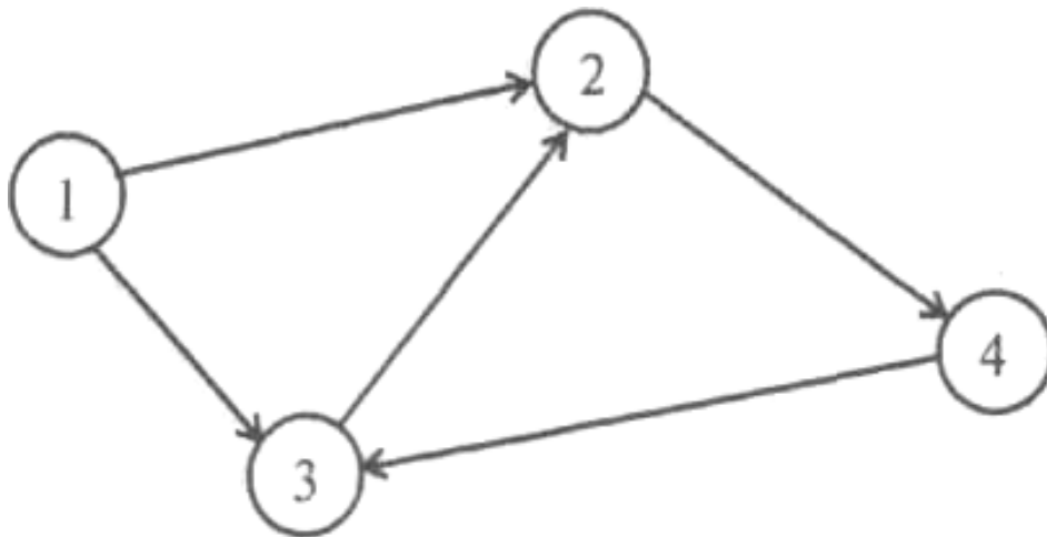
Рисунок .1 – Пример оргграфа с контуром
