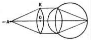
Рис. 7. Схема, поясняющая расчет силы аккомодации.
