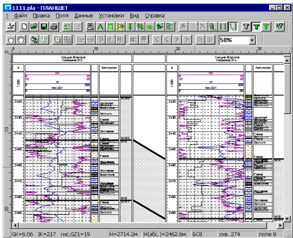
Рисунок 7.5 Пример построения профиля
