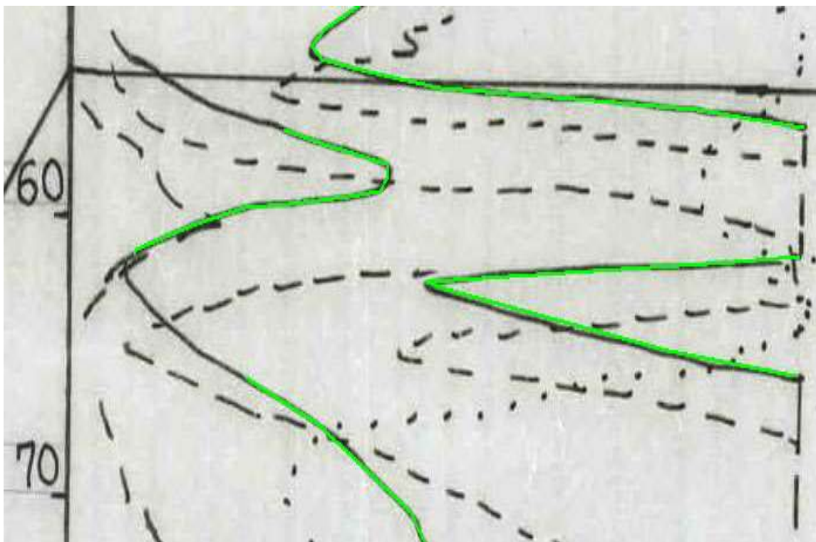
Рисунок 1.1 Оцифровка каротажной кривой, разбитой на несколько шкал (бликов)
