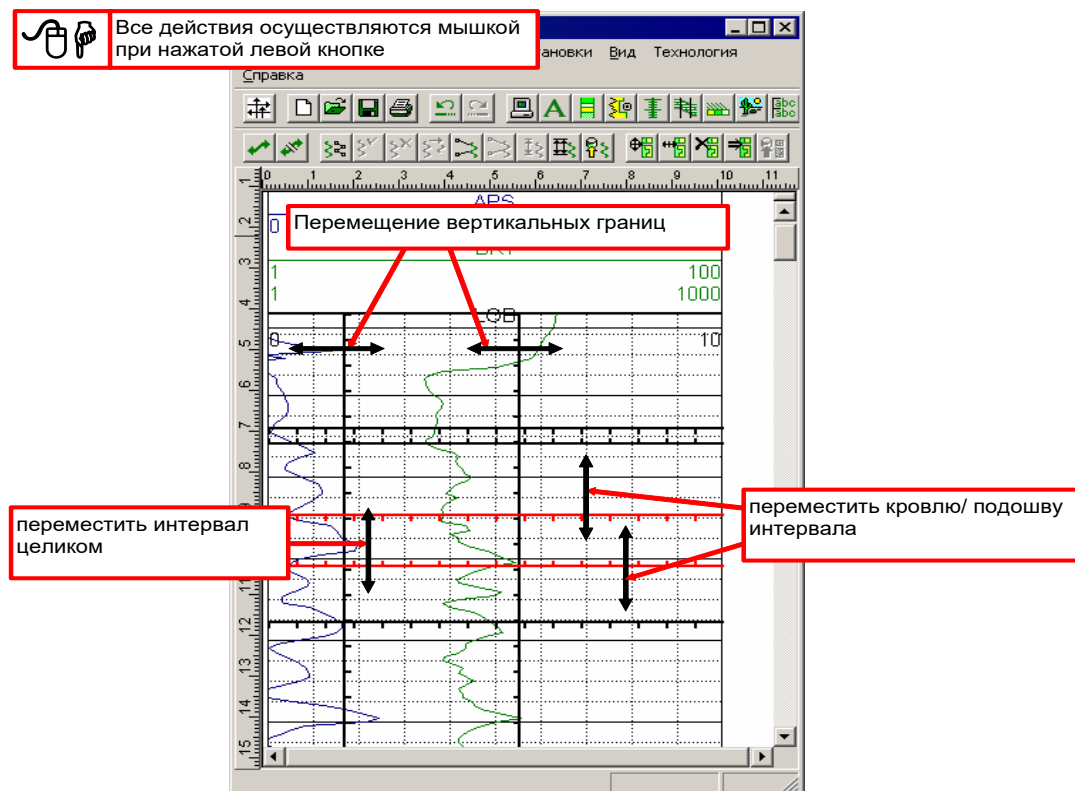
Рисунок 9.1 Пример нормировки геофизических кривых.
