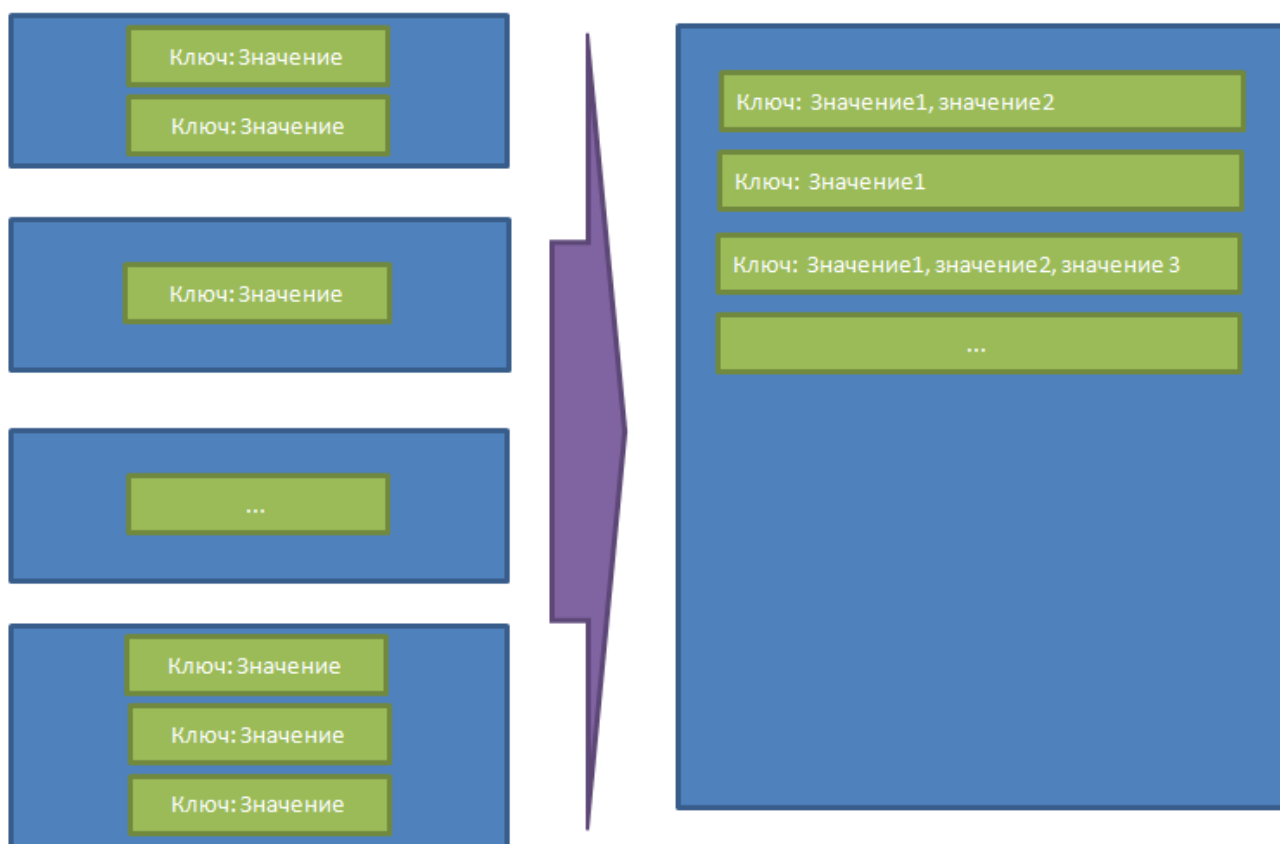
Рисунок 2 – Графическое изображение группировки данных по ключу
