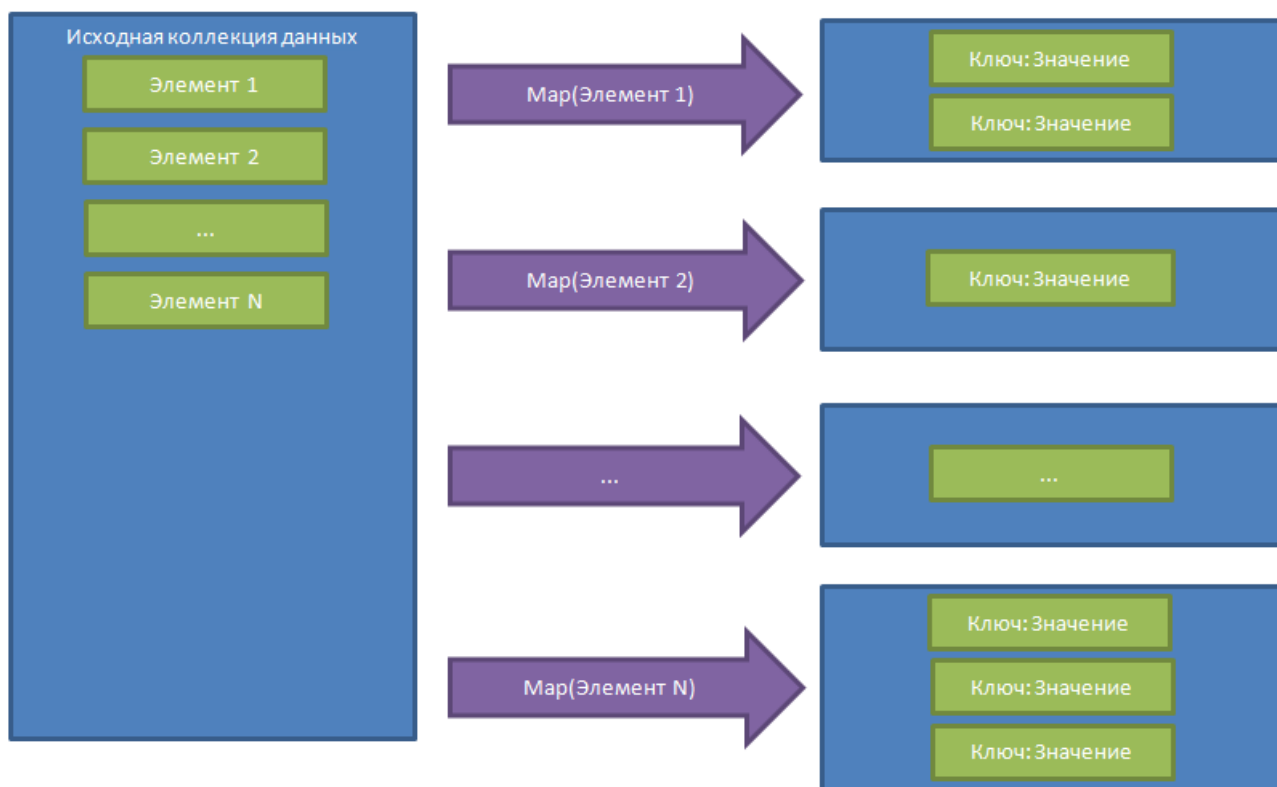
Рисунок 1 – Графическое изображение работы Мар-шага
