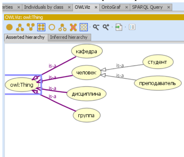
а) OWLViz
