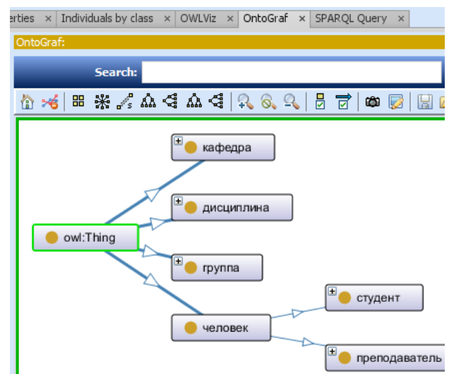
б) OntoGraf
