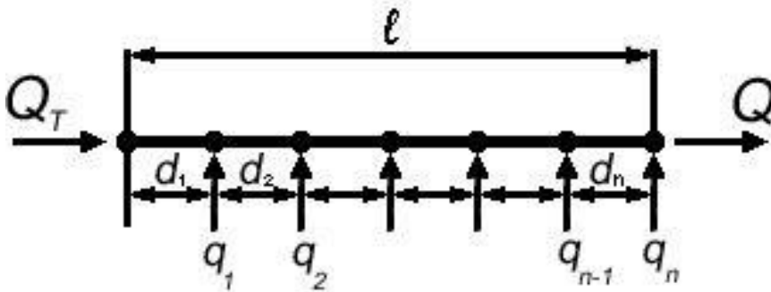
Рисунок 6.5 – Расчетная схема сложного трубопровода II категории
