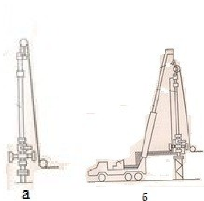
а - стационарный лубрикатор, б - лубрикатор установленный на передвижной вышке
