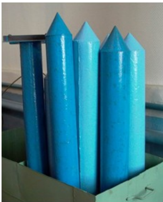
Рисунок 11.7– Калибровка каналов аппаратуры нейтронного каротажа
