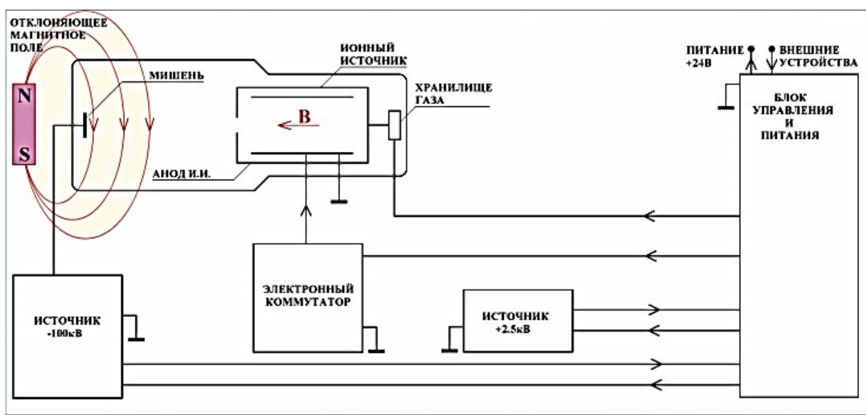
Рисунок 5.4 - Блок – схема включения ускорительной нейтронной трубки
