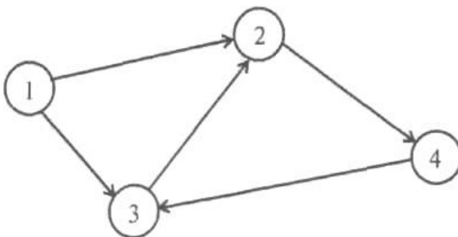
Рисунок 4.1 – Пример орграфа с контуром
