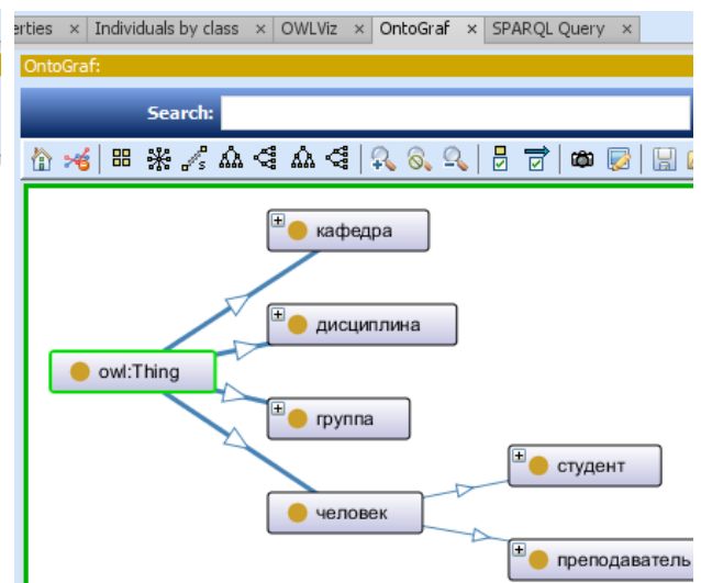
б) OntoGraf
