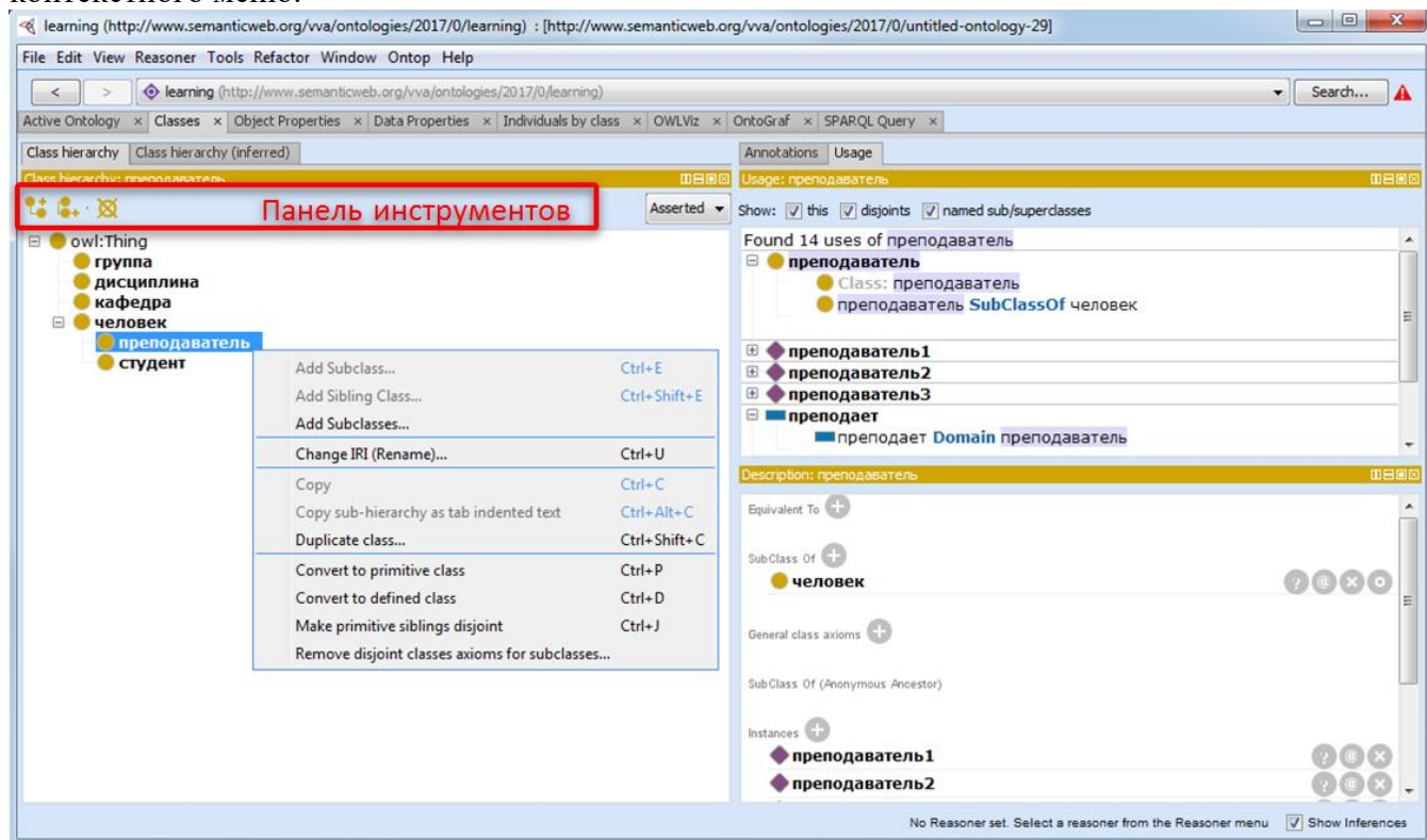
Рис.3. Вкладка «Classes»
