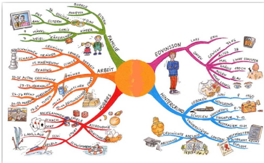
Рисунок 10.6 – Примеры интеллект-карт
