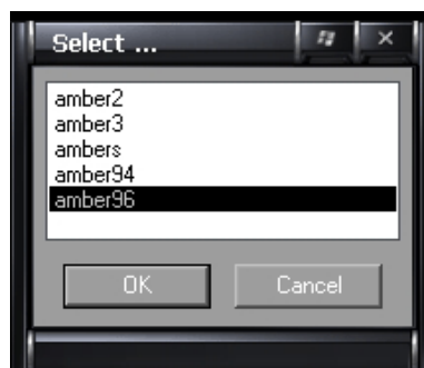
Рисунок 2 – Вид формы для выбора версии силового поля AMBER в
