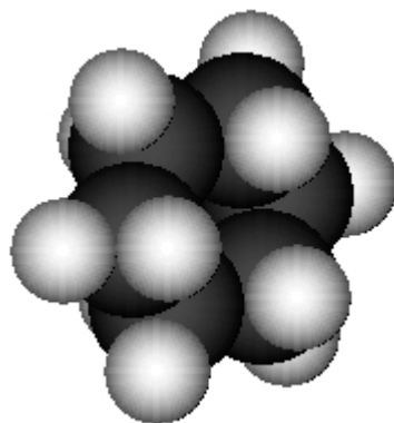
Рисунок 5 - Варианты представления трёхмерной модели циклогексана в HyperChem: а) Balls (Шары); б) Sticks&Dots (Стержни и точки).
