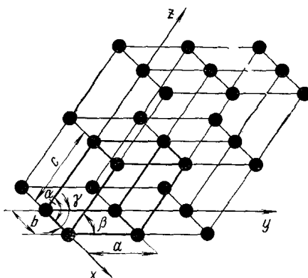
Рисунок 1 – Фрагмент кристаллической решетки и параметры элементарной ячейки.
