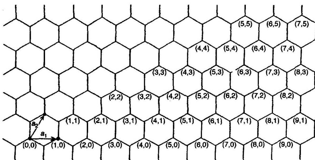
Рисунок 3 – Графитовый слой с атомами углерода, обозначенными в прямоугольной системе координат с осями \vec{a}_1 и \vec{a}_2 .
