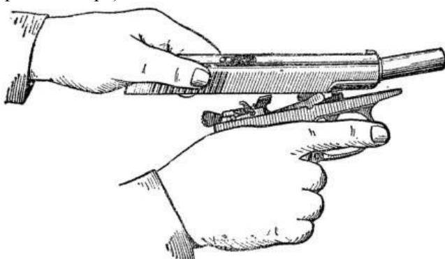
Рис. 7. Присоединение затвора к рамке
