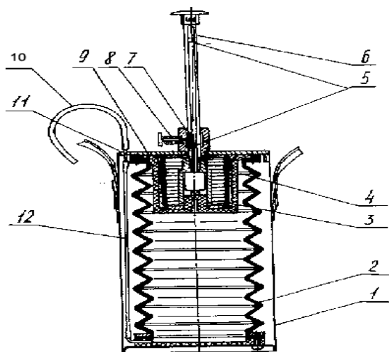
Рис. 12. Газоанализатор УГ-2
