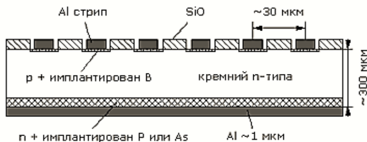
Рисунок 2.5 – Устройство кремниевого микрострипового детектора
