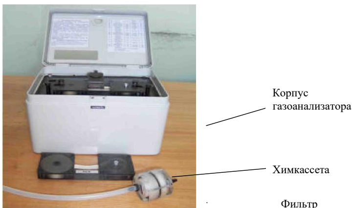
Рисунок 3.2 – Общий вид газоанализатора ГАНК-4
