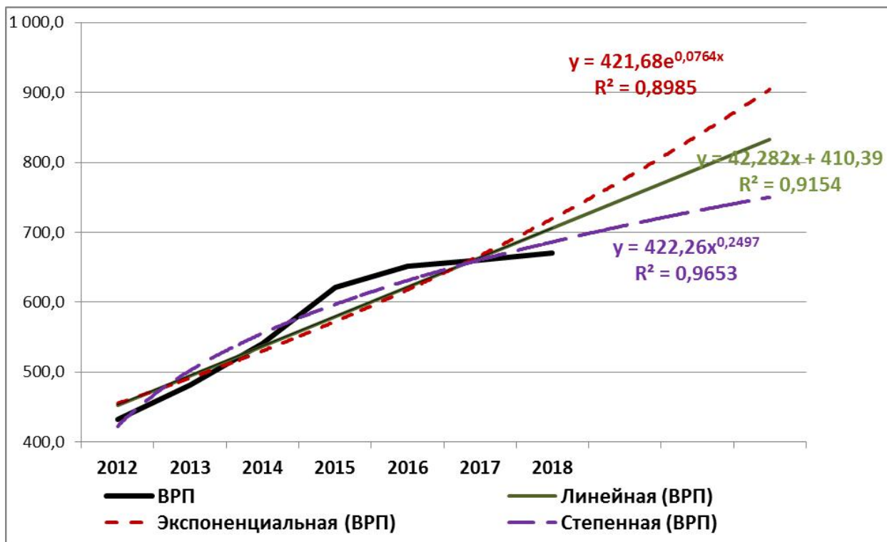
Рисунок 4.1 – Прогноз ВРП Ставропольского края в текущих ценах, млрд. руб.
