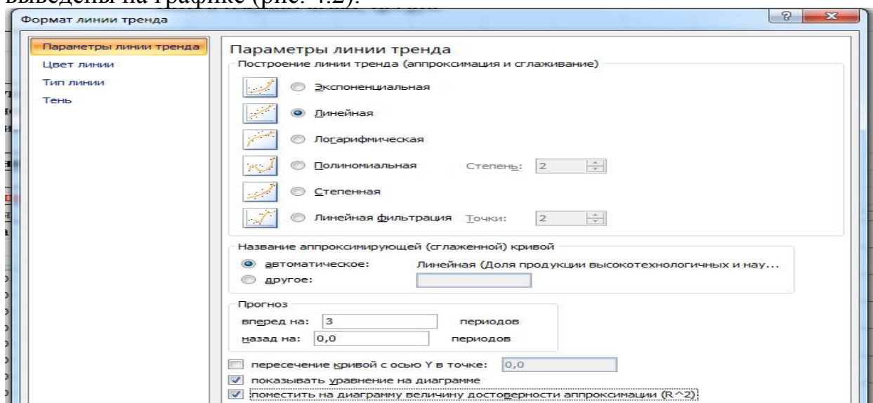
Рисунок 4.2 – Пример определения уравнения тренда
