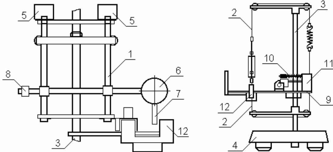
Рис. 1. Схематическое изображение экспериментальной установки.
