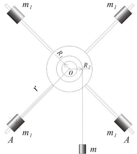
Рис. 23. Маятник Обербека
