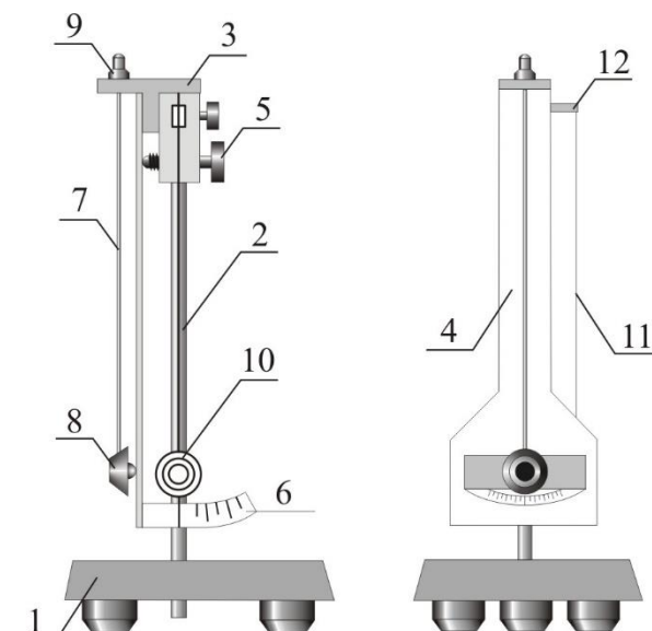
Рис. 3. Схематическое изображение экспериментальной установки
