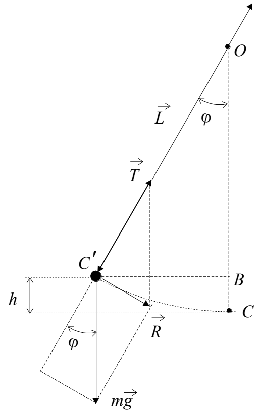
Рис. 1. Математический маятник
