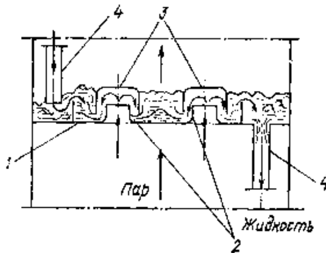
Рисунок 8.1 – Схема работы колпачковой тарелки:
