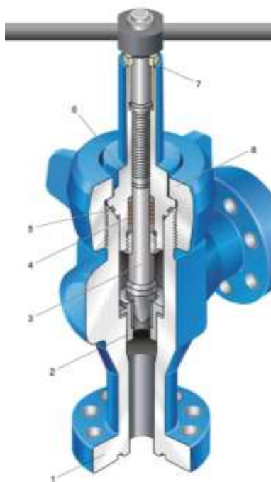
Рисунок 1.10 – Дроссель: 1– корпус; 2 – седло; 3 – игла; 4 – пакет уплотнений; 5 – кольцо уплотнительное; 6 – корпус иглы; 7 – указатель
