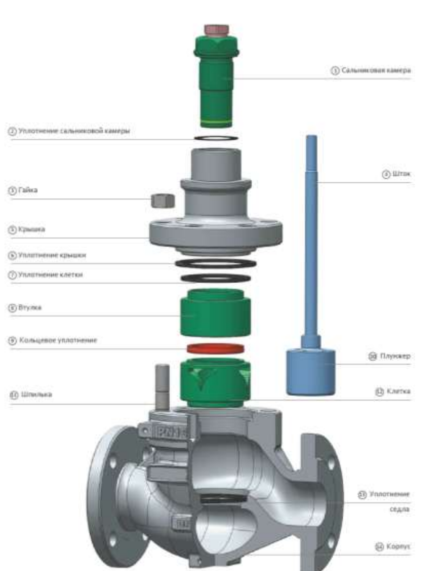
Рисунок 2.1 – Клапан регулирующий
