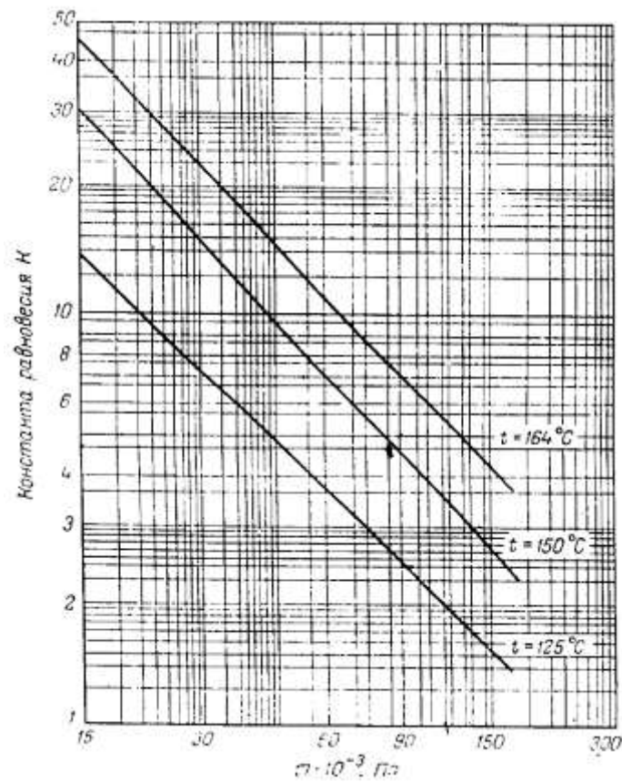
Рисунок 8.4 – Зависимость константы равновесия воды в системе ДЭГ - вода от температуры и давления
