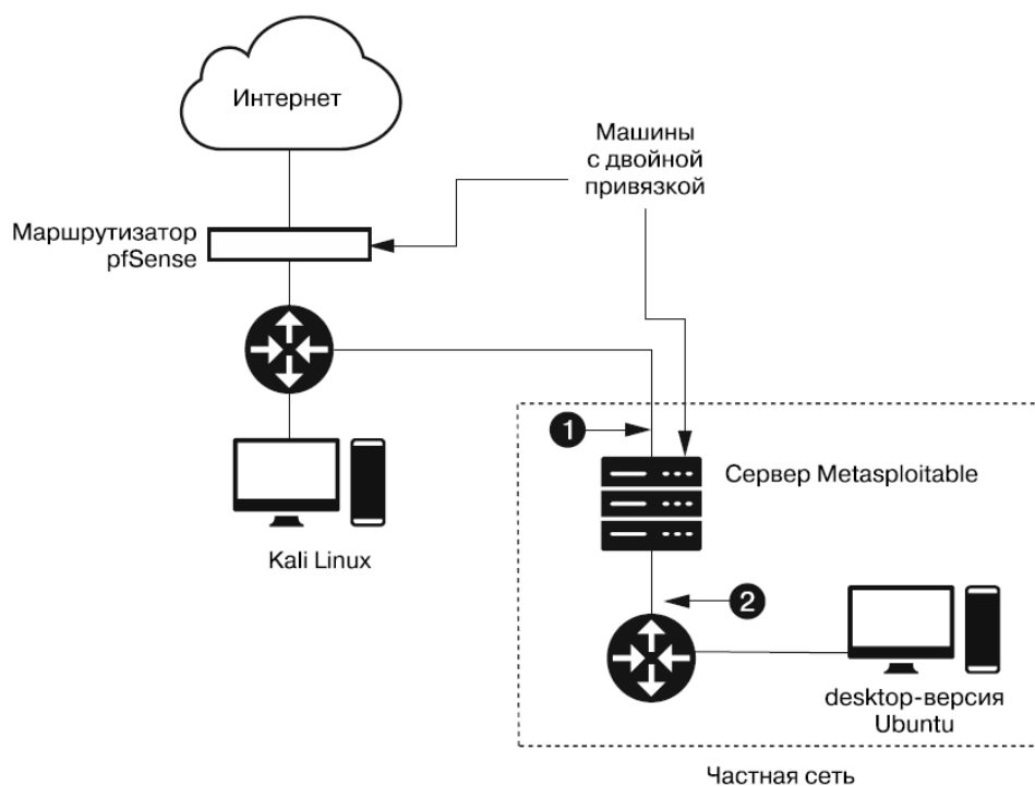
Рис. 14.1. Схема сети
