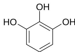
пирогаллол
