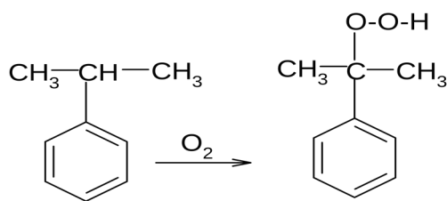
кумол
