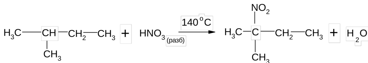
2-метил-2-нитробутан
