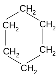
моноклический алкан
