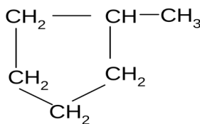
метилциклопентан
