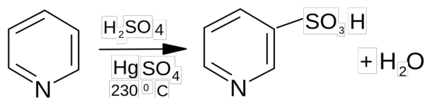
3-сульфопиридин
