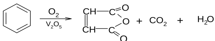
малеиновый ангидрид
