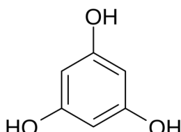
флороглюцин
