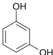
резорцин
