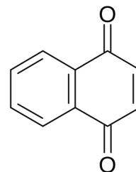
α-нафтахинон
