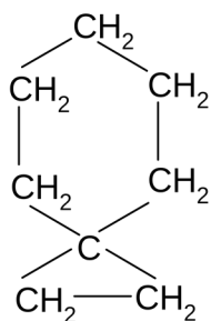
спиранный углеводород
