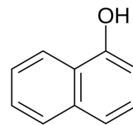
альфа-нафтол
