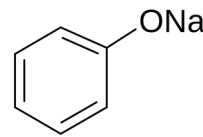
фенолят натрия
