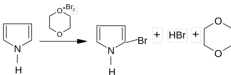
\alpha -бромпиррол
