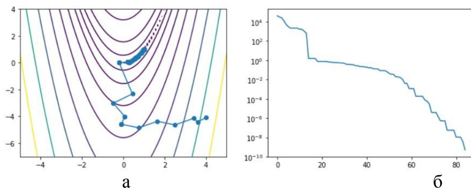
Рисунок 6.6 – Поиск минимума функции Розенброка симплекс-методом Нелдера-Мида: последовательность приближенных решений на различных итерациях
