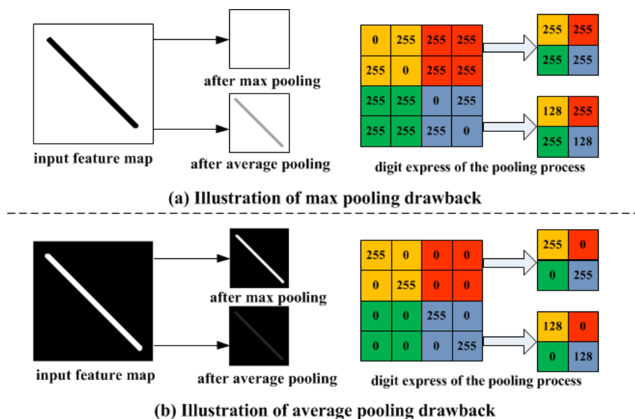
Рисунок 7.3 – Иллюстрация операций субдискретизации MaxPooling и AveragePooling
