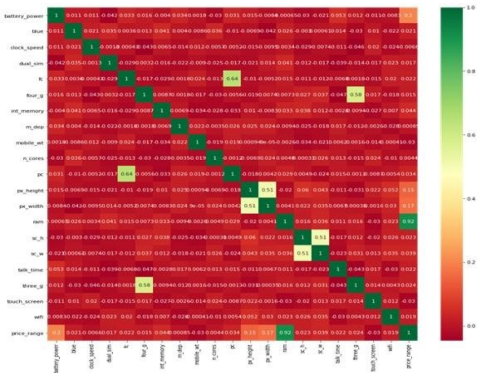
Рисунок 2.1 – Корреляция признаков между собой и целевой переменной После этого выбирается подмножество признаков с наилучшими параметрами на обучающей выборке, а затем он тестируется на тестовом сете.
