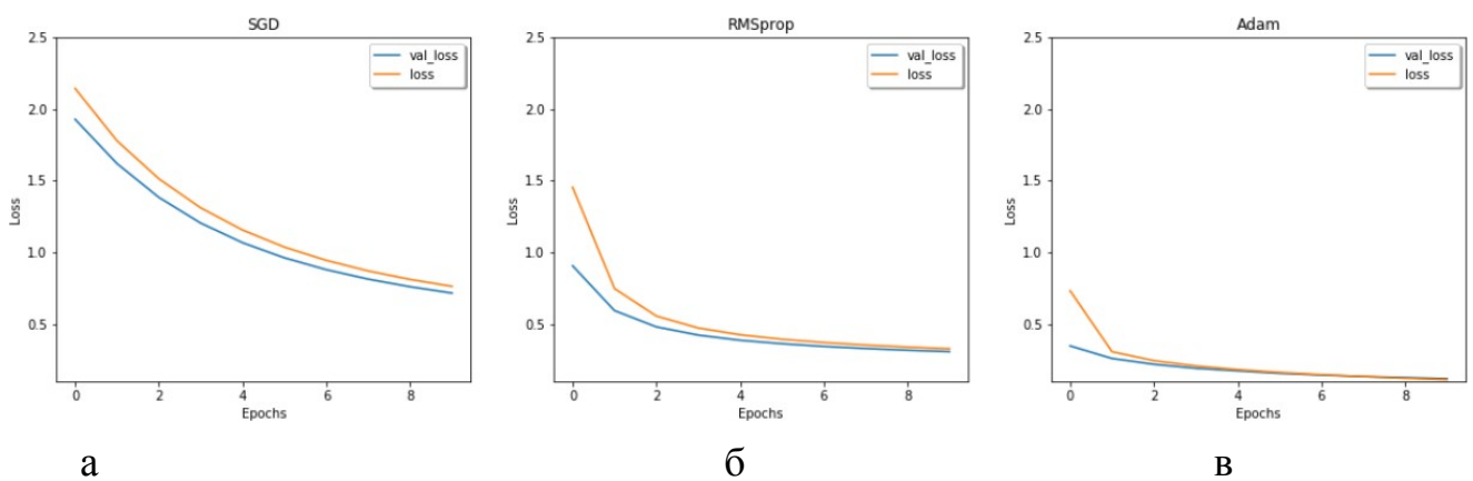
Рисунок 6.13 – Значения функции ошибок по эпохам обучения модели распознавания цифр при использовании в качестве алгоритма оптимизации: стохастического градиентного спуска (а), RMSprop (б), Adam (в)
