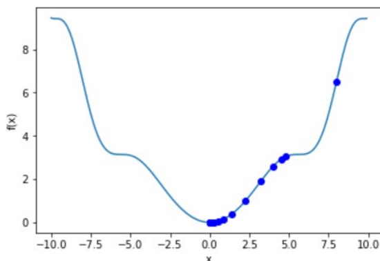
Рисунок 6.9 – Приближенные решения на различных итерациях градиентного спуска при поиске минимума функции f(x) = 0,1x^2 + \sin(0,1x^2)
