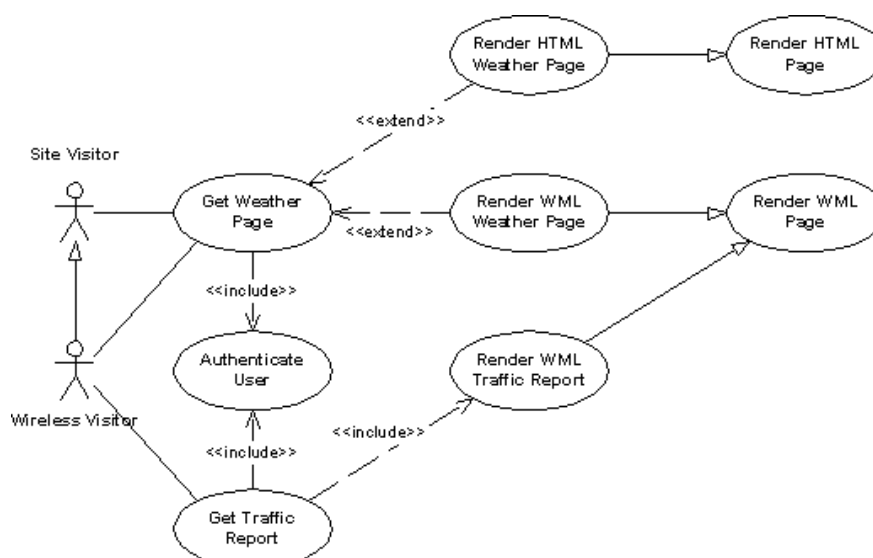
Рис.2: Диаграмма блоков-действий
