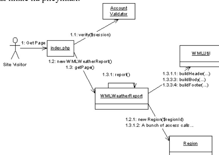
Рис. 6. Диаграмма взаимодействия.
