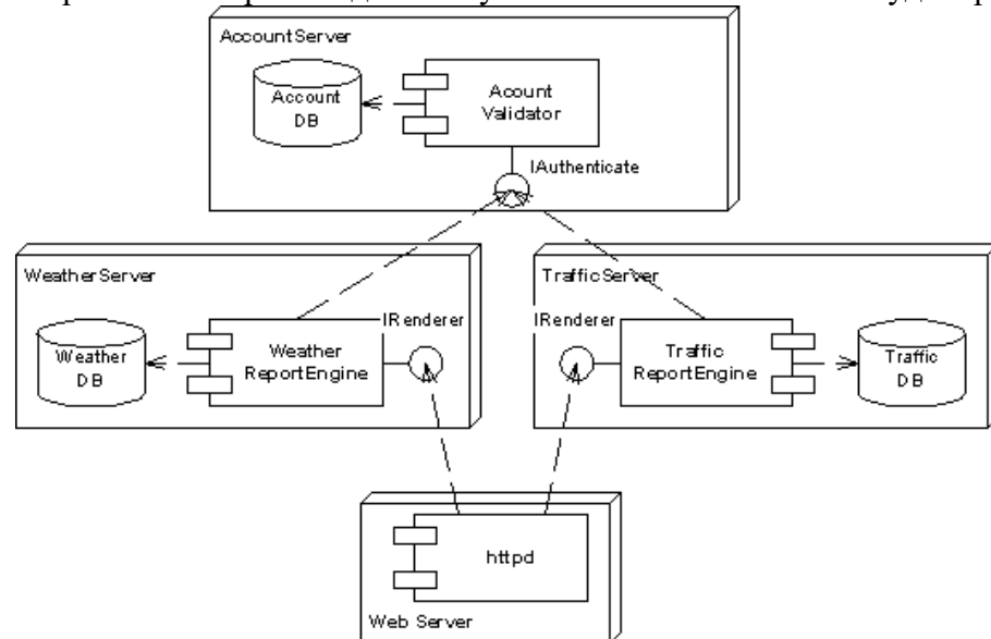
Рис.8: Диаграмма компонентов
