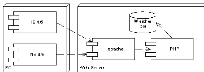
Рис. 4: Диаграмма архитектуры
