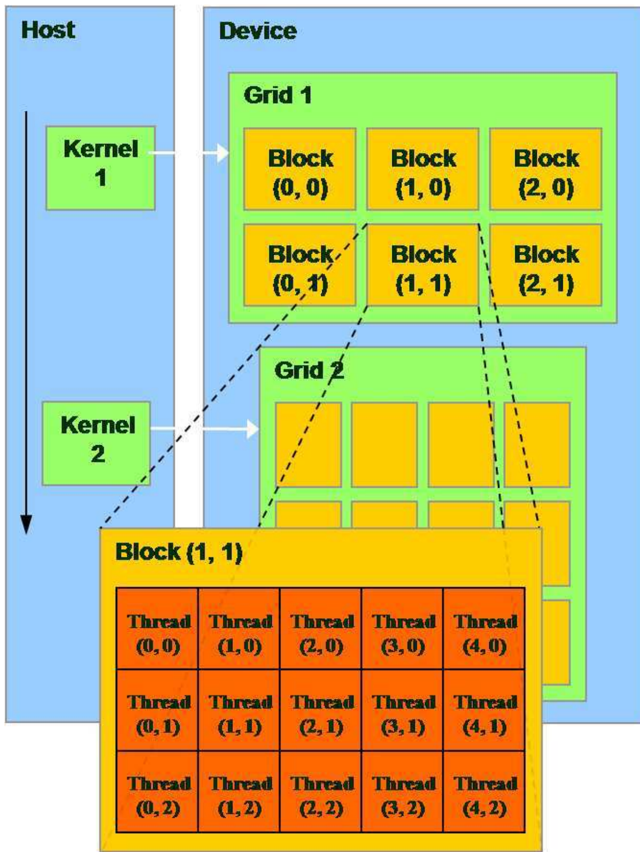
Рис. 18 – Архитектура CUDA
