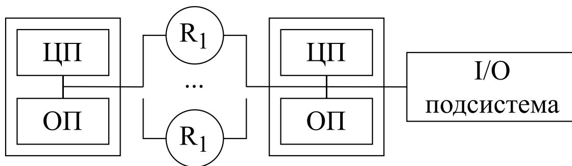
Рис. 6 – Архитектура ММР
