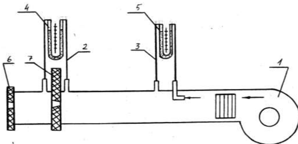
Рисунок 6 – Схема установки
