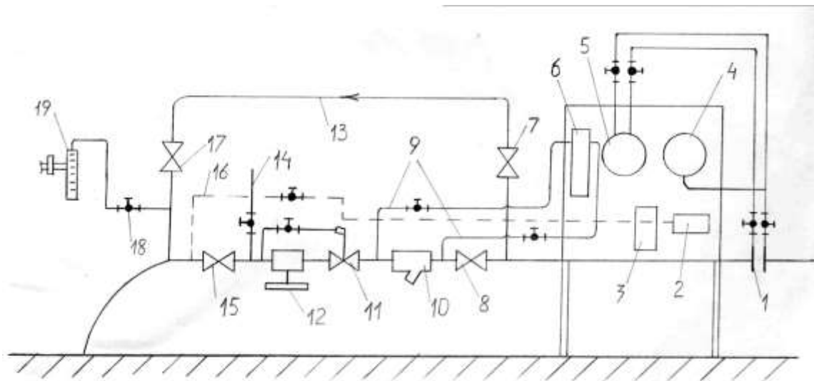
Рисунок 1- Схема ГРП
