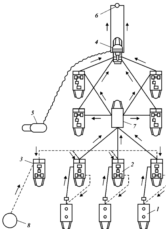
Рис. 16.2. Схема обвязки агрегатов при цементировании облегченным раствором с использованием осреднительной емкости и резервуара для заготовки жидкости затворения:
