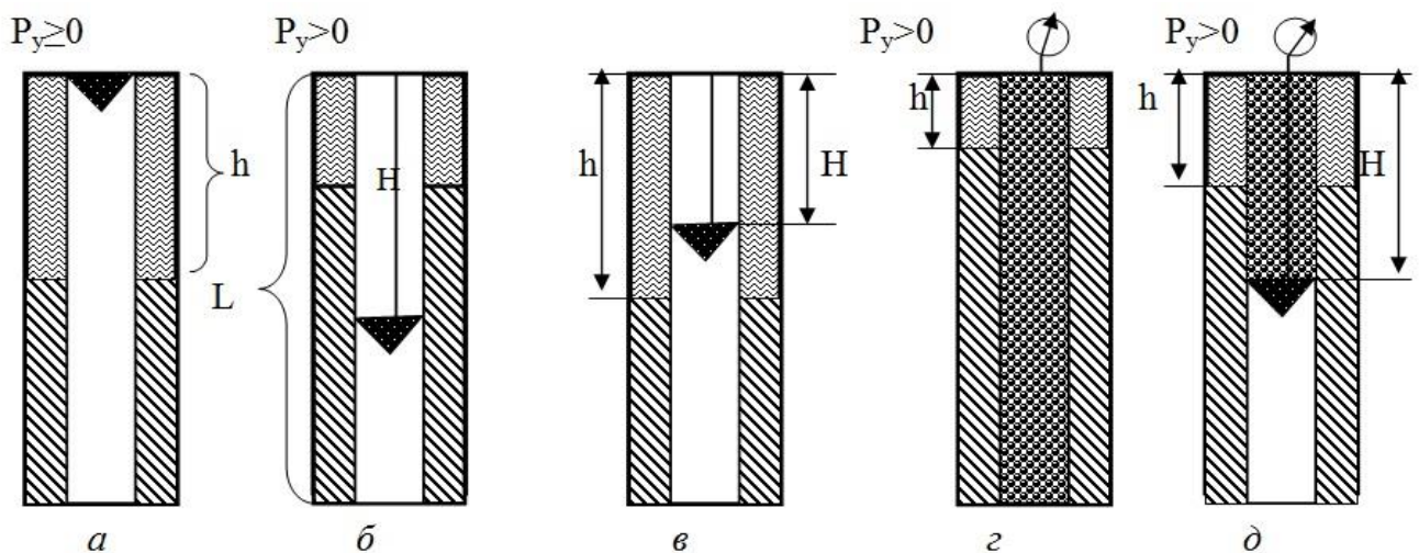
Рисунок 5.1 - Схемы уровней жидкостей в скважине
