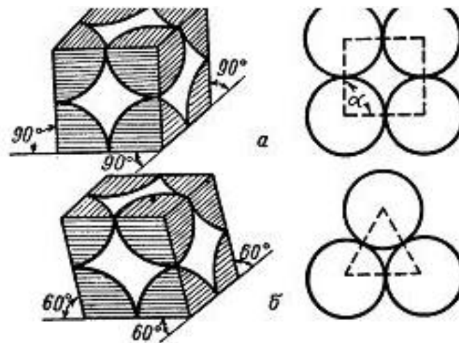
Рисунок 1.2 – Плотная и свободная укладка шаров фиктивного грунта
