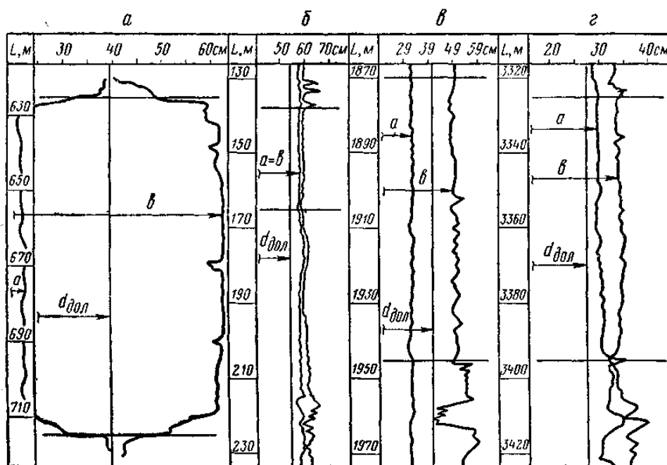
Рисунок 11.2 – Примеры профилеграмм по скважинам
