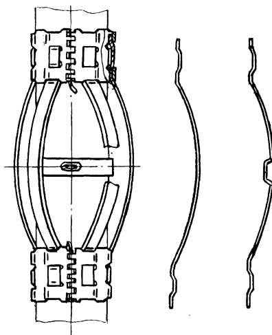
Рисунок 9.5 - Центратор типа ЦЦ
