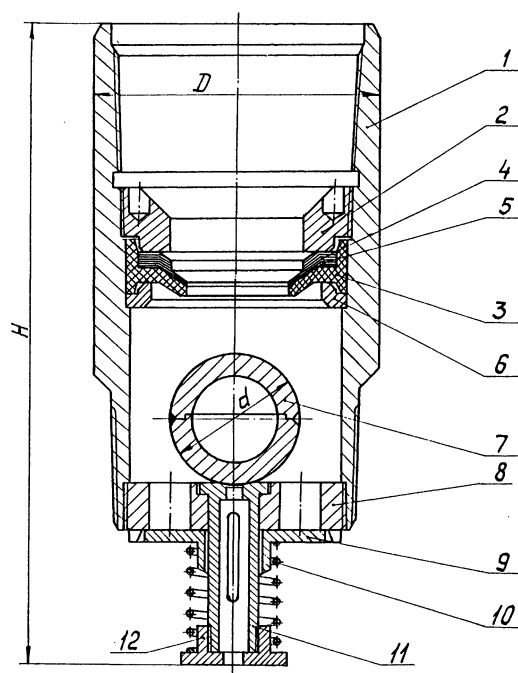
Рисунок 9.3 - Клапан обратный дроссельный модернизированный ЦКОДМ:
