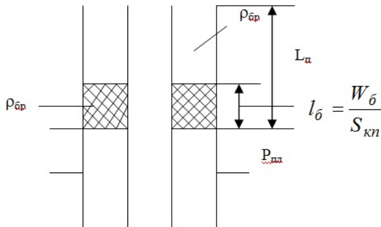
Рисунок 13.1 – Расчетная схема для определения баланса давлений
