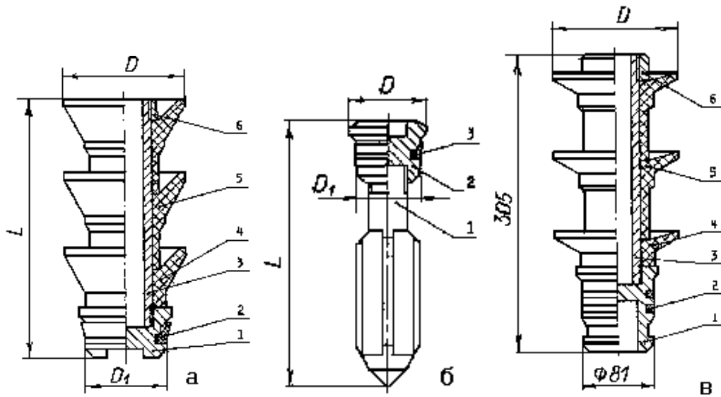
Рисунок 9.8 - Пакер проходной гидравлический универсальный за колонный типа ППГУ:
