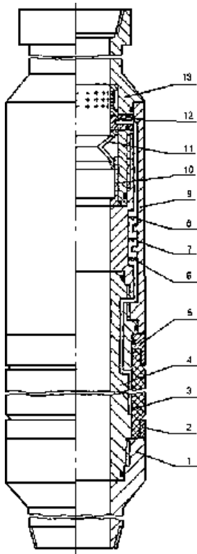
Рисунок 9.8 - Пакер проходной гидравлический универсальный за колонный типа ППГУ:
