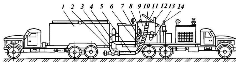
Рис. 16.5. Технологическая схема приготовления и нагнетания вспененных растворов:
