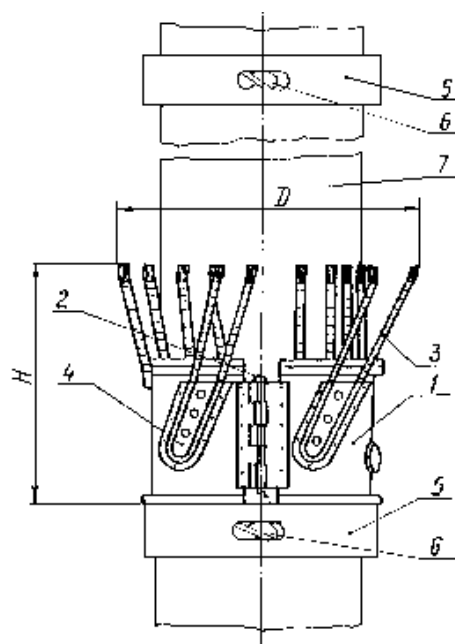
Рисунок 9.6 - Скребок корончатый типа СК:
