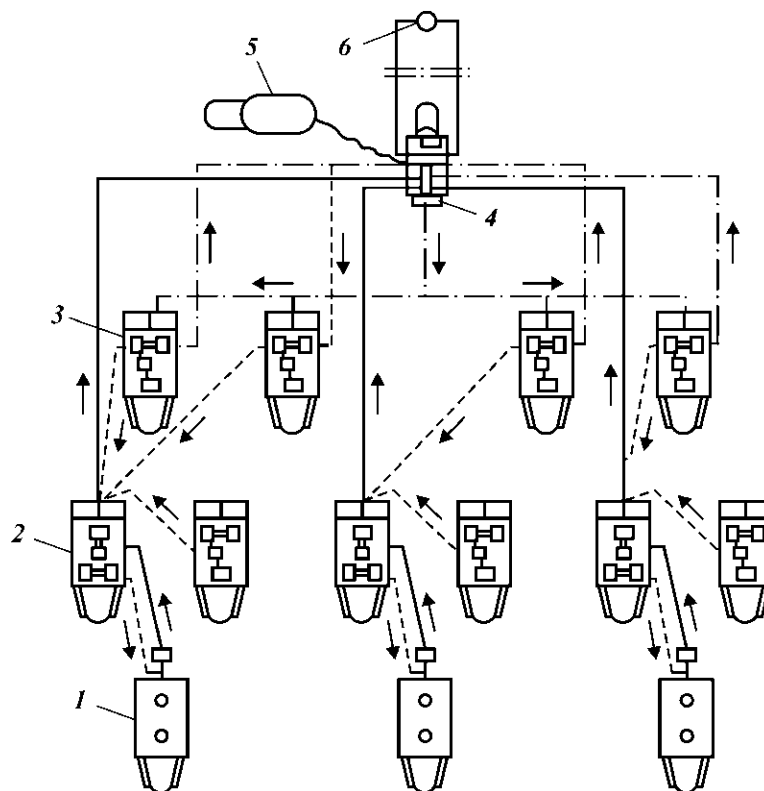
Рис. 16.4. Схема обвязки оборудования при цементировании с использованием для аккумуляции жидкости затворения мерных емкостей цементировочных агрегатов. Обозначения см. на рис. 14.1
