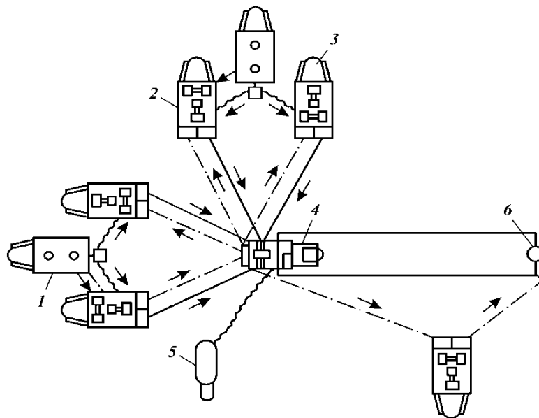
Рис. 16.1. Схема обвязки агрегатов при цементировании скважин с использованием 20—40 т сухого тампонажного материала:
