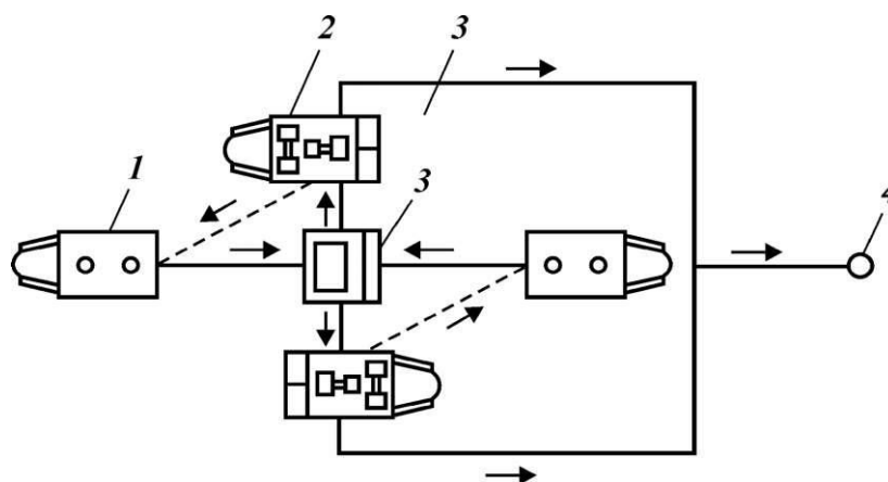
Рис. 16.6. Технологическая схема приготовления и закачки тампонажных растворов с применением фрезерно-струйной мельницы:
