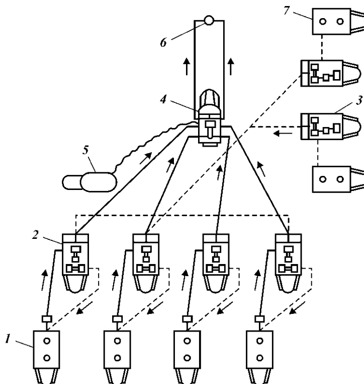
Рис. 16.3. Схема обвязки агрегатов с использованием двух емкостей для аккумуляирования жидкости затворения вместимостью по 25 м 3 : 1 - цементно-смесительная машина 2СМН-20; 2,3 - цементирующий агрегат соответственно ЦА-320М и 3ЦА-400А; 4 - блок манифольда 1БМ-700; 5 - станция контроля цементирования СКЦ-2М; 6 - цементировочная головка; 7 - емкость
