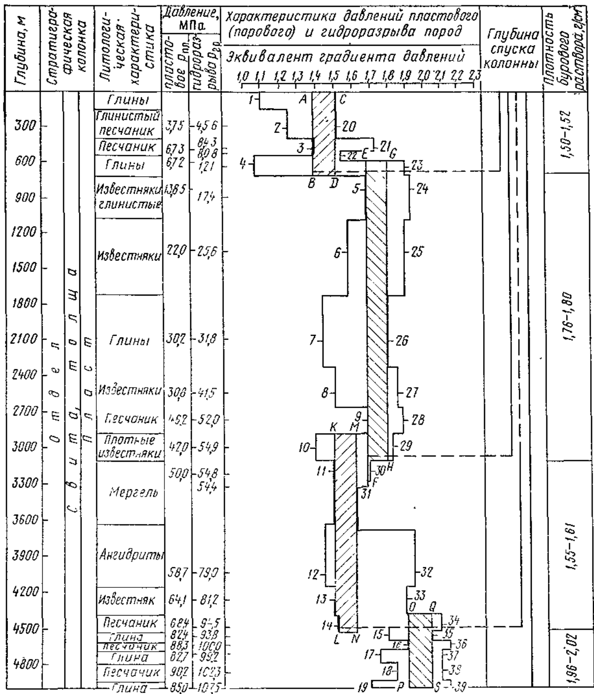
Рисунок 4.1 – Совмещенный график давлений для выбора конструкции скважины
