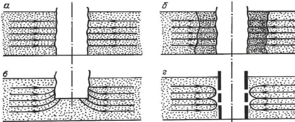
Рисунок 3.1 - Схемы притока в гидродинамически совершенную (а) и гидродинамически несовершенные скважины по качеству (б), степени (в) и характеру (г) вскрытия продуктивного горизонта.
