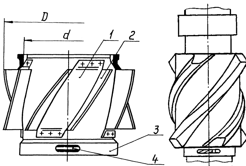
Рисунок 9.7 - Центраторы-турбулизаторы с упругими (ЦТ) и жесткими (ЦТГ) лопастями; 1-накладки; 2-упругие лопасти; 3-корпус; 4-винтовой клин.
