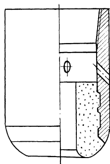
Рисунок 9.1 - Башмак колонный БКМ-146
