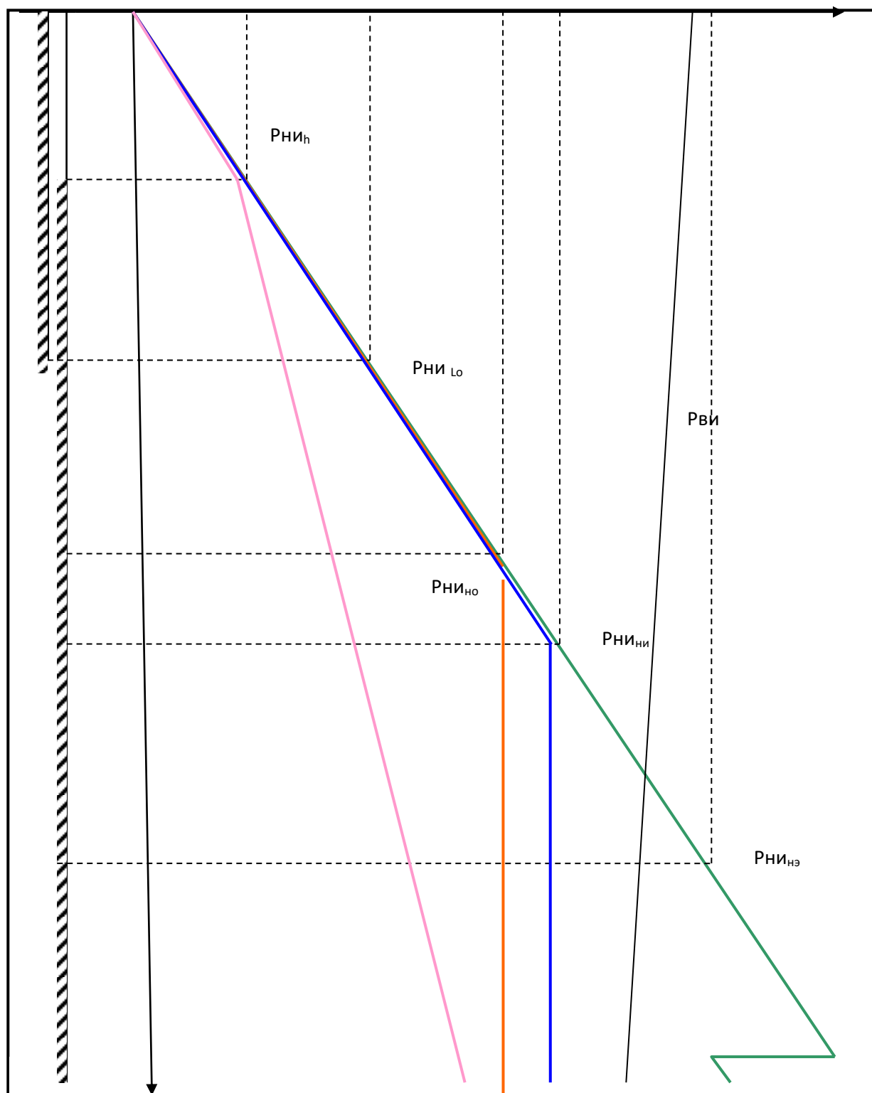
Рисунок 4.1 - Эпюры избыточных наружных давлений
