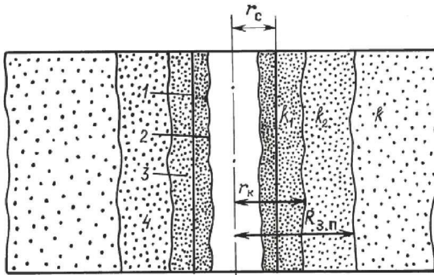
Рисунок 3.2 - Схемы прискважинной зоны пласта после вскрытия его бурением:
