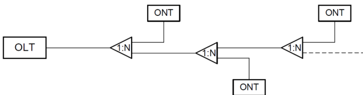
Рисунок 5 – Топология «шина»
