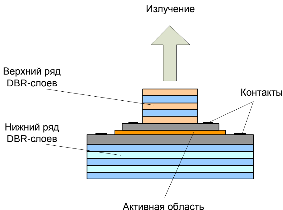
Рисунок 5 – Структура VCSEL-лазеров
