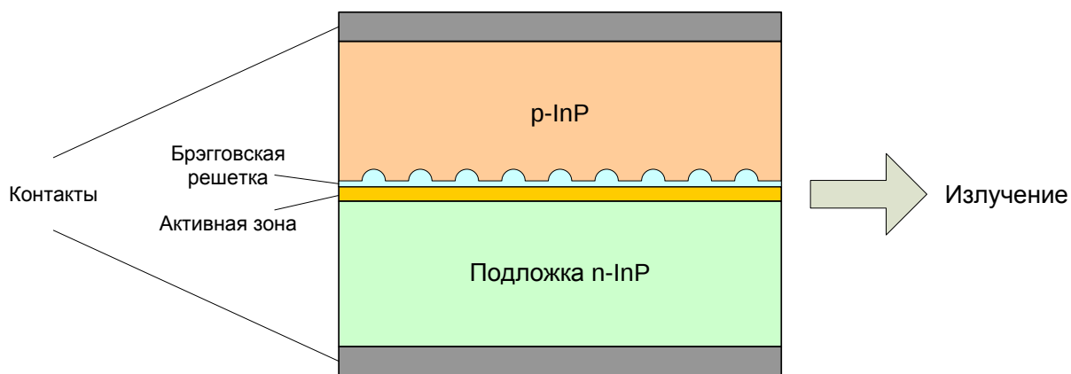
Рисунок 3 – Структура DFB-лазеров
