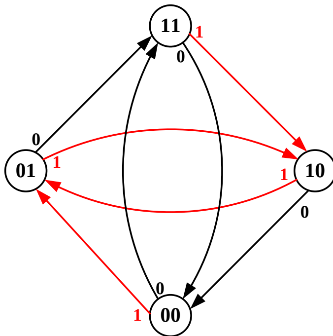
Рисунок 2 – Граф формирования кодовых комбинаций кода Миллера
