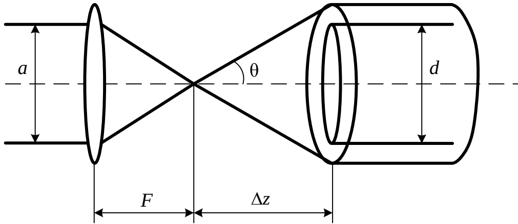
Рисунок 13 – Ввод излучения в оптоволокно
