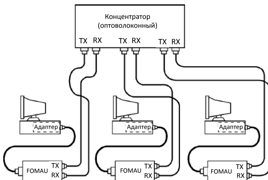
Рисунок 3 – Объединение компьютеров в сеть по стандарту 10BASE-FL
