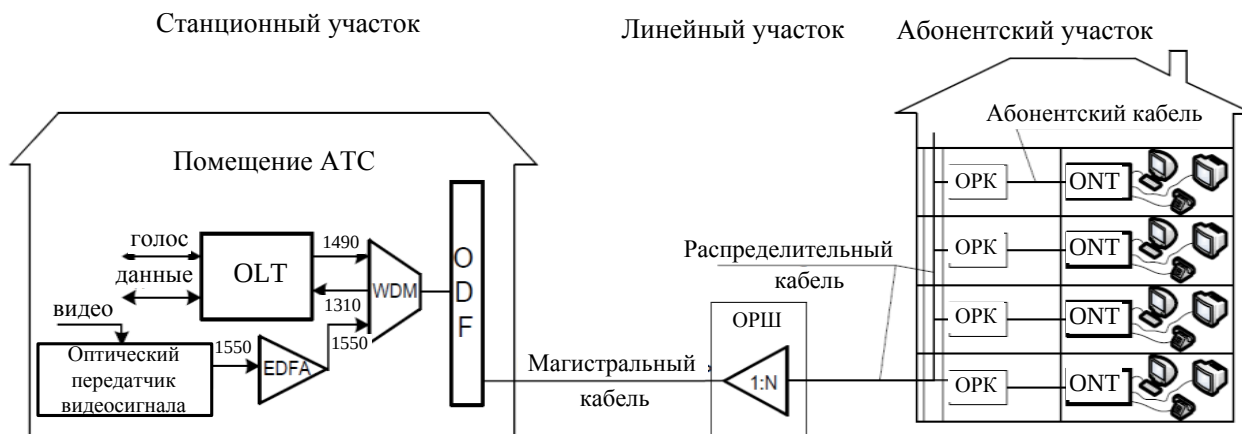
Рисунок 1 – Схема пассивной оптической сети
