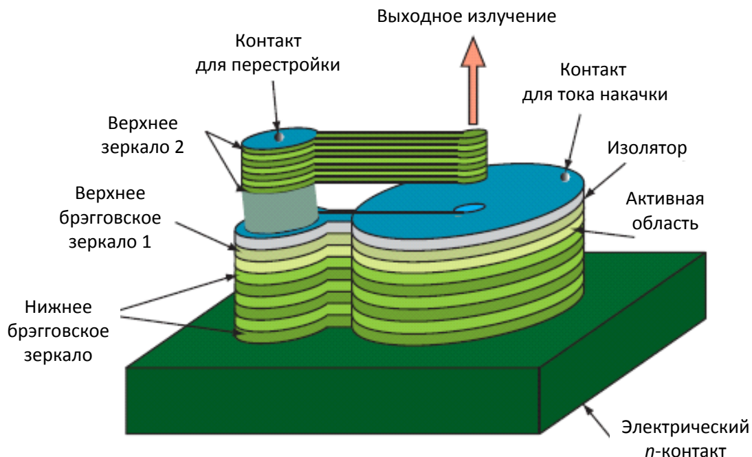
Рисунок 10 – Структурная схема перестраиваемого лазера консольного типа
