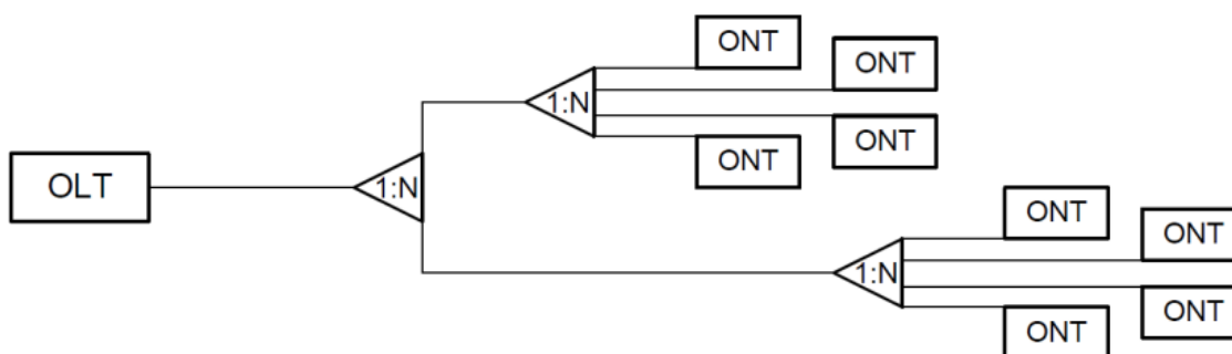
Рисунок 3 – Многоуровневая схема включения сплиттеров
