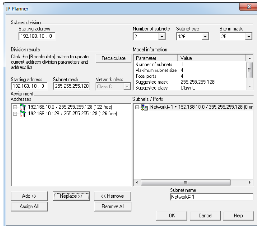
Рисунок 13 – Окно автоматического назначения IP-адресов
