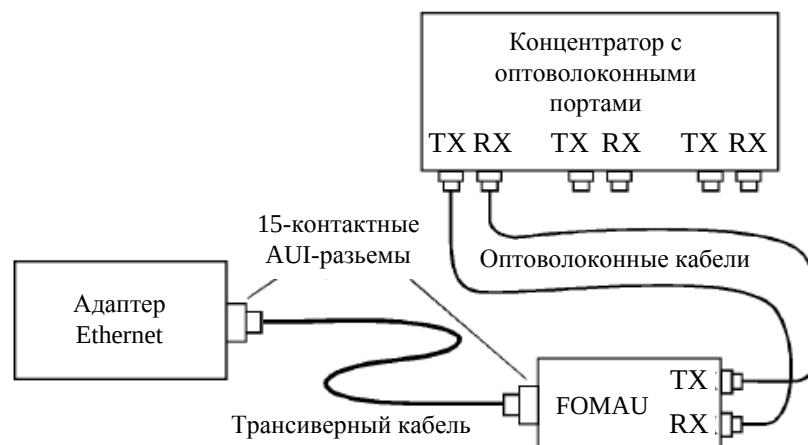
Рисунок 1 – Соединение адаптера и концентратора в 10BASE-FL
