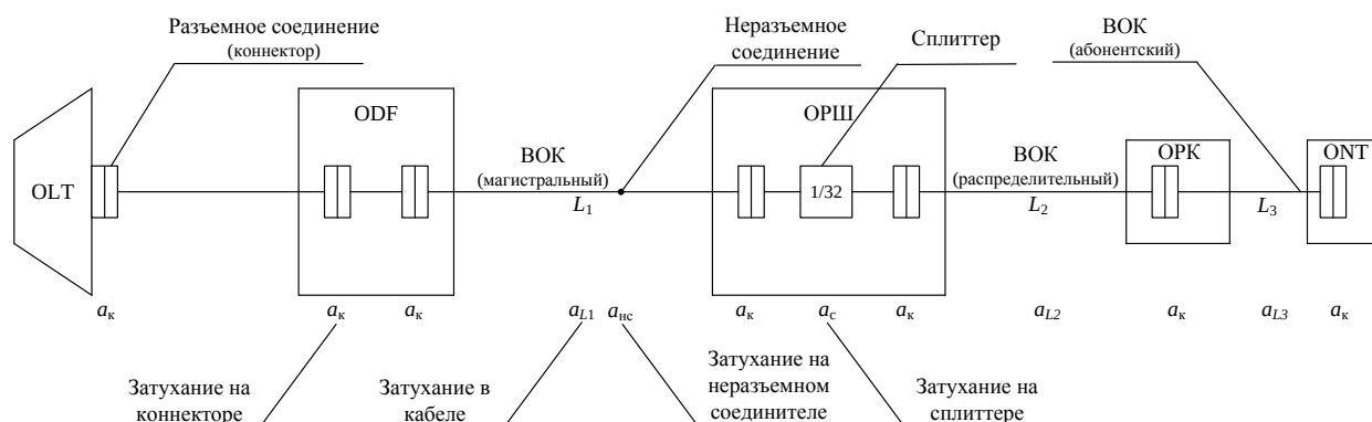
Рисунок 2 – Графический расчет оптического бюджета в сети xPON
