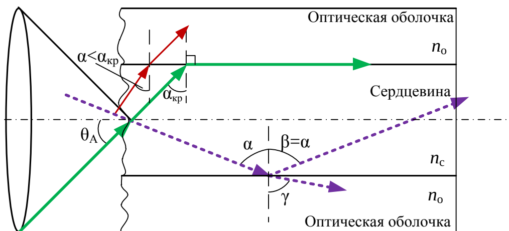
Рисунок 11 – Прохождение луча через границу раздела двух сред
