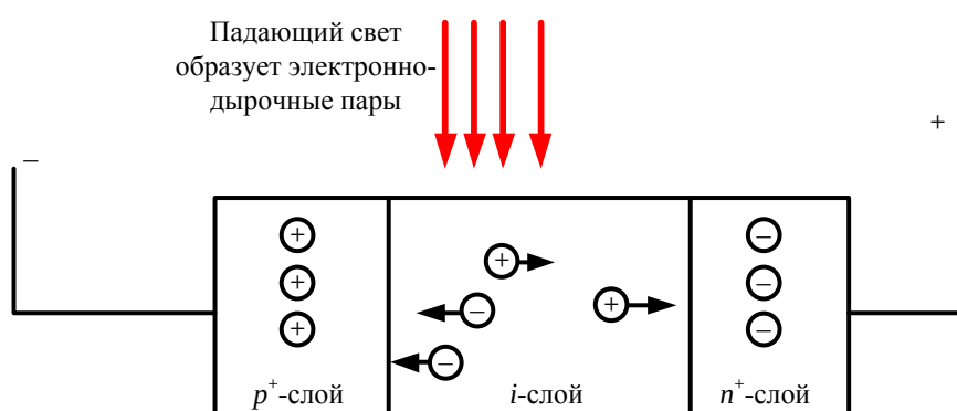
Рисунок 1 – Схема структуры p-i-n -фотодиода
