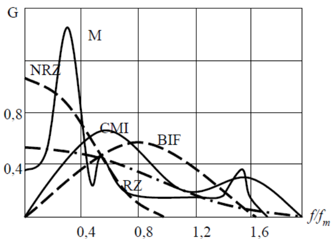
Рисунок 3 – Энергетические спектры линейных кодов
