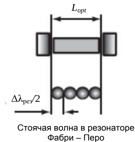
Рисунок 6 – Схема лазера с резонатором Фабри – Перо
