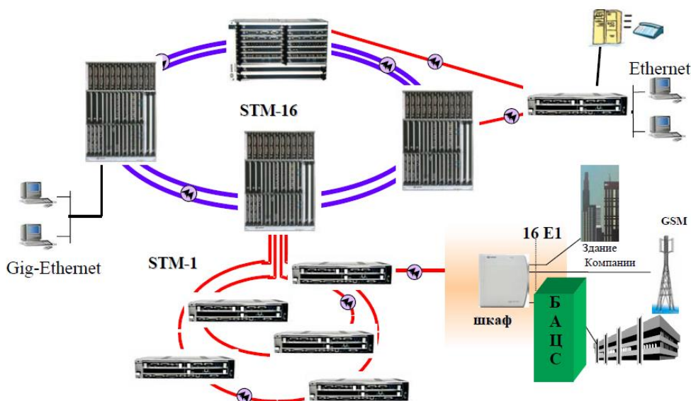
Рисунок 8 – Организация сети с помощью мультиплексора ОЛТ-2500 eXtra
