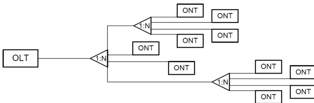
Рисунок 6 – Топология «дерево»
