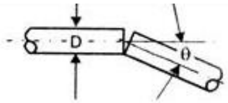
Рисунок 2 – Угловое смещение оптических волокон
