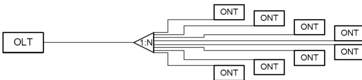
Рисунок 2 – Одноуровневая схема включения сплиттеров
