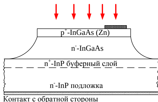
Рисунок 3 – Обобщенная схема PIN-фотодиода на основе InGaAs
