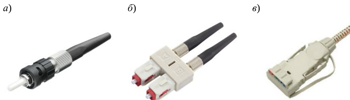
Рисунок 2 – Типы разъемов для оптоволоконного кабеля: а – ST-разъем, б – SC-разъем, в – MIC FDDI-разъем
