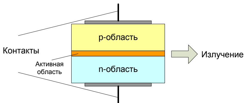
Рисунок 2 – Структура лазеров с резонатором Фабри – Перо
