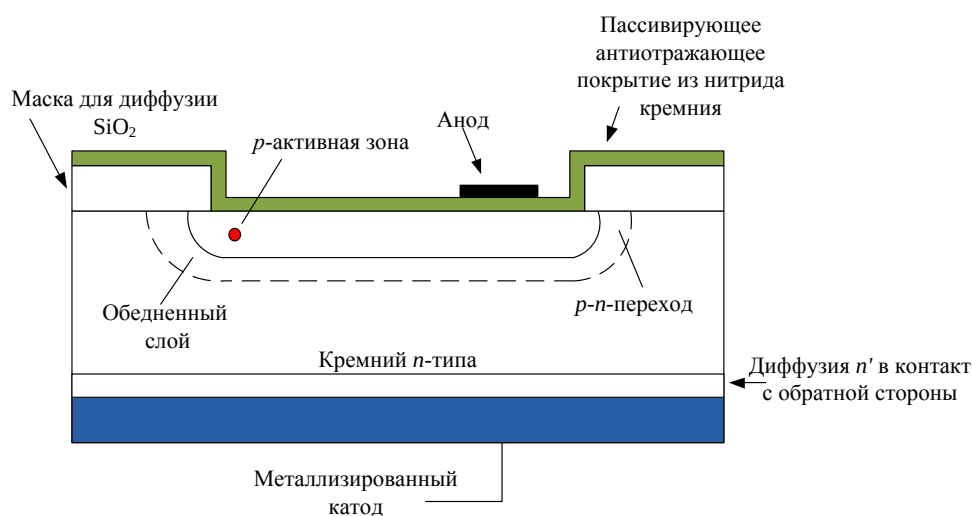
Рисунок 2 – Поперечное сечение кремниевого фотодиода
