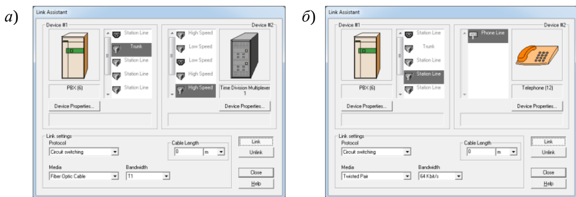
Рисунок 12 – Соединение мультиплексоров и АТС (а), АТС и телефонного аппарата (б)
