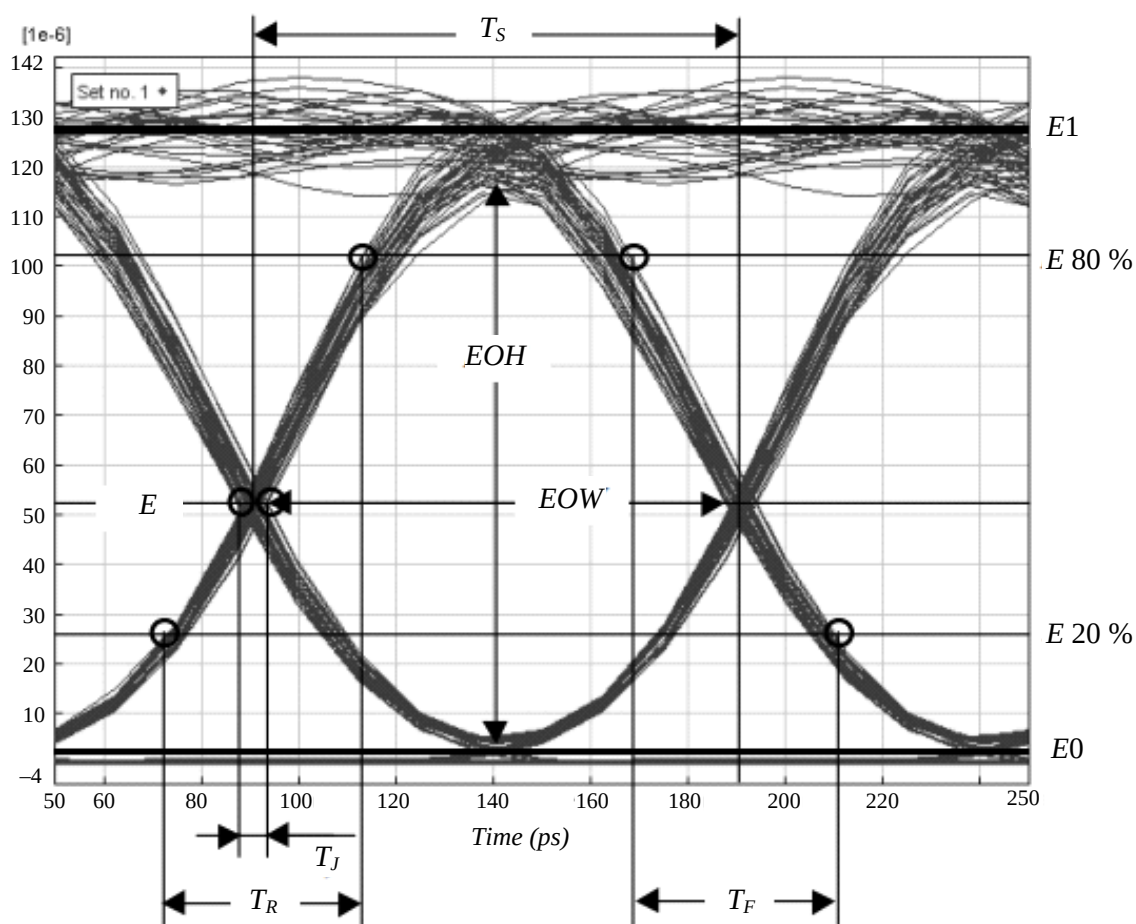
Рисунок 6 – Глаз-диаграмма на экране осциллографа
