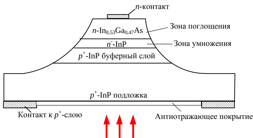
Рисунок 4 – Поперечное сечение типичной гетероструктуры лавинного фотодиода
