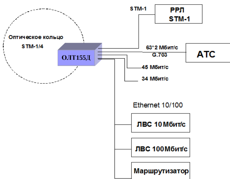
Рисунок 4 – Сетевые интерфейсы ОЛТ-155Д
