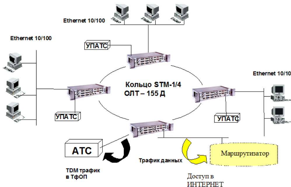
Рисунок 2 – Кольцевая топология
