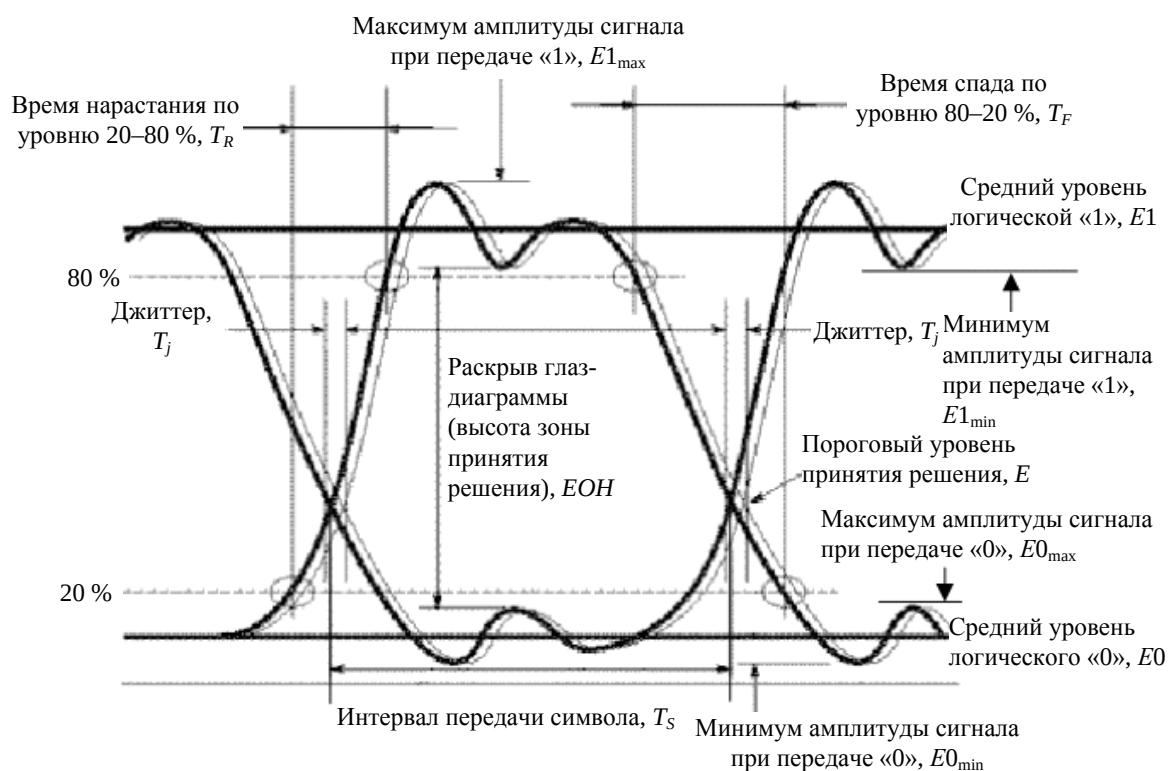
Рисунок 5 – Идентификация глаз-диаграммы
