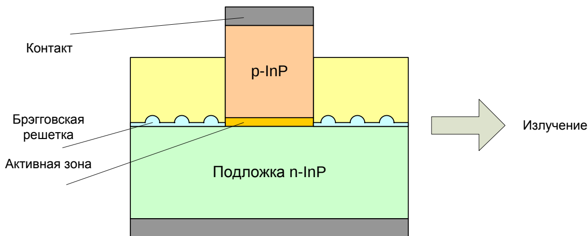
Рисунок 4 – Структура DBR-лазеров
