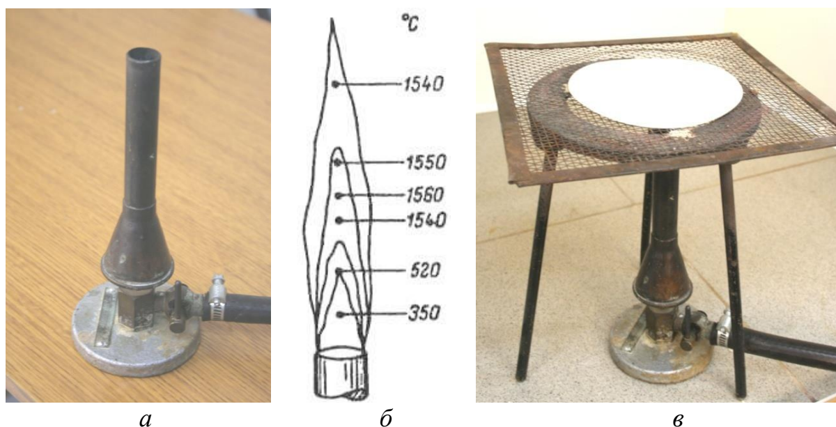
Рисунок 12. Горелка Теклю (а), распределение температуры в пламени газовой горелки (б) и штатив-подставка с асбестовой сеткой над горелкой (в)
