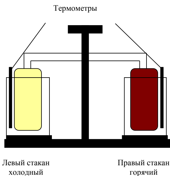
Рисунок 20. Установка для демонстрации влияния температуры на химическое равновесие
