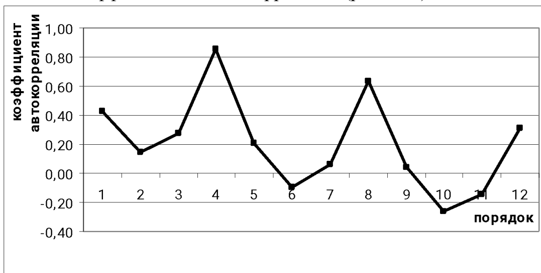
Рис. 11.2 Коррелограмма, построенная по квартальным данным (заметна сильная положительная корреляция между каждым четвертым кварталом)
