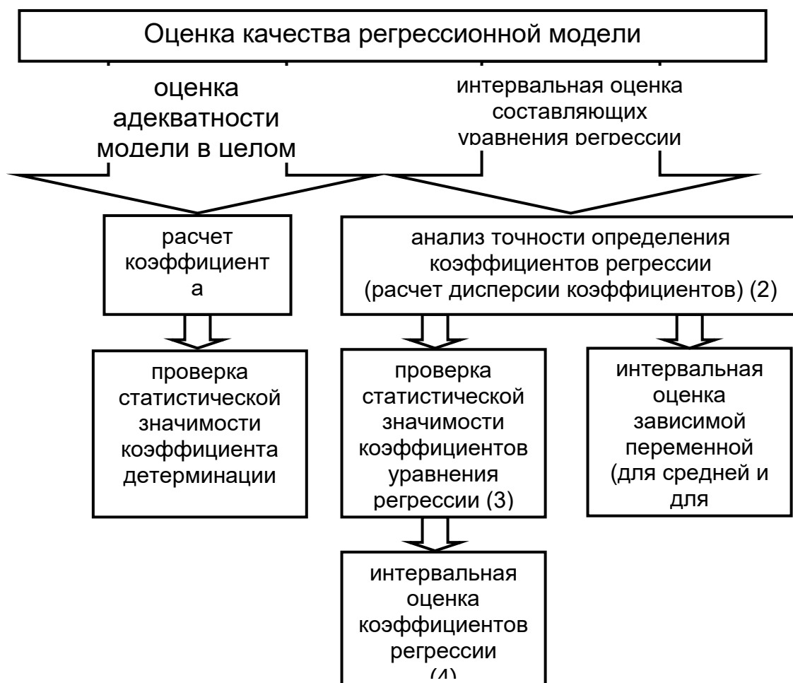
Рис. 6.2 Анализ качества регрессионной модели
