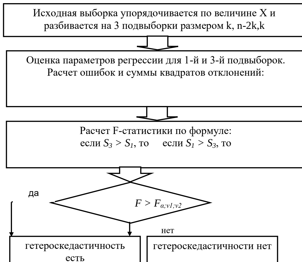
Рис.14.1 Алгоритм применения теста Голдфельда-Квандта
