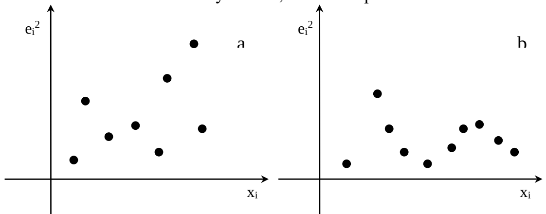
Рис. 13.3 Невозможность установления гетероскедастичности при помощи графического анализа остатков
