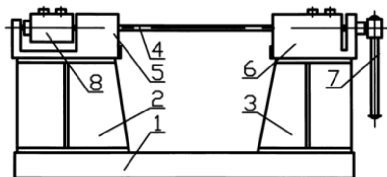
Рисунок 8.1 – Установка для испытания стержня на устойчивость
