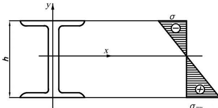
Рисунок 5.2 – Эпюра нормальных напряжений в поперечном сечении балки
