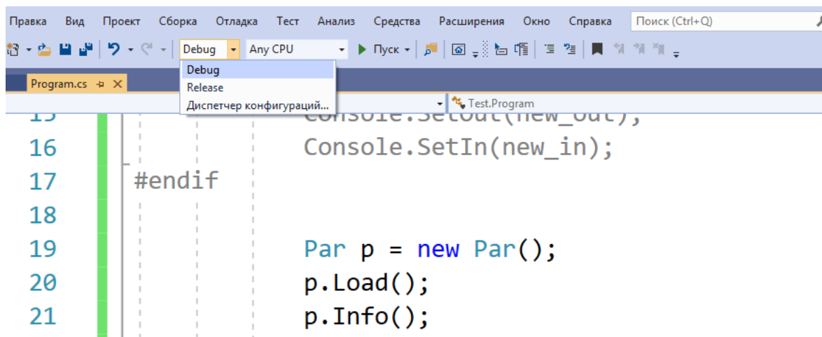
Рисунок 6.5 – Настройки конфигурации
