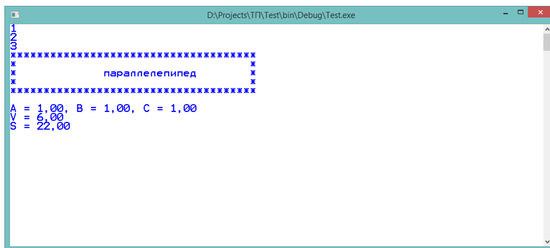
Рисунок 6.6 – Выполнение debug-приложения
