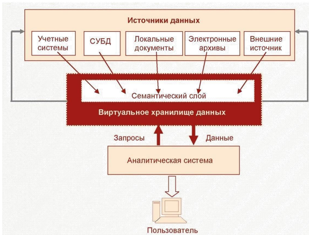
Рис.4.11 Виртуальное ХД.
