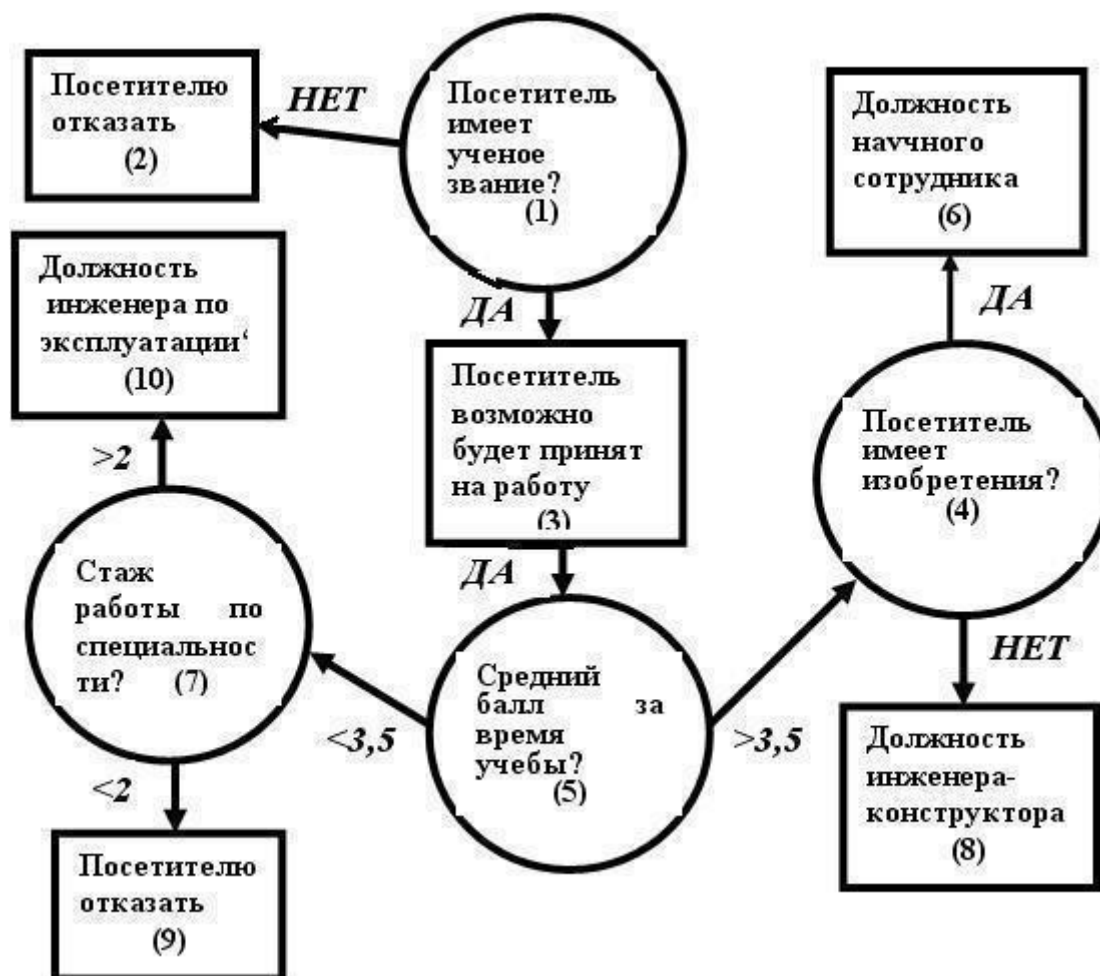
Рис.3.8. Дерево решений для выбора должности
