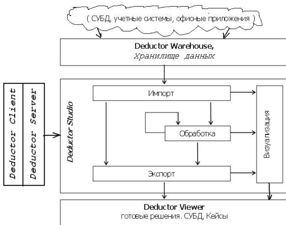
Рис.4.14 Архитектура Deductor.
