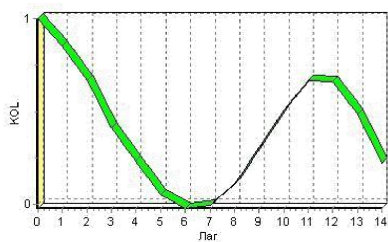
Рис. 1. Автокорреляция.
