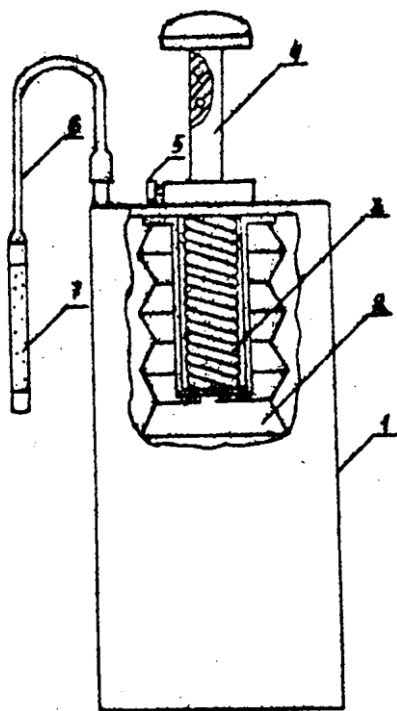
Рисунок 8.1 – Газоанализатор УГ-2:
