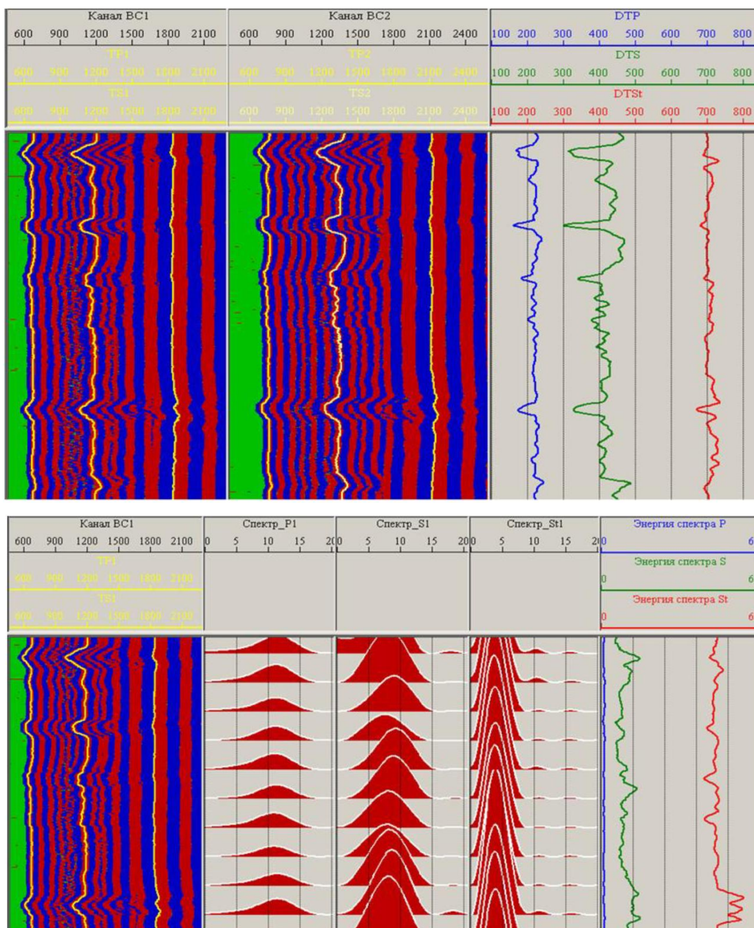
Рисунок 5 – Кинематические и динамические характеристики акустических волн
