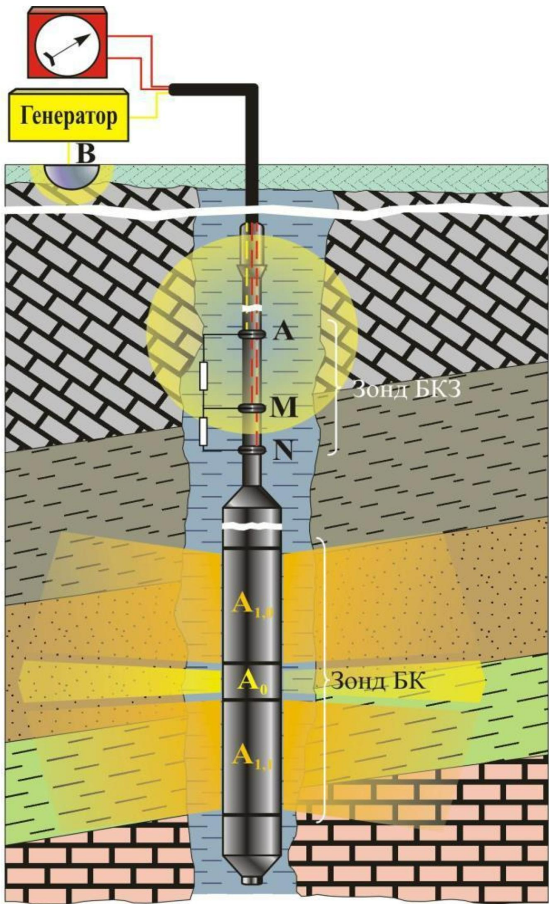
Рисунок 2 – Схема замера зондом БК
