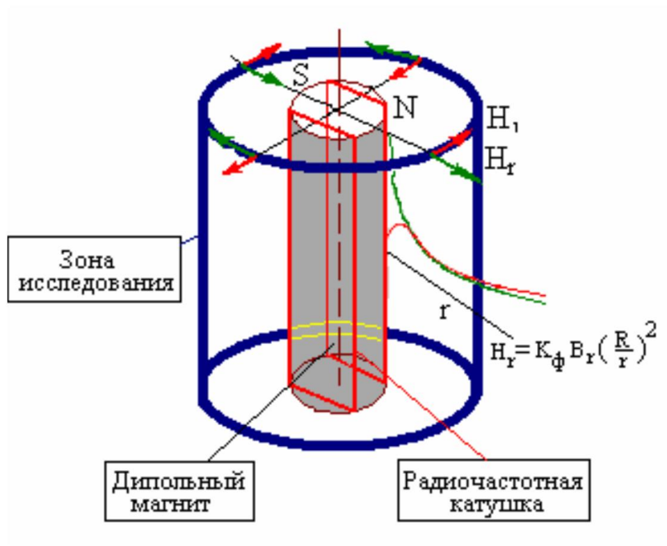
Рисунок 5 – Ядерно-магнитный каротаж
