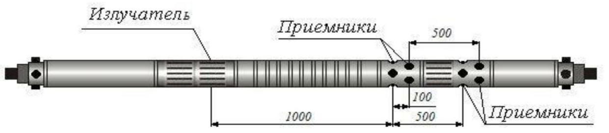
Рисунок 5 – Прибор АКЦ
