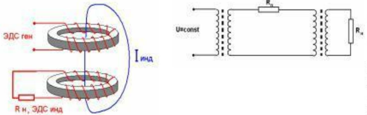
Рисунок 9 – Скважинный индукционный резистивиметр
