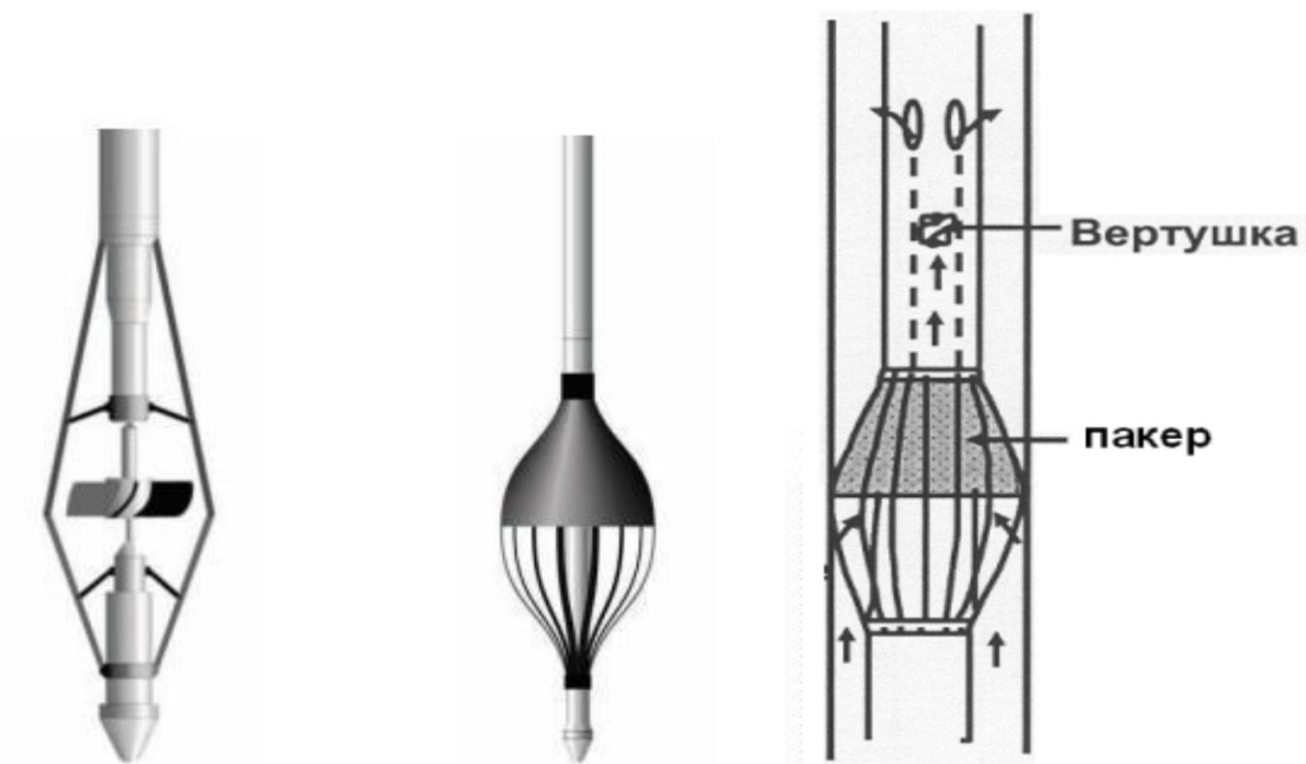
Рисунок 6 – Нефтяные турбинные расходомеры с пакером и без пакера
