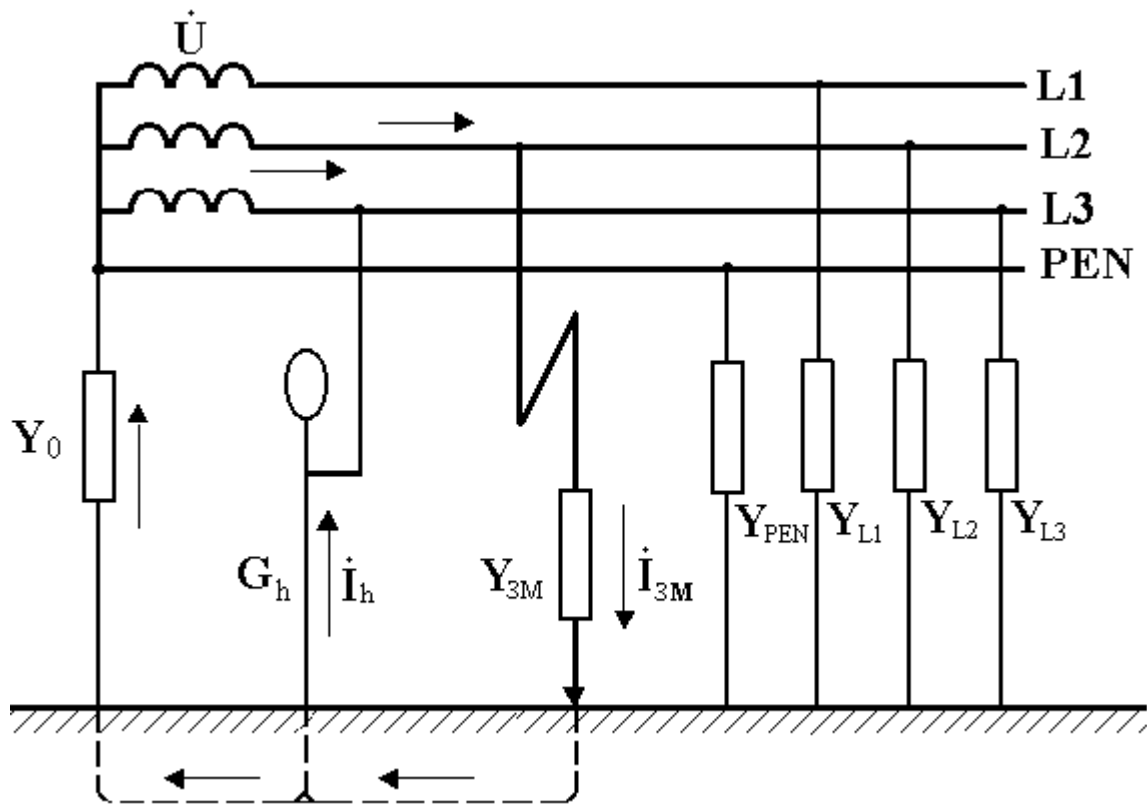
Рисунок 1.2 – Прикосновение к исправному проводу в сети с заземленной нейтралью типа TN-C при аварийном режиме работы
