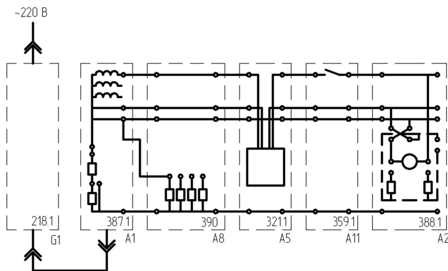
Рисунок 3.5 – Схема для выявления действия защиты при ошибочном соединении нулевых рабочего и защитного проводников
