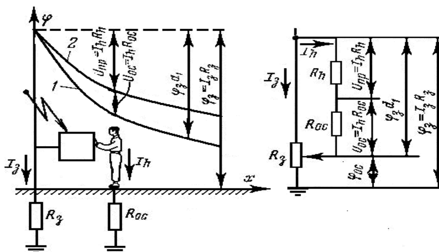
Рисунок 5.1 – К определению напряжения прикосновения с учетом падения напряжения в сопротивлении растеканию тока основания, на котором стоит человек:
