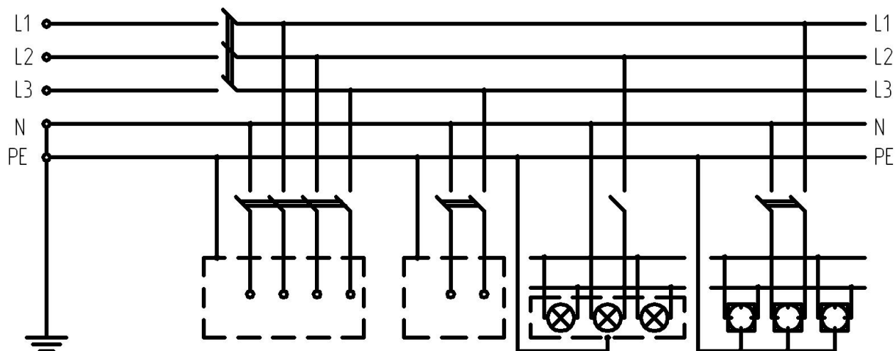
Рисунок 3.2 – Система TN-S
