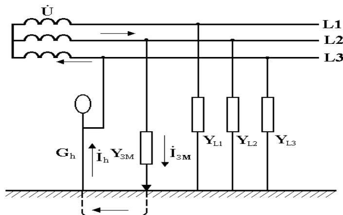
Рисунок 4.3 – Однофазное прикосновение к исправному проводу в сети с изолированной нейтралью типа ИТ при аварийном режиме работы
