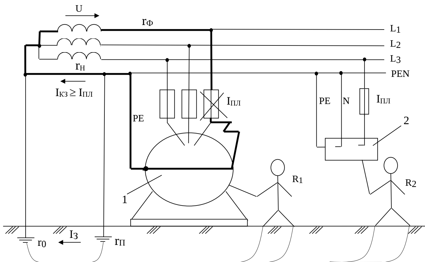
Рисунок 7.1 – Схема защитного зануления в системе TN - C :
