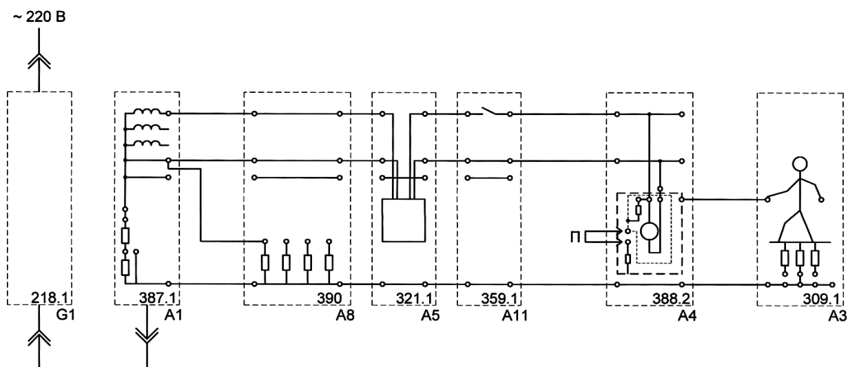
Рисунок 7.3 – Схема для выявления действия защиты при повреждении рабочей изоляции электроприемника класса II
