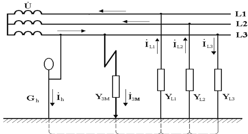
Рисунок 4.4 – Однофазное прикосновение к неисправному проводу в сети с изолированной нейтралью типа IT при аварийном режиме работы
