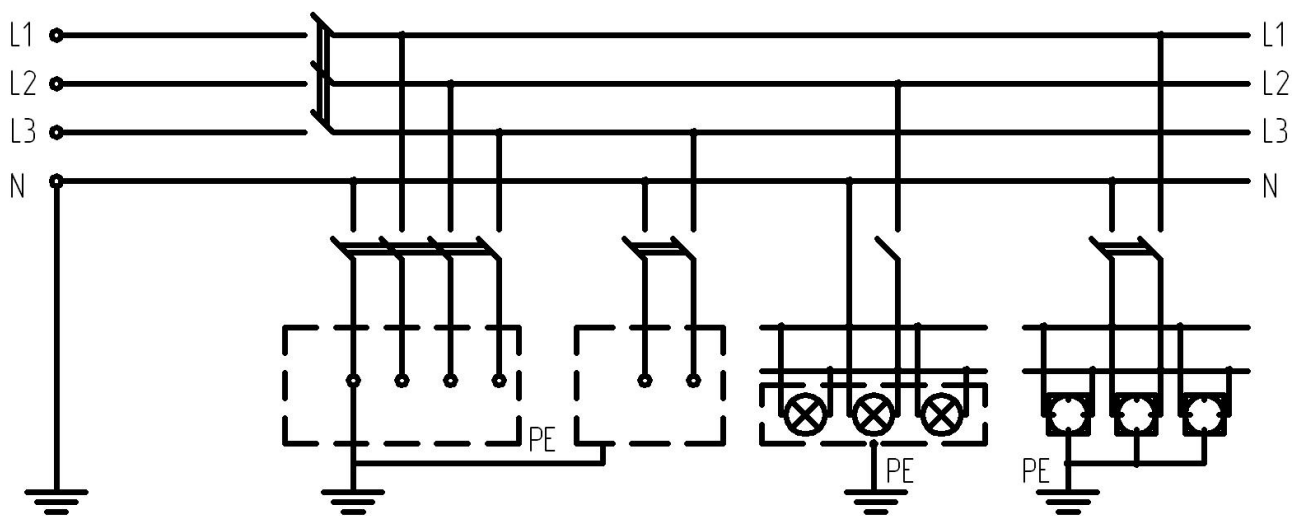
Рисунок 5.1 – Схема заземления TT
