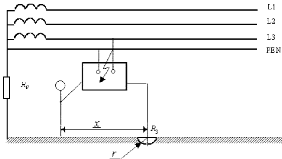
Рисунок 1.8 – Замыкание фазы на заземленный корпус в сети TN - C
