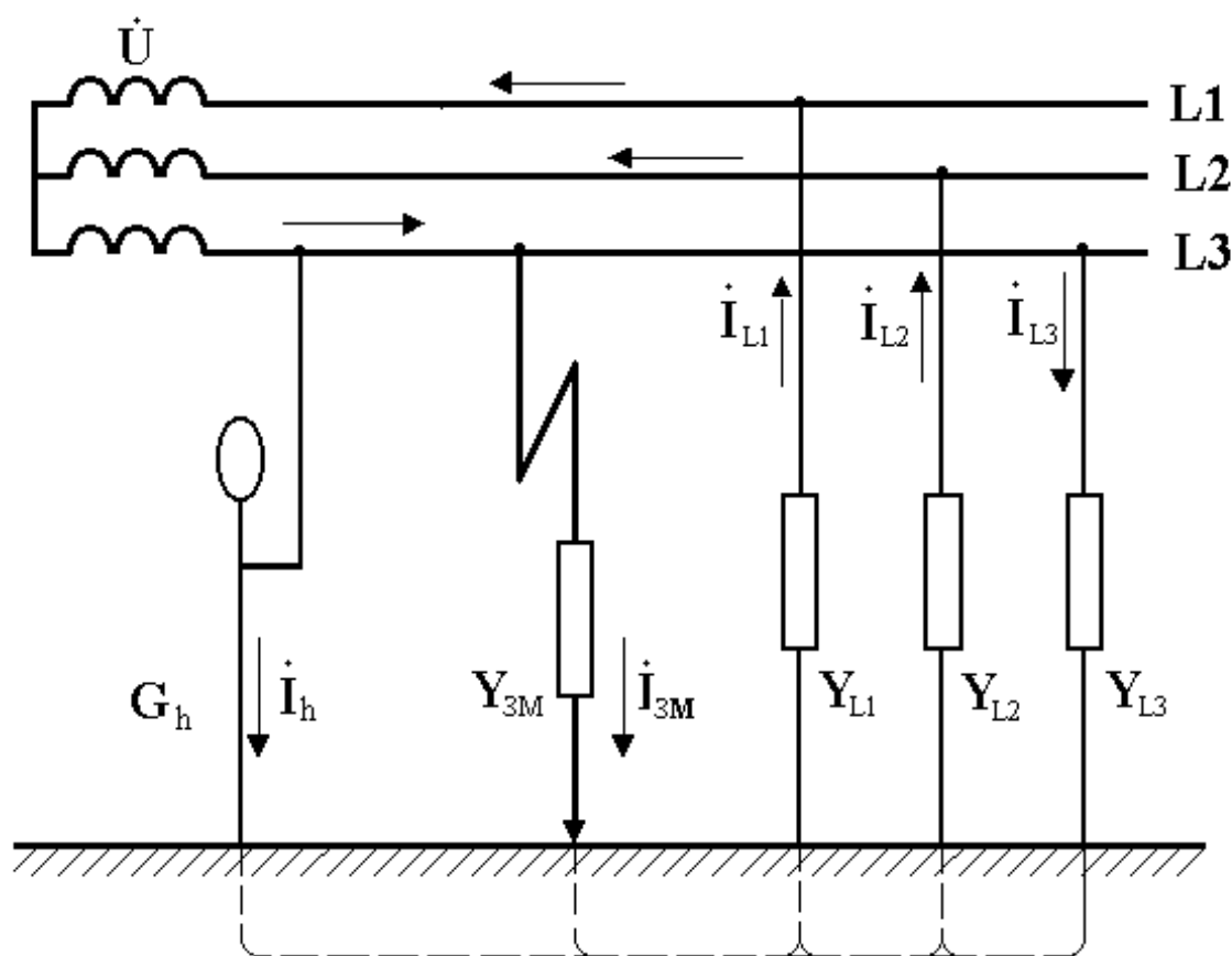
Рисунок 6.5 – Однофазное прикосновение к неисправному проводу в сети с изолированной нейтралью типа IT при аварийном режиме работы
