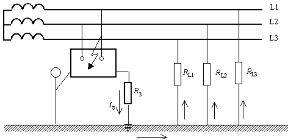
Рисунок 1.6 – Замыкание фазы сети IT на заземленный корпус
