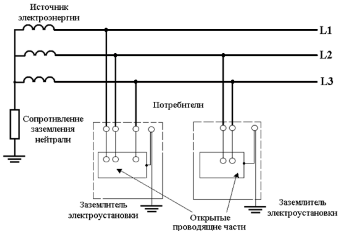
Рисунок 6.1 – Система IT
