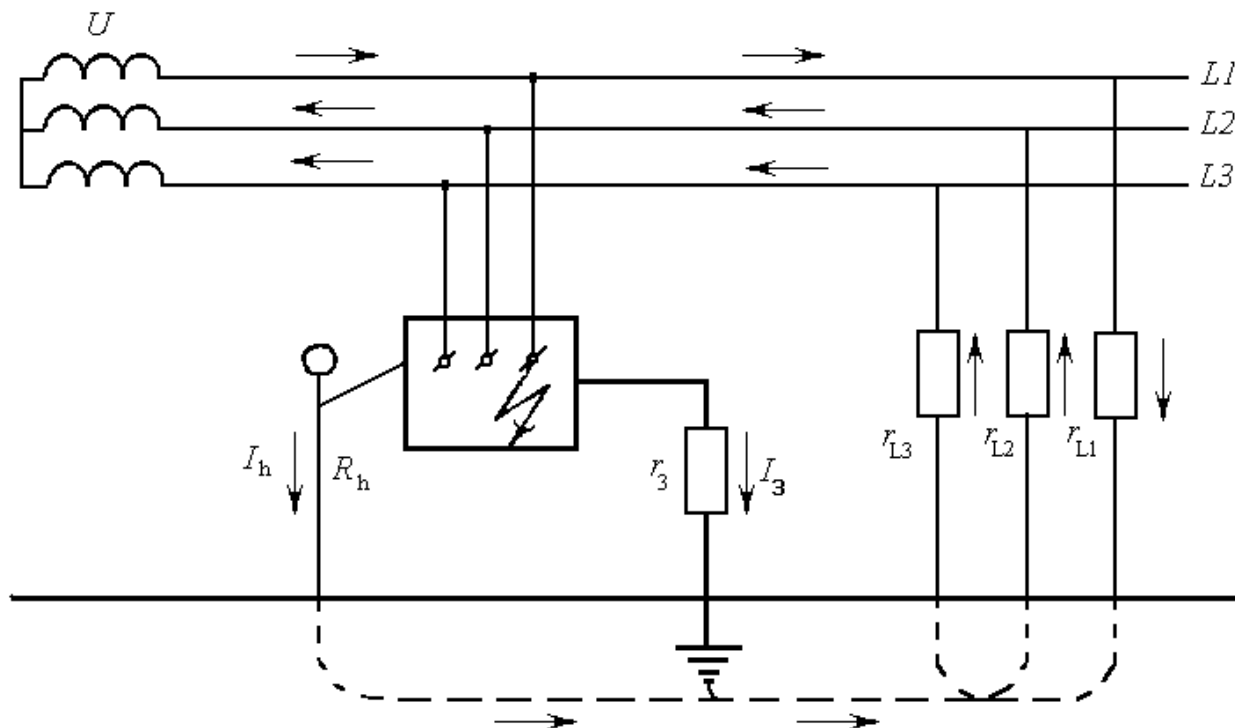
Рисунок 1.1 – Схема сети с изолированной нейтралью (типа IT ) и защитным заземлением электроустановки
