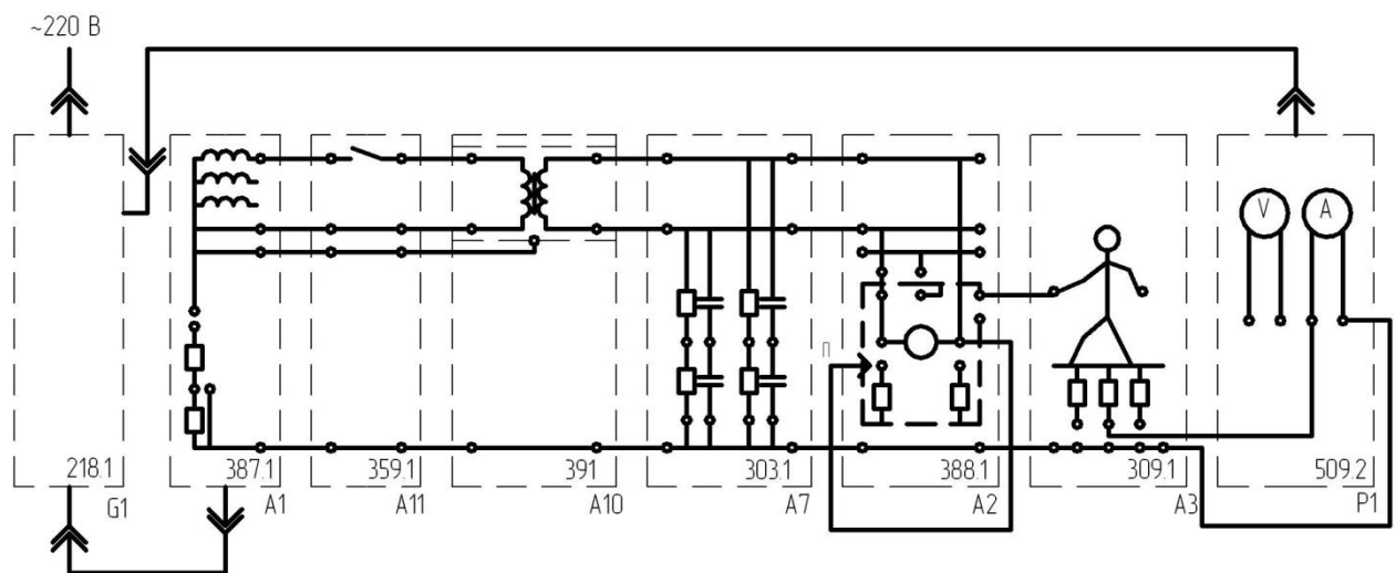
Рисунок 6.3 – Схема для выявления действия защиты при повреждении рабочей изоляции электроприемника класса 01 (снижении сопротивления изоляции фазы до 1 Ом)
