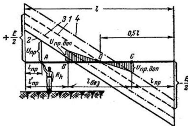
Рисунок 1.2.5 – Потенциальная характеристика незаземлённого провода к которому прикасается человек. 1 – до прикосновения человека к проводу;
