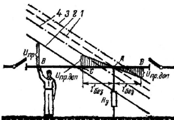
Рисунок 1.2.7 – Потенциальные характеристики провода заземлённого в одной точке A , до прикосновения к нему человека и после.
