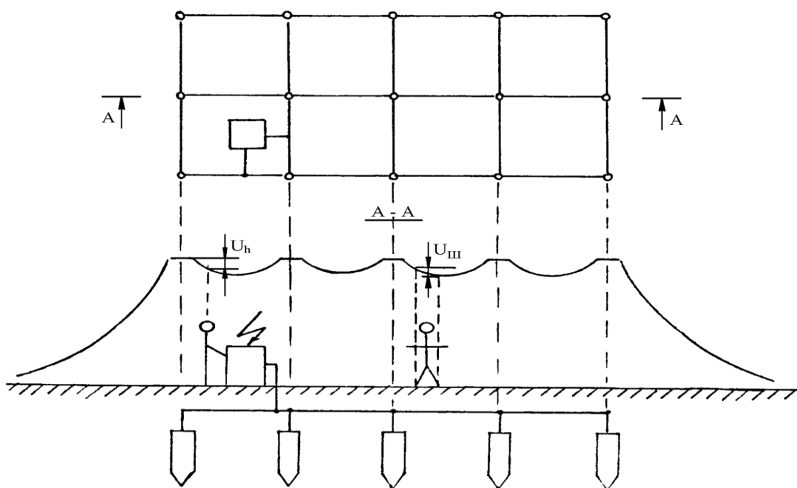
Рисунок 1.4 – Контурное заземляющее устройство
