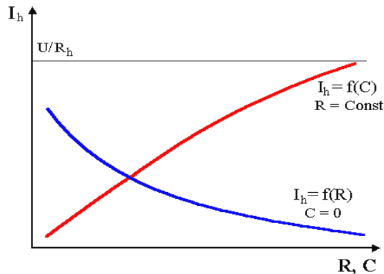
Рисунок 4.2 – Зависимость значения тока, протекающего через тело человека, прикоснувшегося к фазному проводу в сети ИТ с симметричными параметрами в нормальном режиме работы, от сопротивления изоляции и емкости фазных проводов относительно земли
