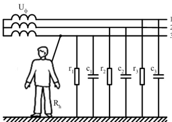
Рисунок 2.2 – Трехпроводная сеть с изолированной нейтралью; нормальный режим
