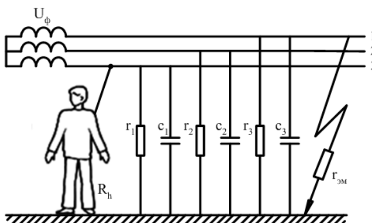
Рисунок 2.3 – Трехпроводная сеть с изолированной нейтралью; аварийный режим
