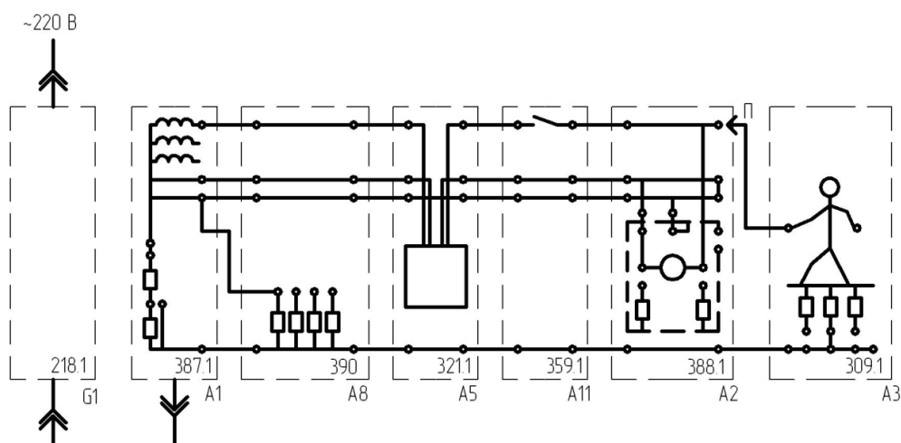
Рисунок 3.3 – Схема для выявления действия защиты при прямом прикосновении человека к частям, находящимся под напряжением
