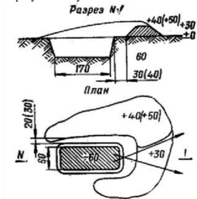
Одиночный окоп для стрельбы из автомата с колена
