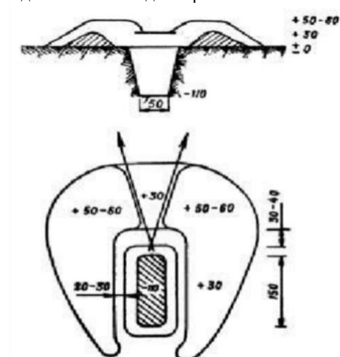
Одиночный окоп для стрельбы из автомата стоя
