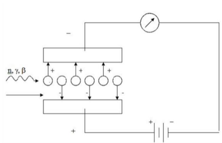
Рисунок 2.3 – Принципиальная схема работы ионизационной камеры
