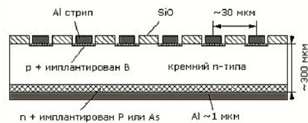
Рисунок 2.5 – Устройство кремниевого микрострипового детектора
