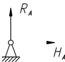
Рисунок 2 – Шарнирно-неподвижная опора
