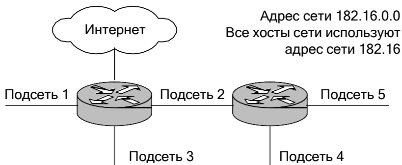
Рисунок 1.2 – Использование подсетей
