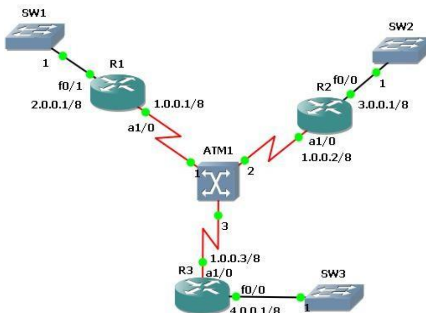
Рисунок 20 – Топология сети ATM
