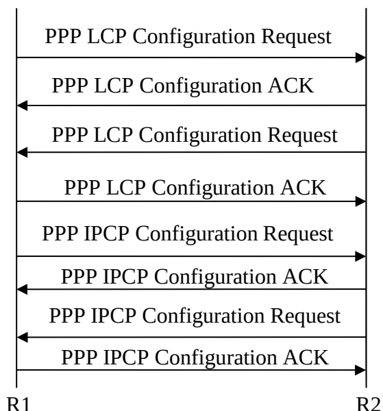
Рисунок 7 - Сценарий установления PPP соединения
