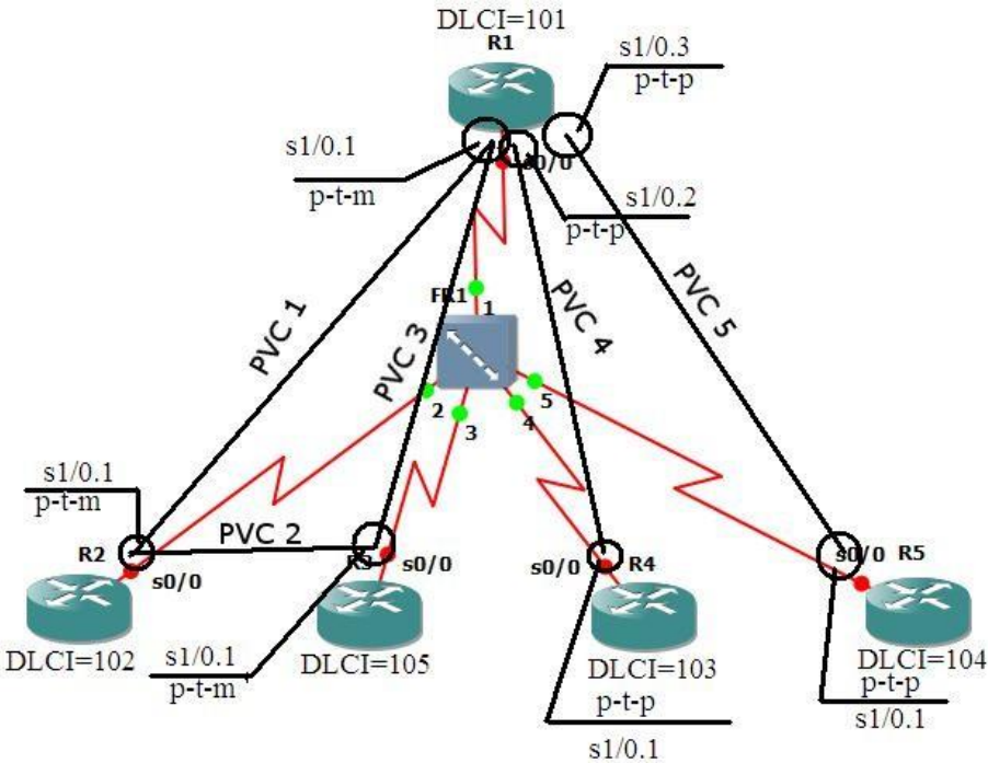
Рисунок 19 – Исследуемая топология
