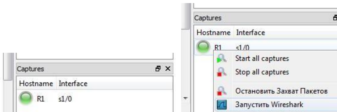
Рисунок 4 - Процедура захвата пакетов
