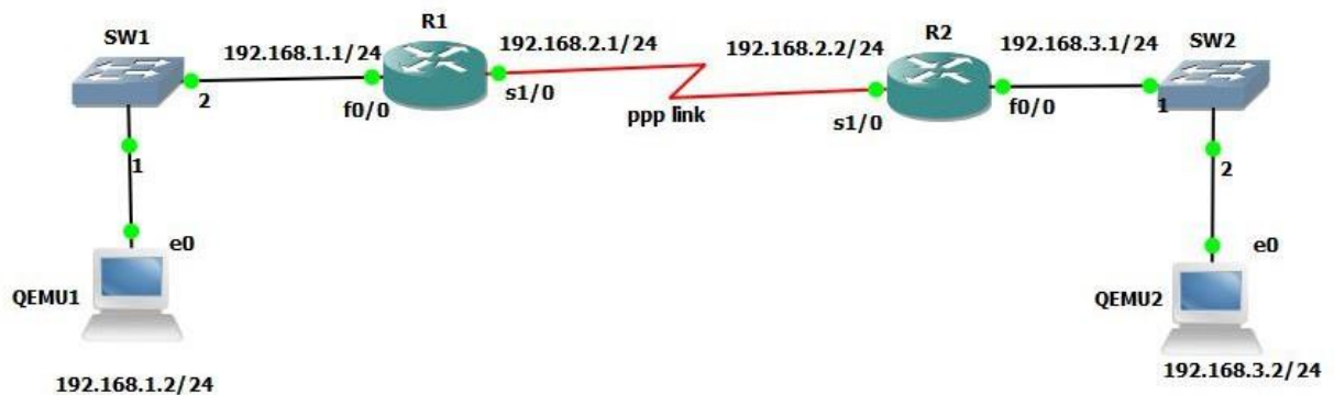
Рисунок 1 - Топология сети
