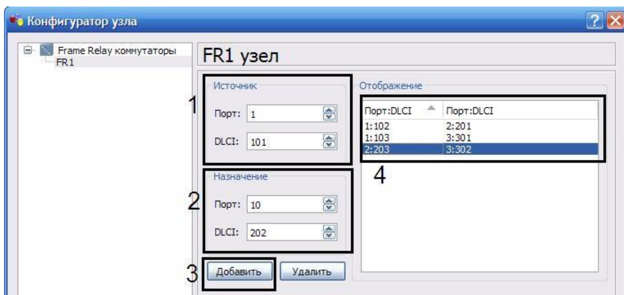
Рисунок 16 – создание таблицы коммутации
