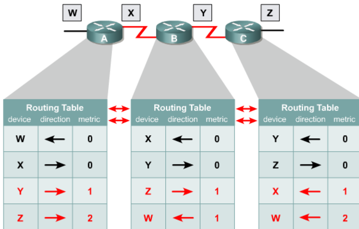
Рис.1. Дистанционно-векторная маршрутизация.
