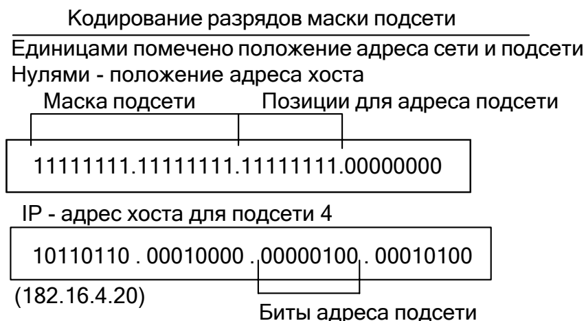
Рисунок 1.7 – Просмотр IP-адреса с помощью маски подсети
