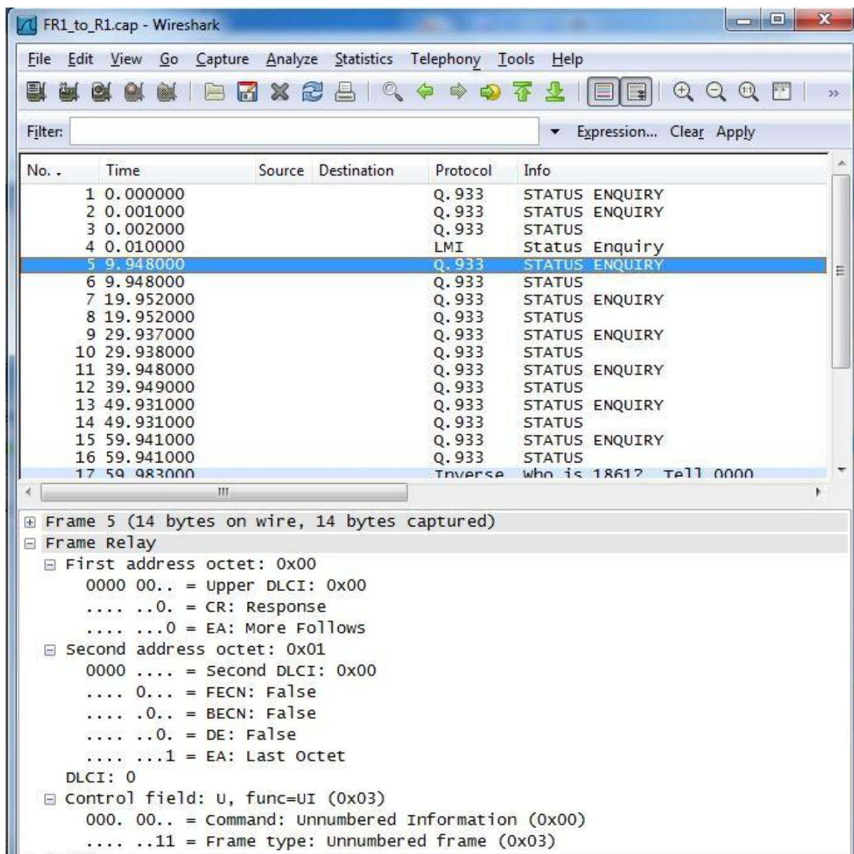
Рисунок 18 – Захват сообщений интерфейса LMI
