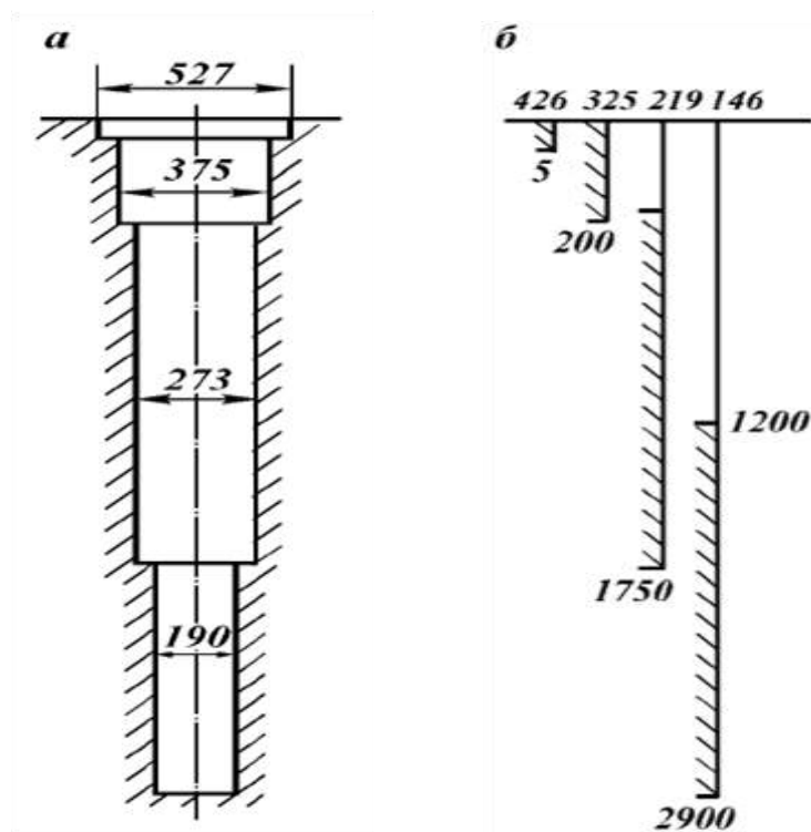
Рис. 6 – Конструкция скважины
