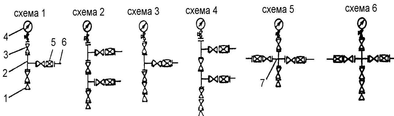
Рисунок 10 – Типовые схемы фонтанных елок:
