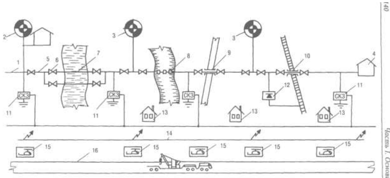
Рис. 22– Состав сооружений магистрального нефтепровода: 1 – подводящий трубопровод; 2 – головная нефтеперекачивающая станция; 3 – промежуточная нефтеперекачивающая станция; 4 – конечный пункт; 5 – линейная часть; 6 – линейная задвижка; 7 – дюкер; 8 – надземный переход; 9 – переход под автодорогой; 10 – переход под железной дорогой; 11 – станция катодной защиты; 12 – дренажная установка; 13 – дом обходчика; 14 – линия связи; 15 – вертолетная площадка; 16 – вдоль трассовая дорога.
