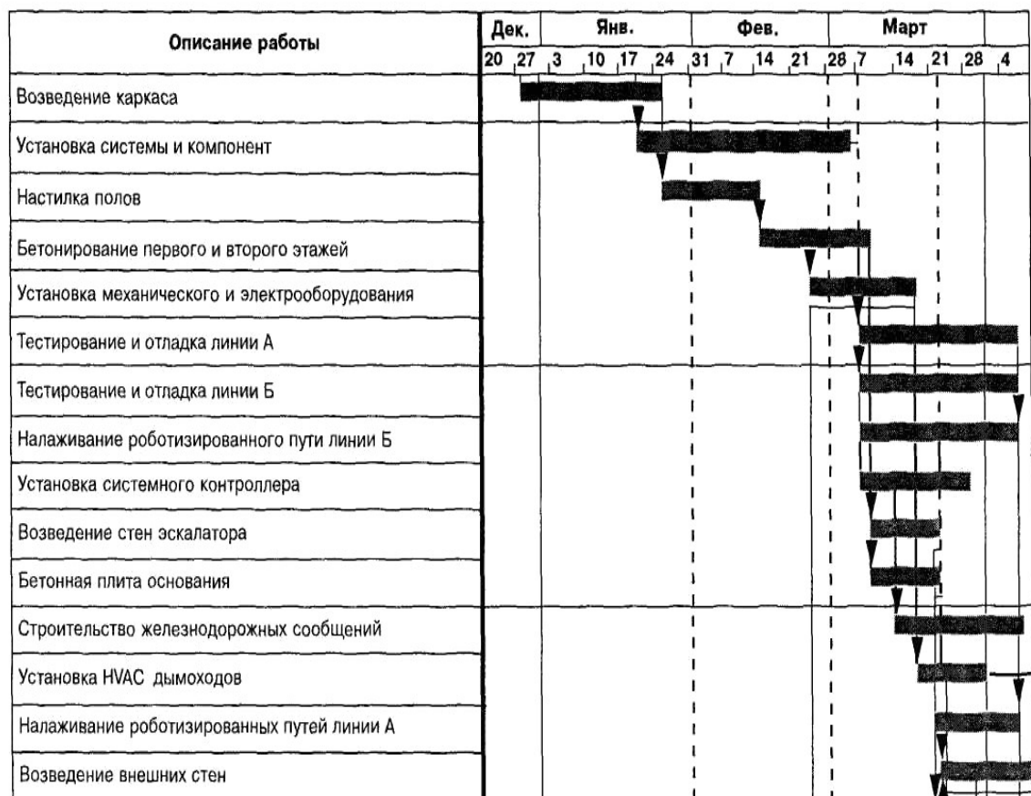
Рисунок 4.2 – Диаграмма Ганта
