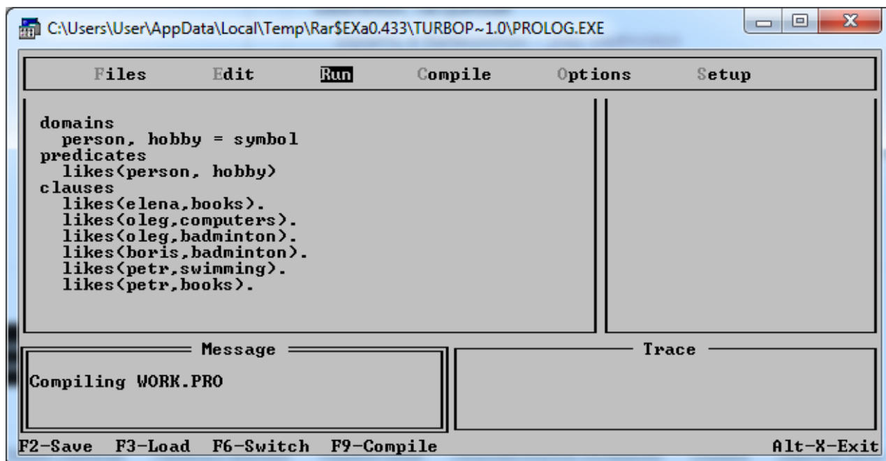
Рисунок 2.4 – Пример 2.3
