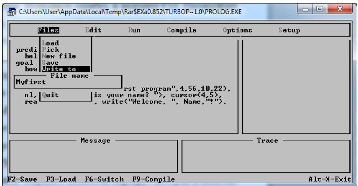
Рисунок 1.9 – Пример 1.1 (сохранение)
