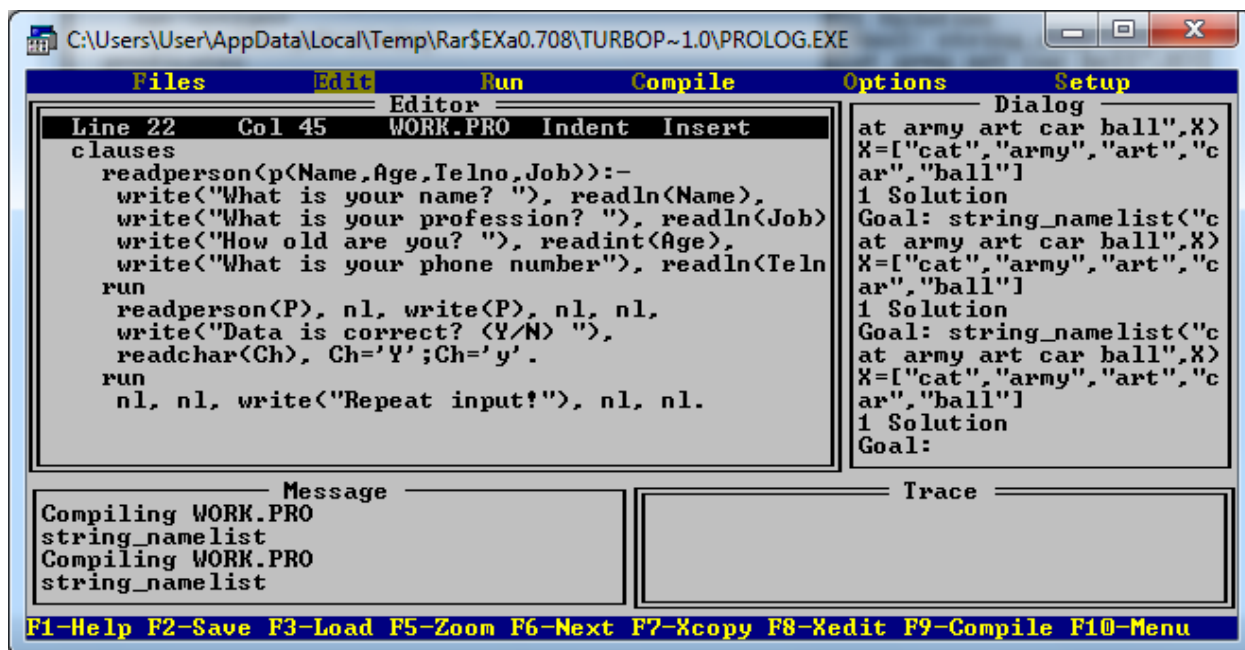
Рисунок 8.2 – Пример 8.1 (продолжение)
