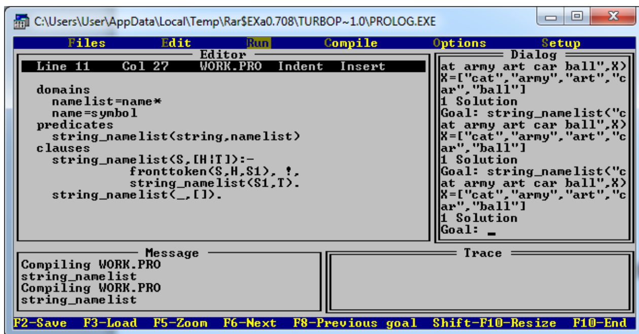
Рисунок 7.2 – Пример программы
