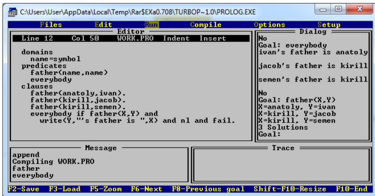
Рисунок 5.1 – Пример 5.1
