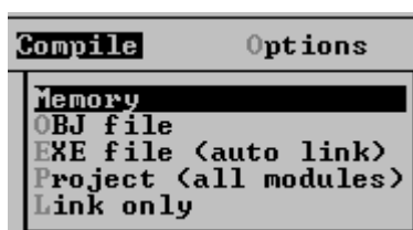
Рисунок 1.3 – Меню Compile
