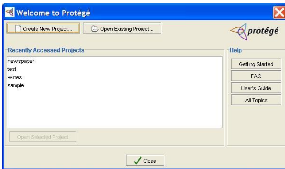
Рисунок 13.1 – Окно приветствия
