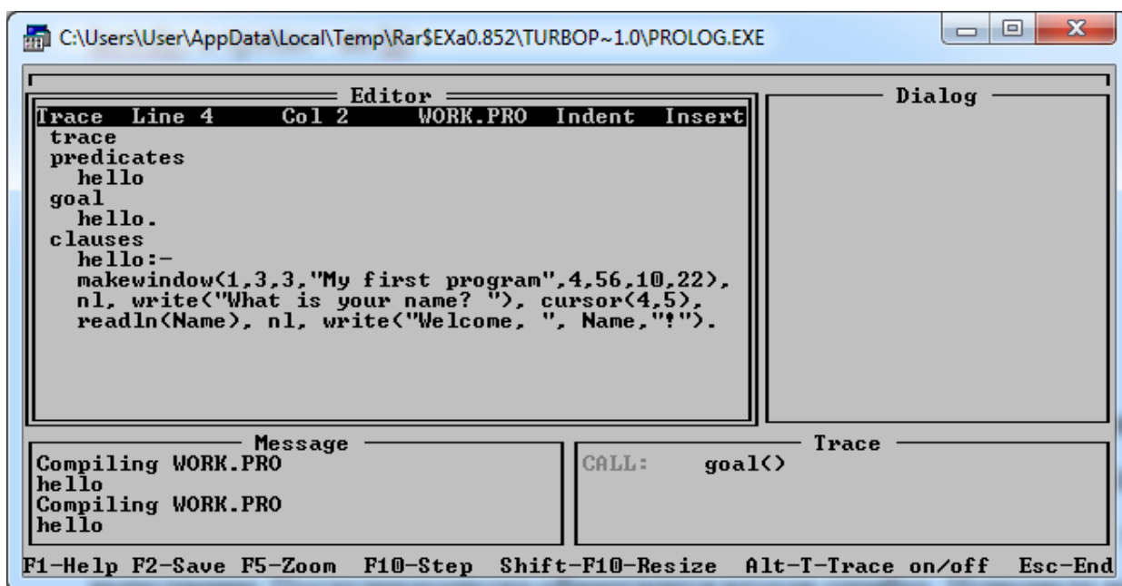
Рисунок 1.10 – Пример 1.1 (трассировка)
