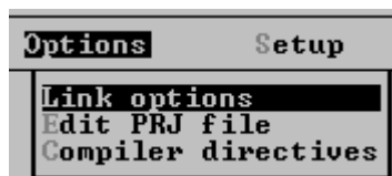
Рисунок 1.4 – Меню Options
