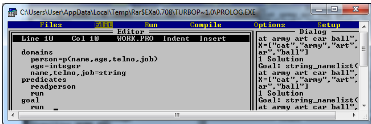
Рисунок 8.1 – Пример 8.1
