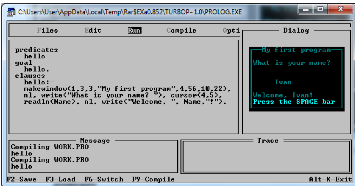
Рисунок 1.7 – Пример 1.1 (выполнение)
