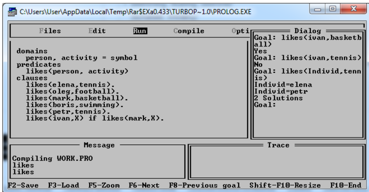
Рисунок 2.1 – Пример 2.1
